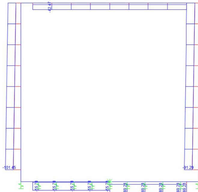
Figura 9.8 - Sforzo Normale – Involuppo SLE-Frequente
