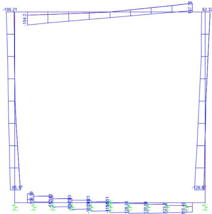
Figura 9.5 - Taglio – Inviluppo SLU
