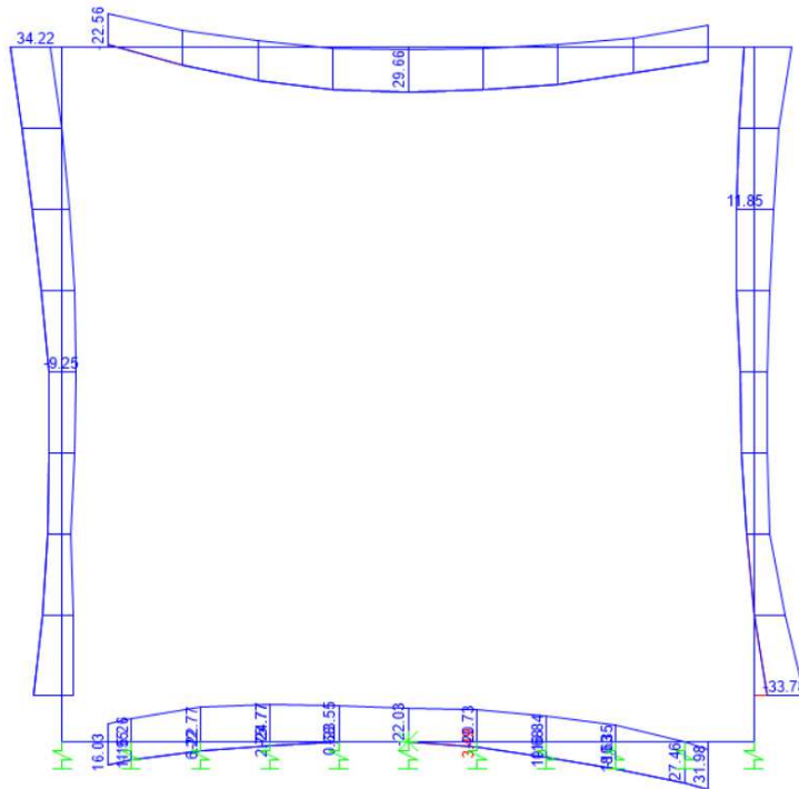
Figura 9.9 - Momento flettente – Inviluppo SLE-Frequente
