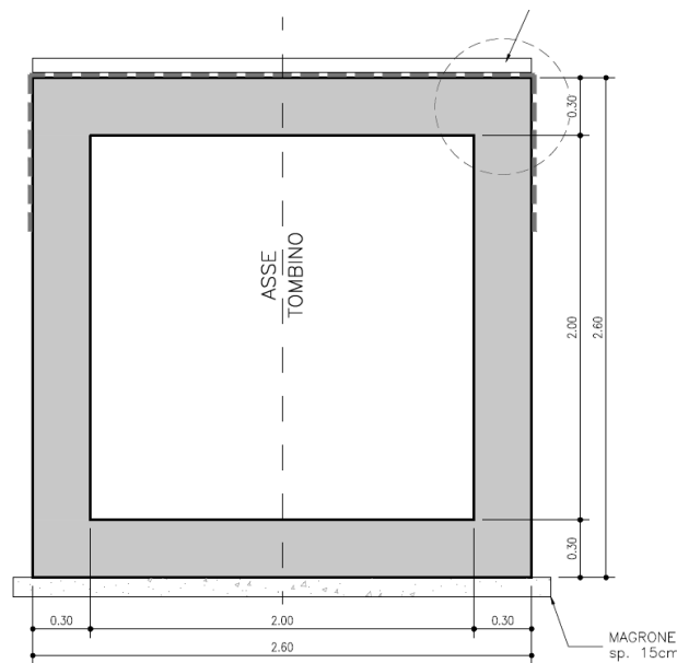
Figura 2.1– Sezione trasversale tombino idraulico
