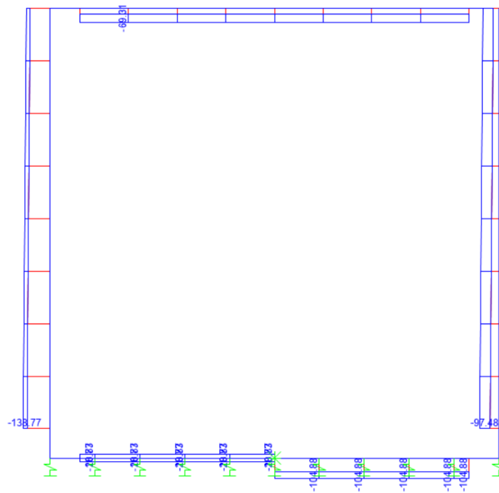
Figura 9.6 - Sforzo Normale – Inviluppo SLE-Rara
