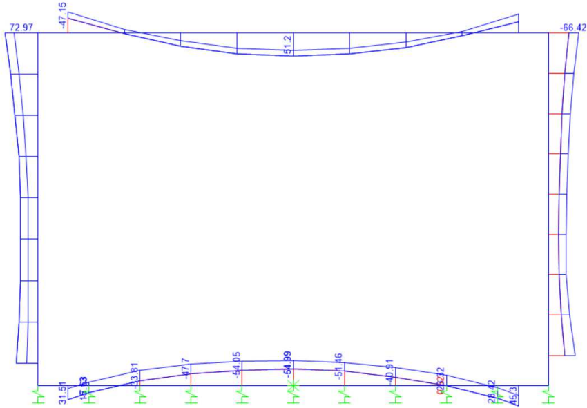
Figura 9.9 - Momento flettente – Involuppo SLE-Frequente
