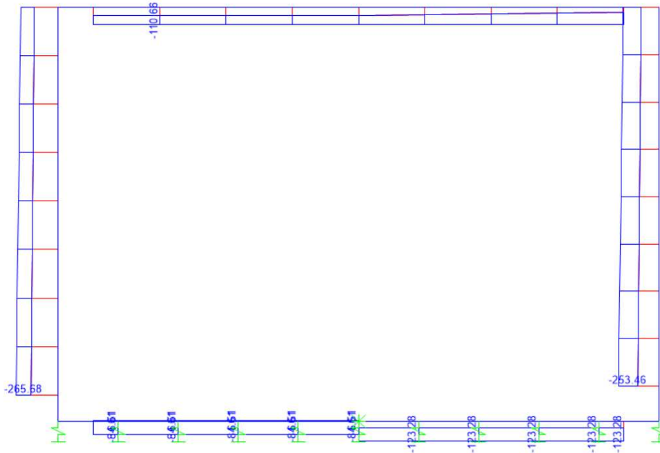
Figura 9.3 - Sforzo Normale – Inviluppo SLU
