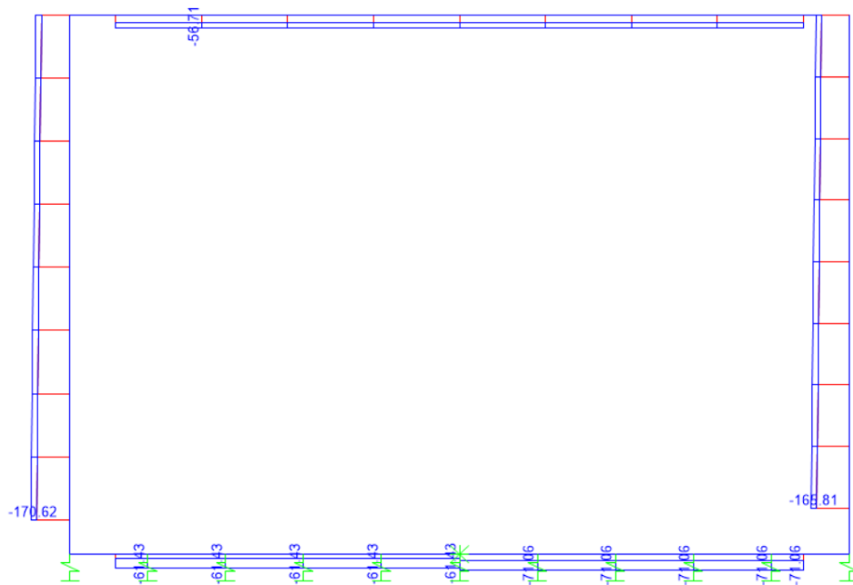
Figura 9.8 - Sforzo Normale – Involuppo SLE-Frequente
