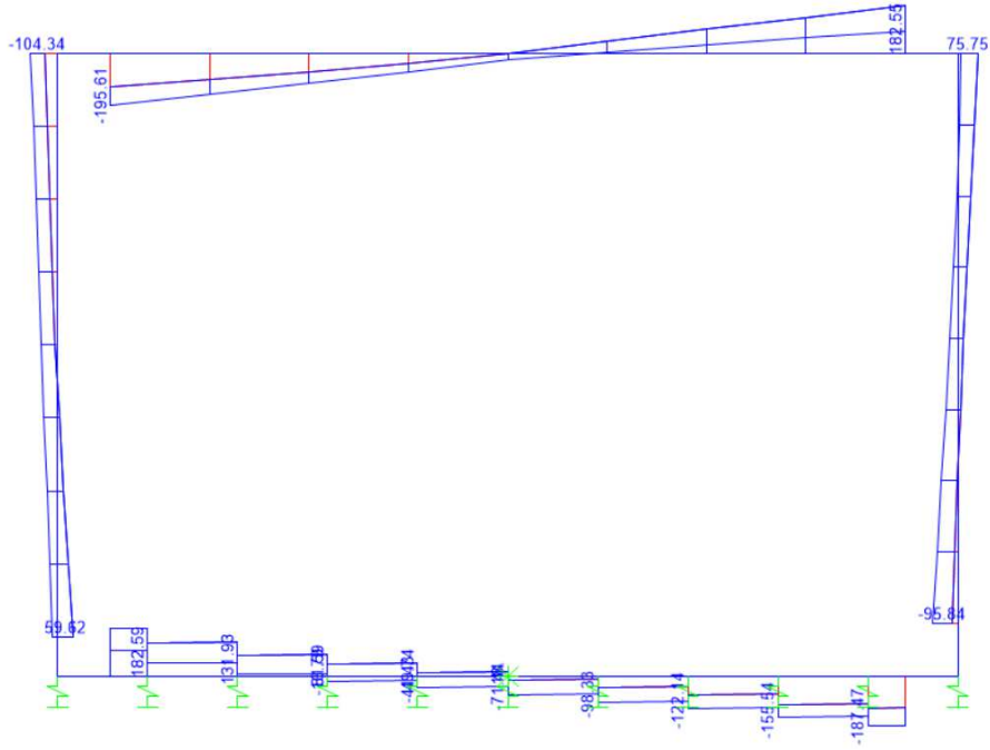
Figura 9.5 - Taglio – Inviluppo SLU
