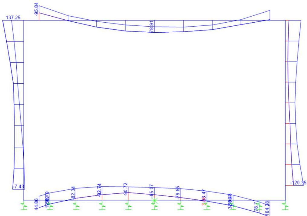
Figura 9.4 - Momento flettente – Inviluppo SLU
