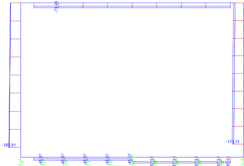
Figura 9.6 - Sforzo Normale – Inviluppo SLE-Rara
