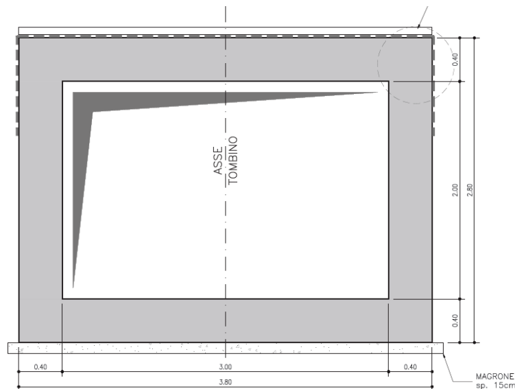
Figura 2.1- Sezione trasversale tombino idraulico
