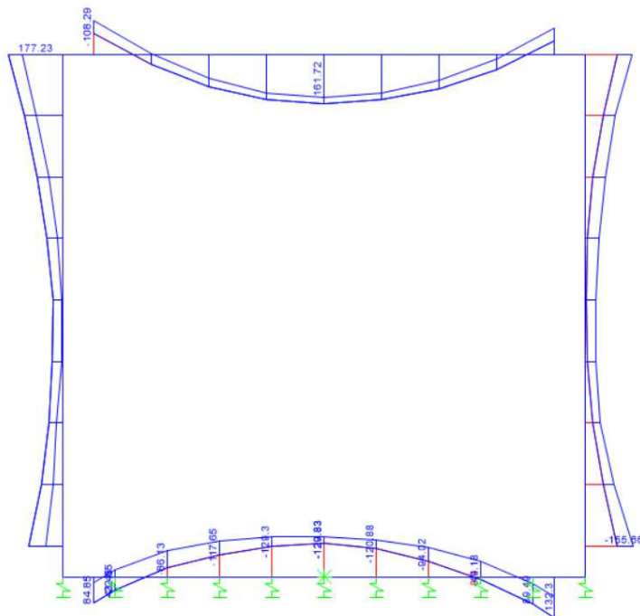
Figura 9.9 - Momento flettente – Involuppo SLE-Frequente
