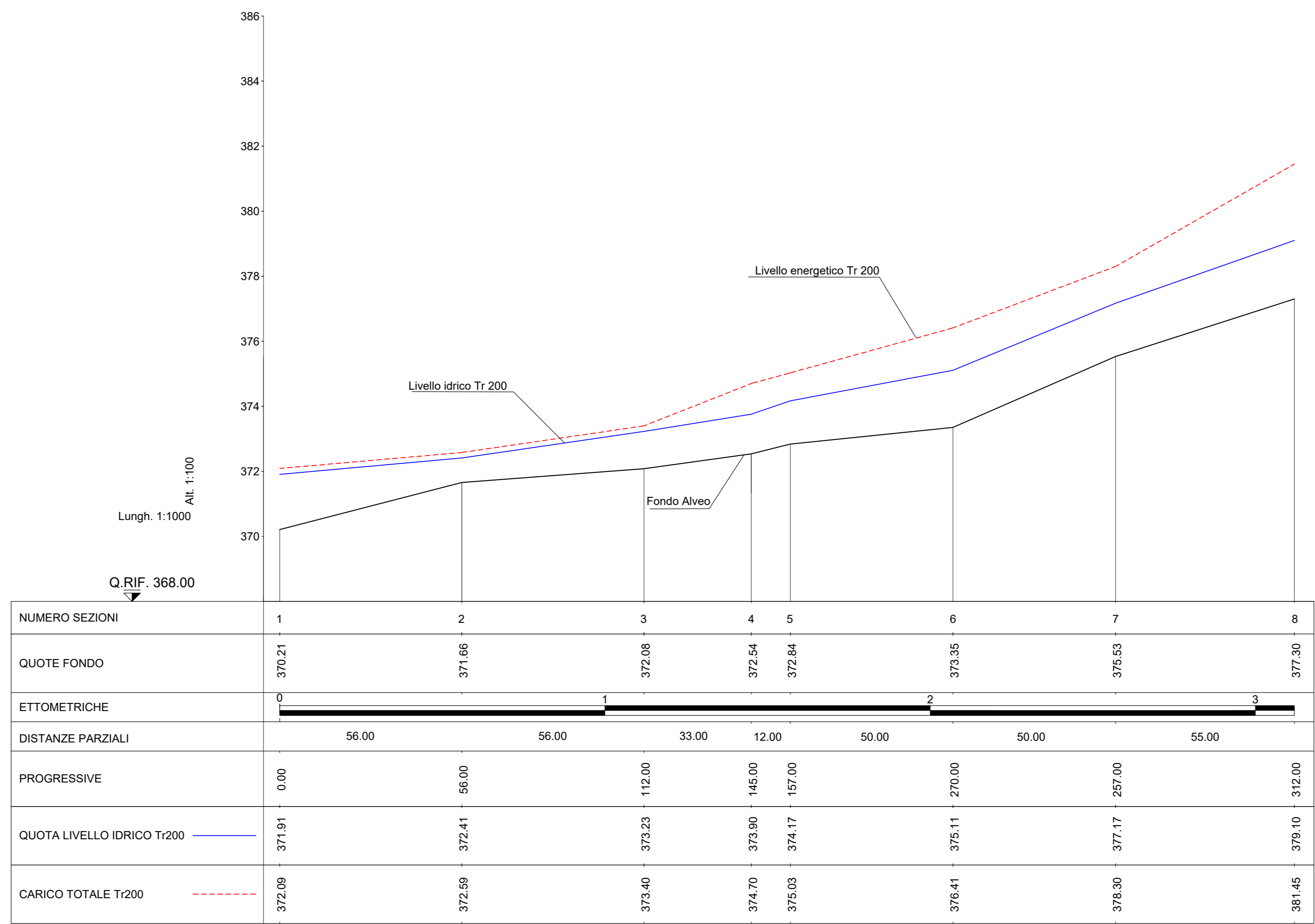
NW20 - Profilo di rigurgito ante operam
