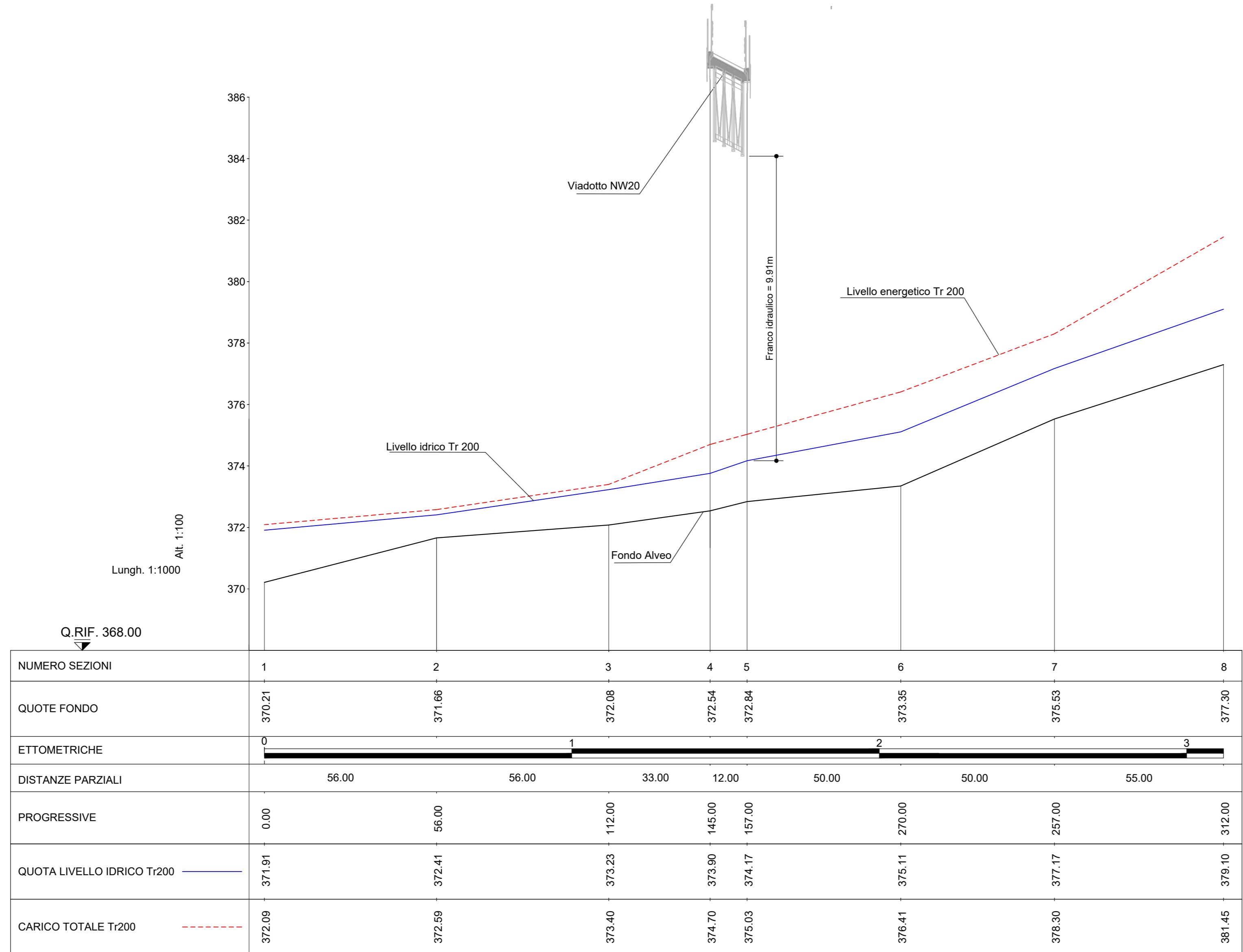
NW20 - Profilo di rigurgito post operam
