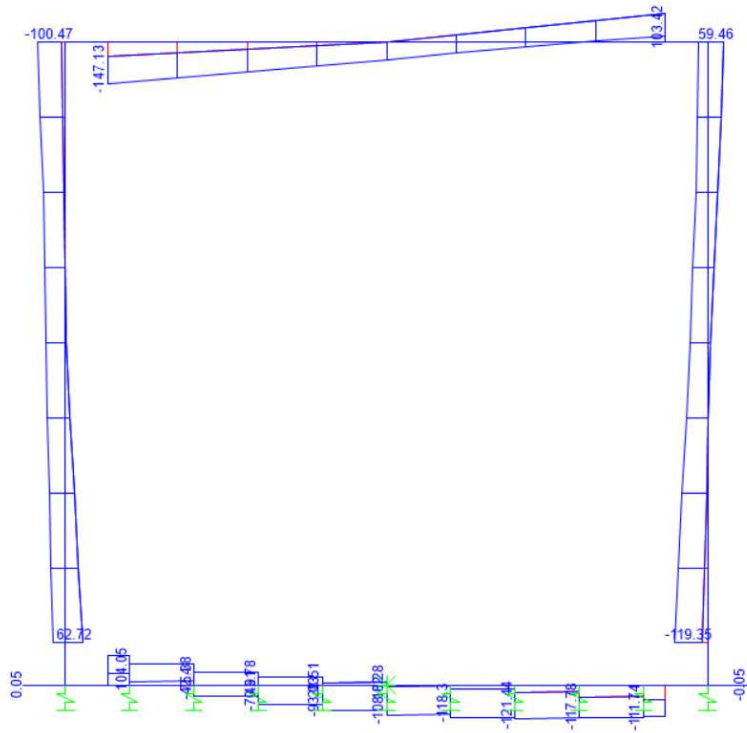
Figura 9.5 - Taglio – Inviluppo SLU
