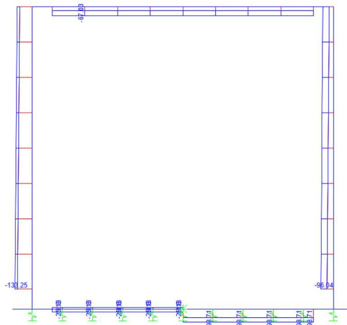
Figura 9.6 - Sforzo Normale – Inviluppo SLE-Rara
