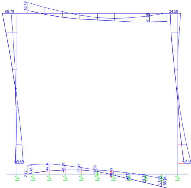
Figura 9.7 - Momento flettente – Involuppo SLE-Rara
