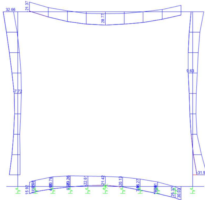
Figura 9.9 - Momento flettente – Inviluppo SLE-Frequente
