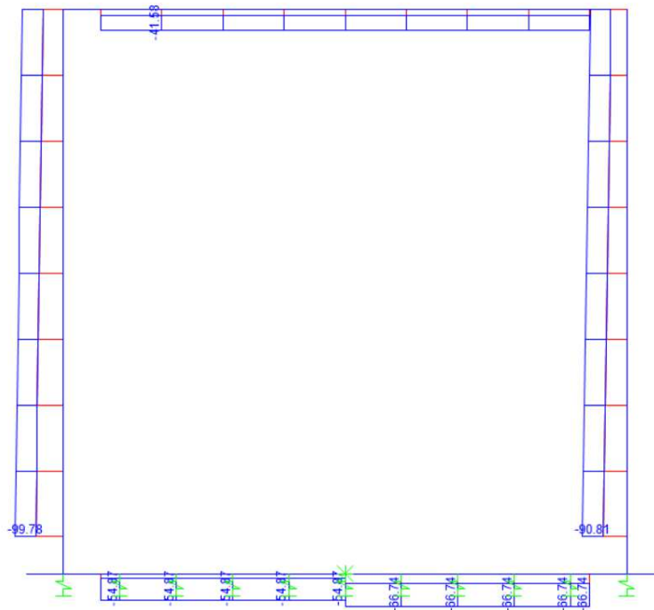
Figura 9.8 - Sforzo Normale – Involuppo SLE-Frequente
