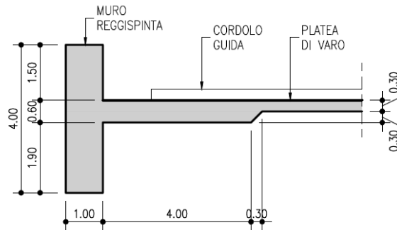
Fig. 3.4 Struttura reggispinta
