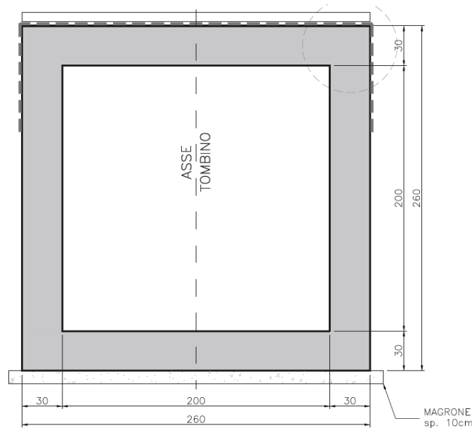
Fig. 3.2 Tombino scatolare - sezione trasversale
