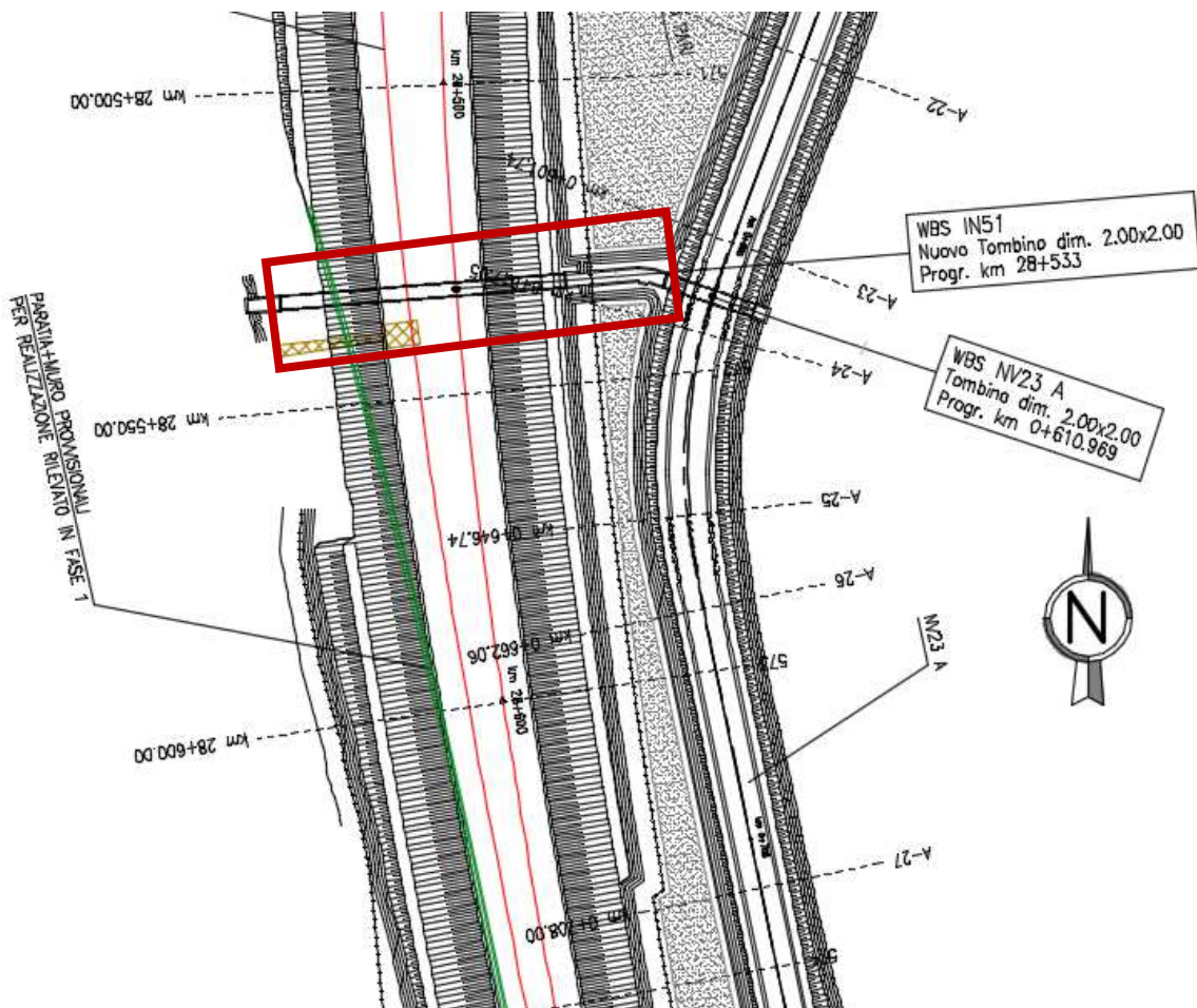
Fig. 3.1: Inquadramento dell'opera
