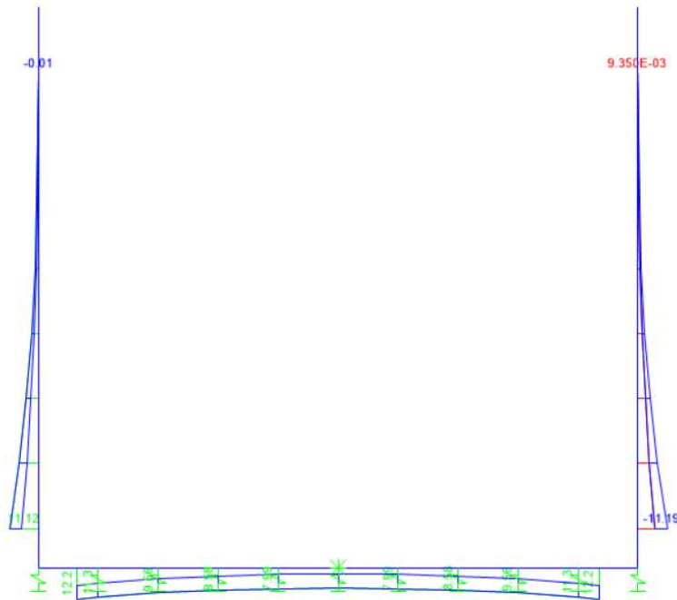
Figura 9.7 - Momento flettente - Inviluppo SLE-Rara
