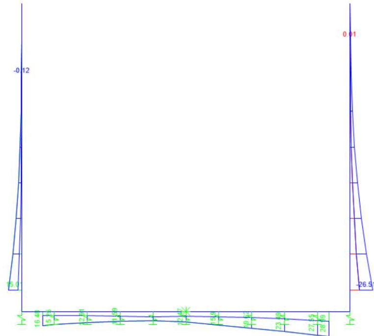
Figura 9.5 - Momento flettente - Inviluppo SLU
