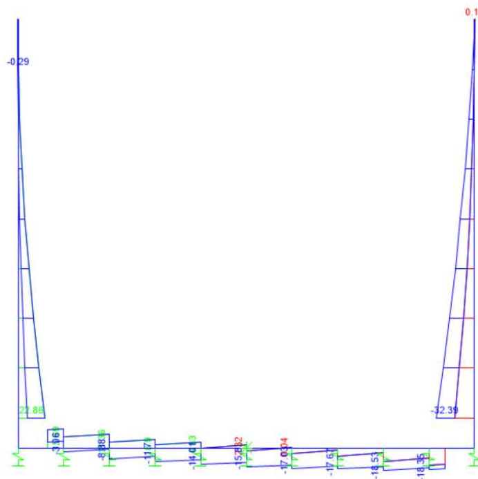
Figura 9.4 - Taglio - Involuppo SLU
