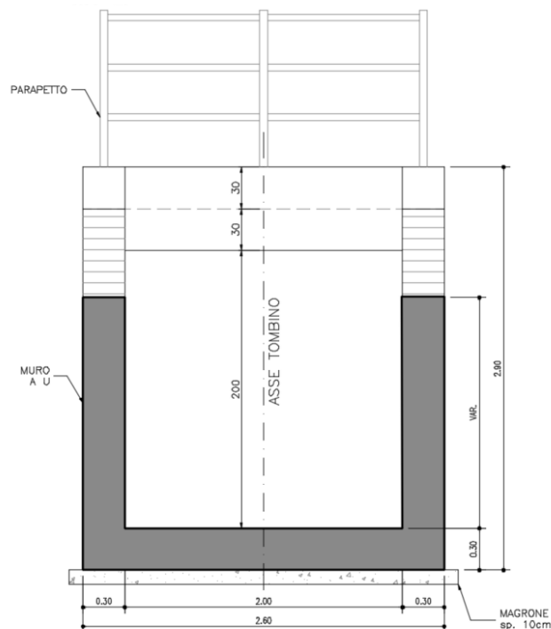
Figura 2.1– Sezione trasversale muro di imbocco
