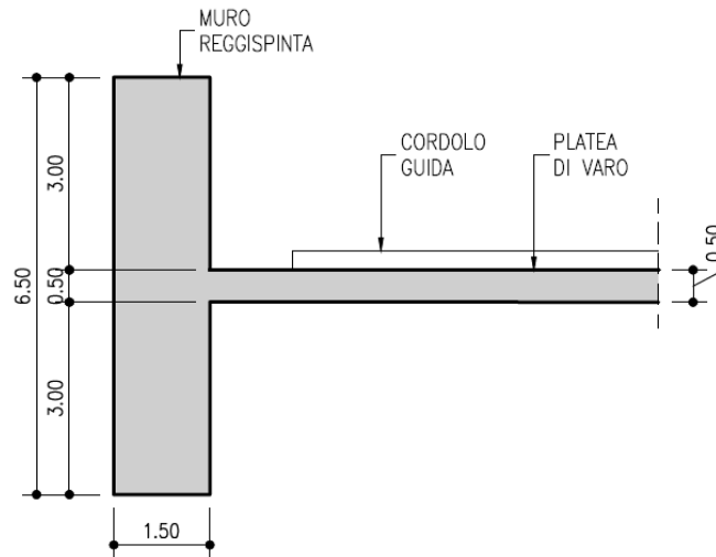
Fig. 3.3 Struttura reggispinta
