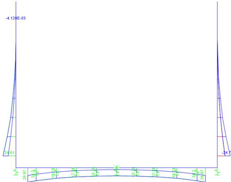
Figura 9.7 - Momento flettente - Involuppo SLE-Rara
