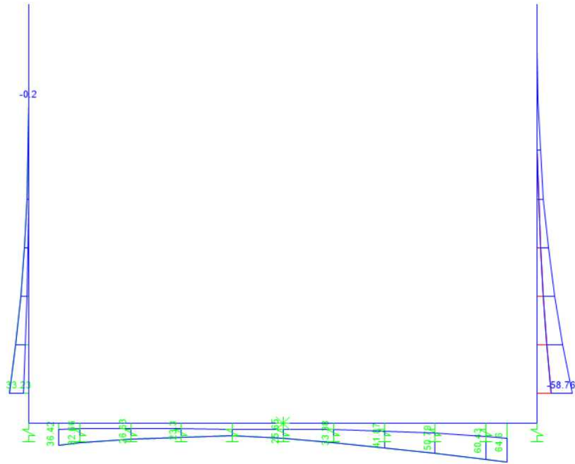
Figura 9.5 - Momento flettente – Involuppo SLU
