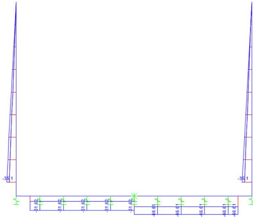
Figura 9.3 - Sforzo Normale – Involuppo SLU
