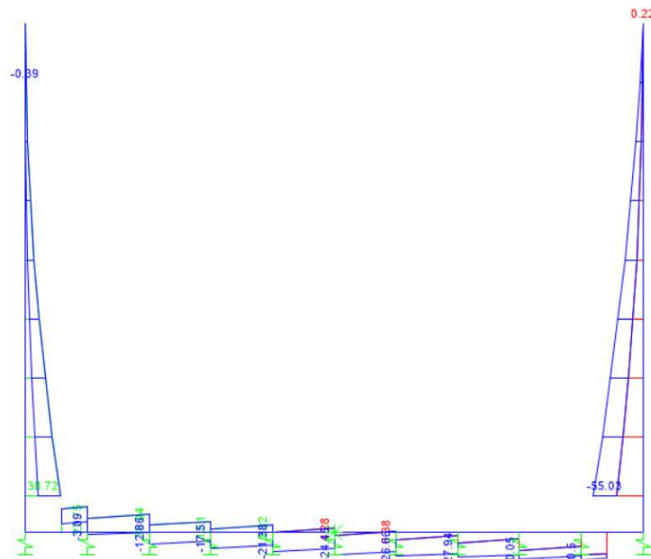
Figura 9.4 - Taglio – Involuppo SLU
