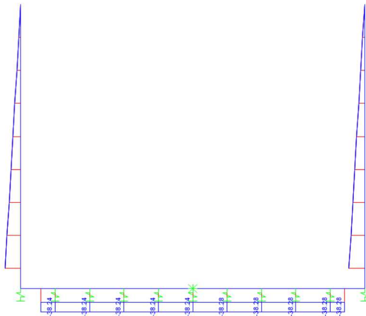
Figura 9.6 - Sforzo Normale – Involuppo SLE-Rara
