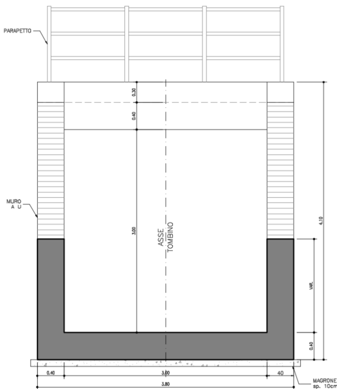
Figura 2.1– Sezione trasversale muro di imbocco
