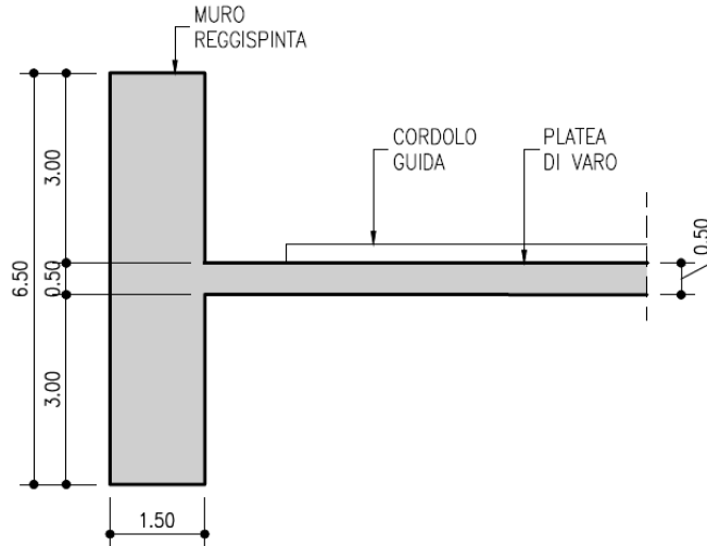
Fig. 3.3 Struttura reggispinta
