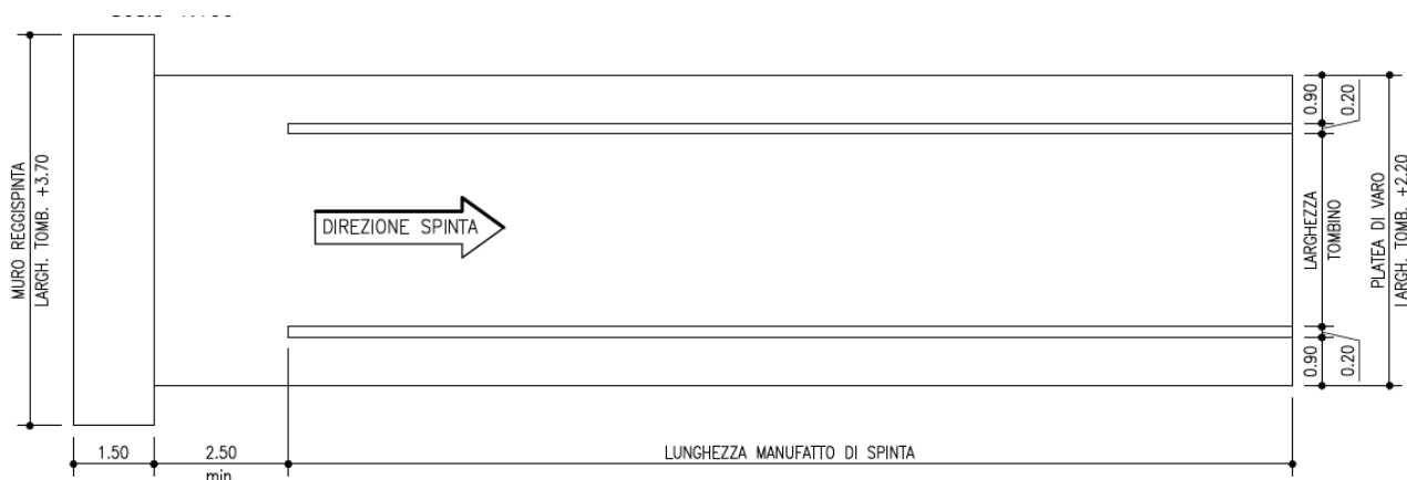
Fig. 3.2 Pianta platea di varo
