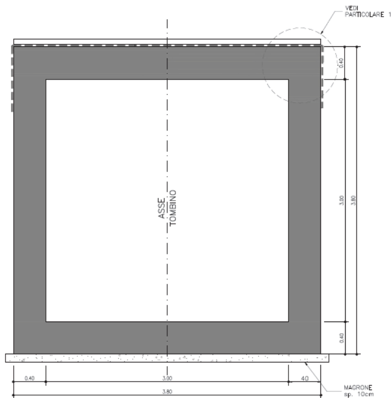
Fig. 1: Sezione trasversale del tombino
