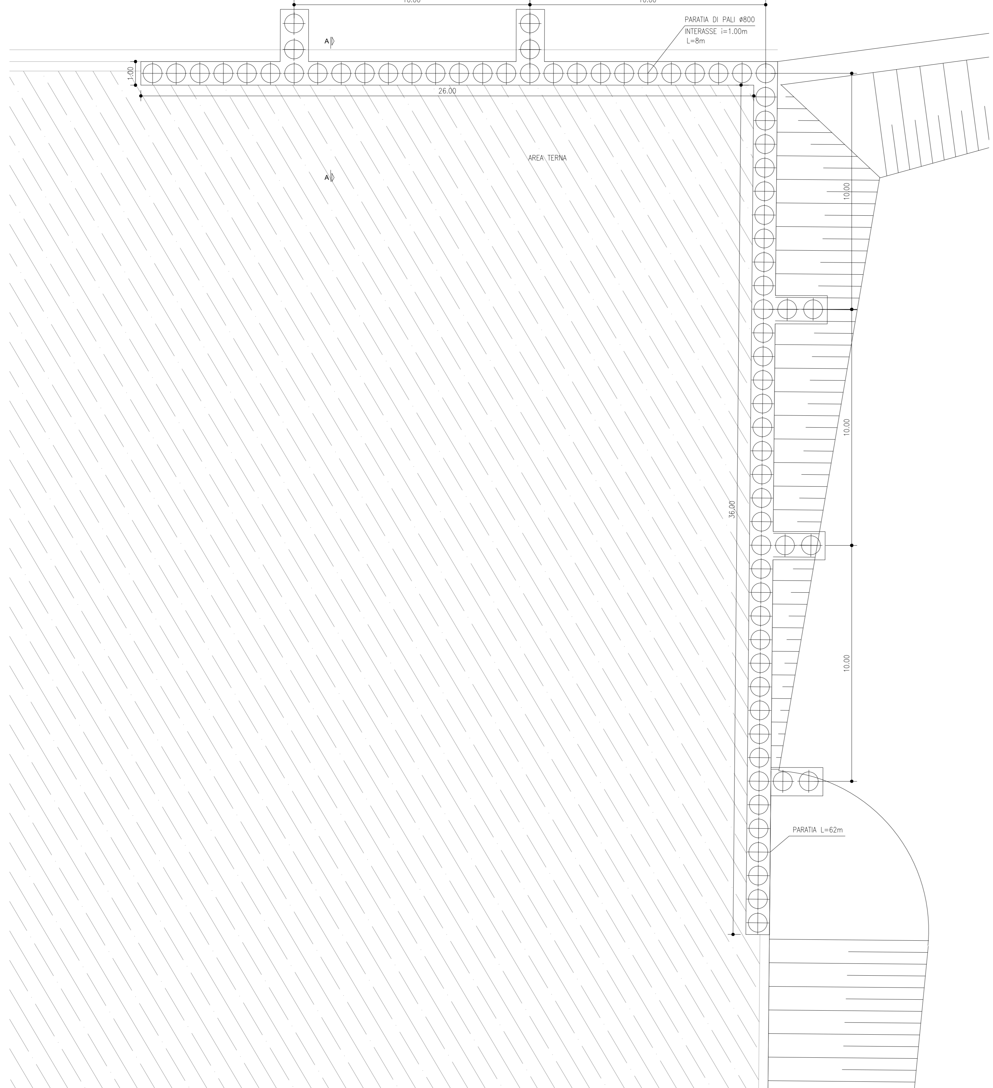
PARATIA SCALA 1:100 PIANTA
