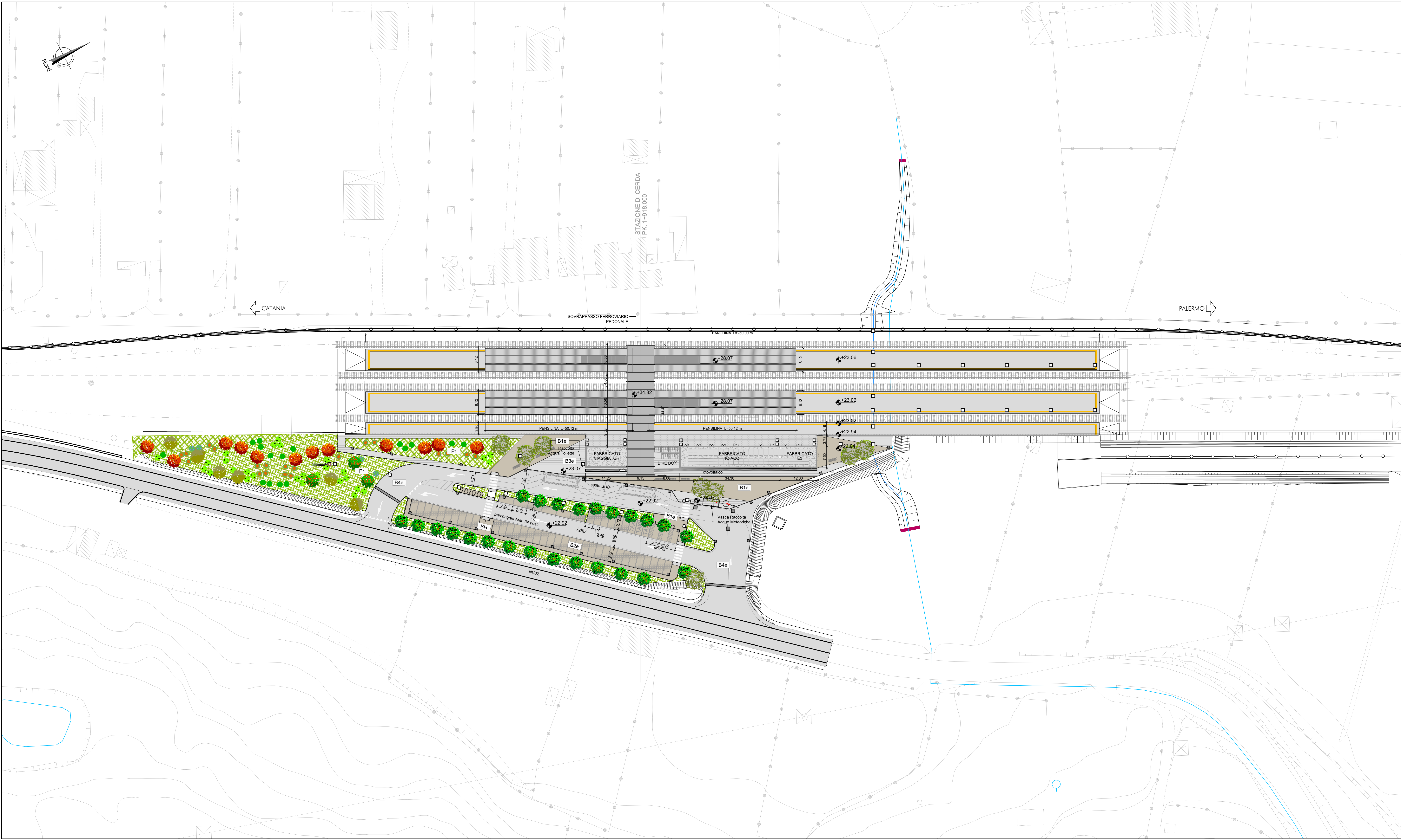
Planimetria generale Scala 1:500
