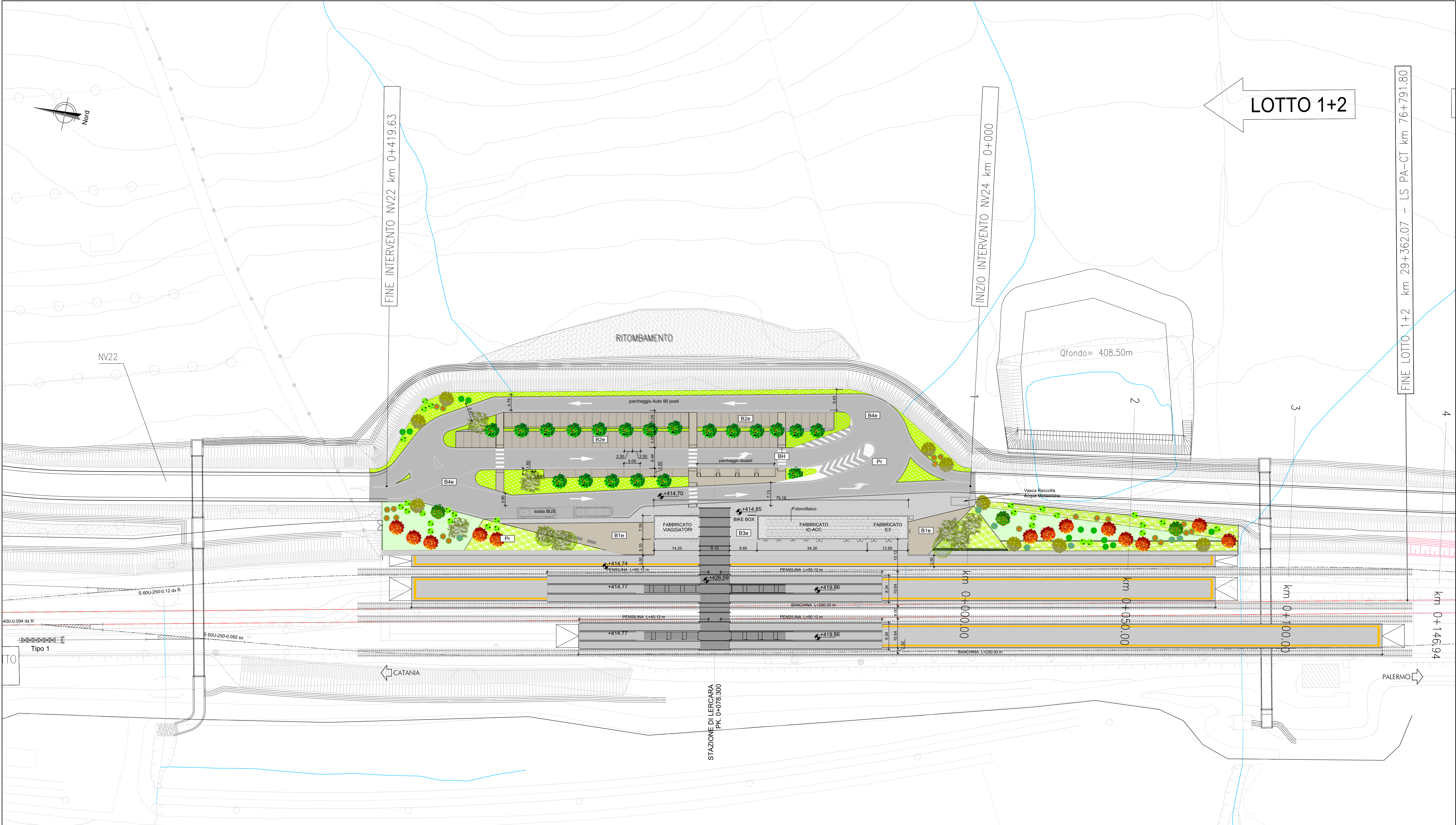
Planimetria generale Scala 1:500
