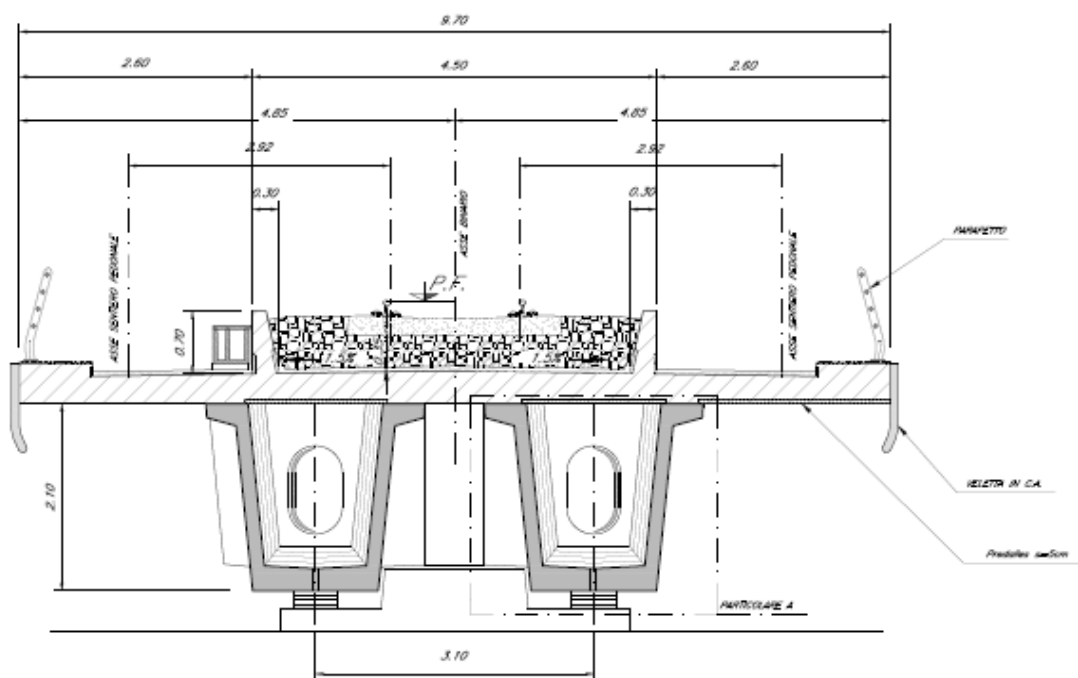
Figura 7 – VI01 Sezione in CAP
