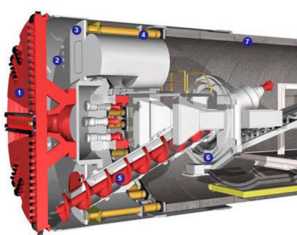
Figura 5 Schema di una macchina TBM, tipo EPB (1. Testa Fresante; 2. Camera di scavo; 3. Parete di contenimento dotata di sistema d'accesso (camera iperbarica) alla camera di scavo; 4. Pistoni di avanzamento; 5. Coclea; 6. Erettore dei conchi; 7. Anelli di sosteg
