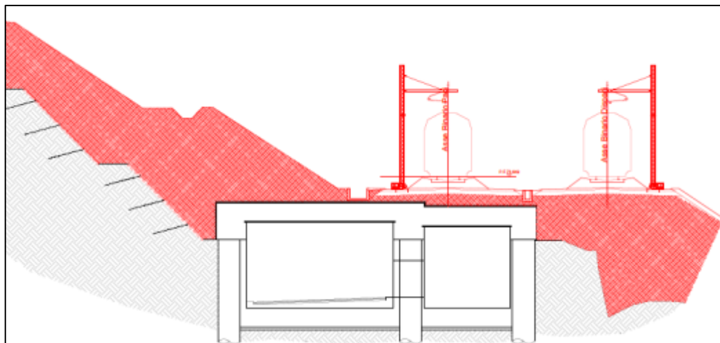
Figura 6 Galleria artificiale a servizio di un tratto della NV06
