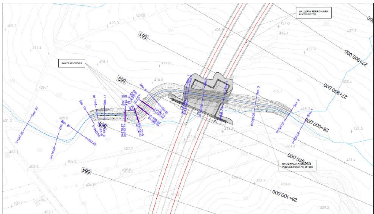
Figura 18 Configurazione post operam pk 28+000
