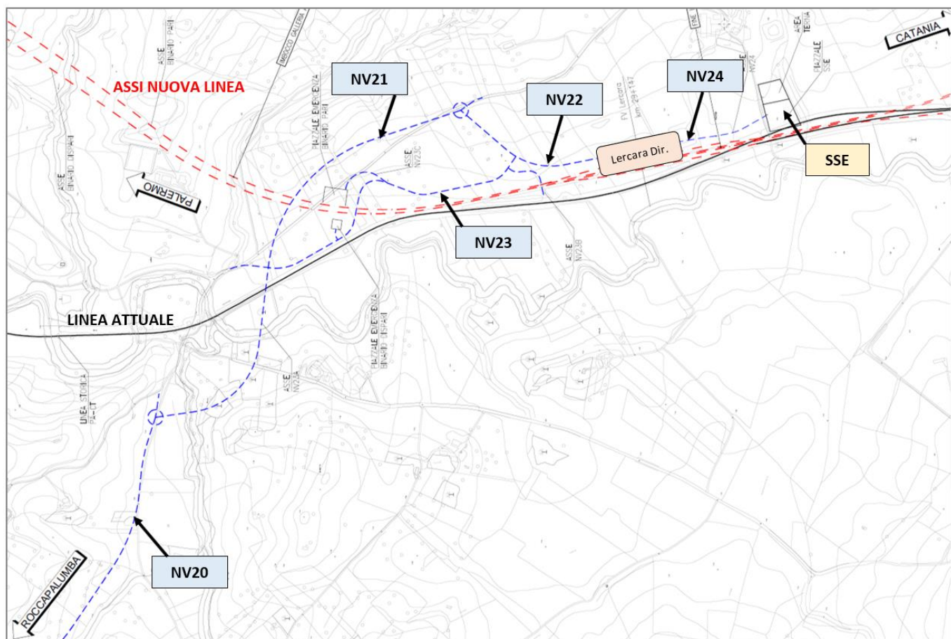
Figura 16 – Assetto viabilità lato Catania
