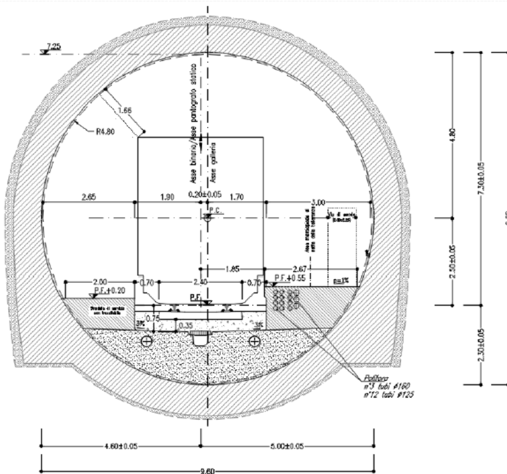
Figura 2 Sezione di intradosso scavo tradizionale per traslazione TBM
