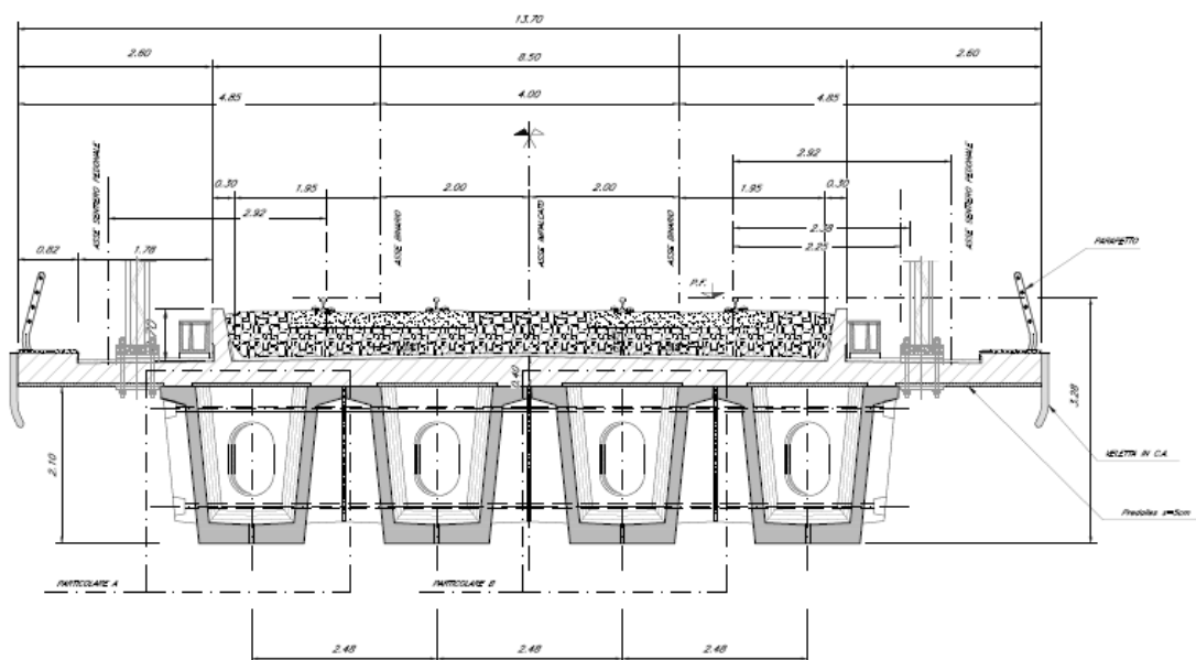
Figura 9 – VI02 Sezione campata in CAP da 25 m
