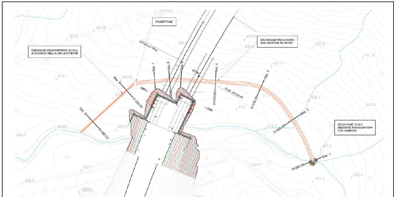
Figura 17 Deviazione provvisoria pk 28+000
