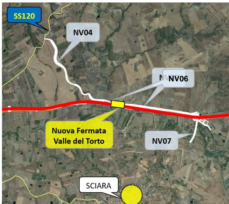
Figura 13 – Sistema di viabilità per l'accesso alla fermata di Valle del Torto (NV04 – NV06 – NV07)
