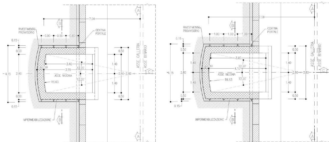
Figura 3 Pianta nicchia tecnologica standard (a sx) e nicchia specializzata TE (a dx)
