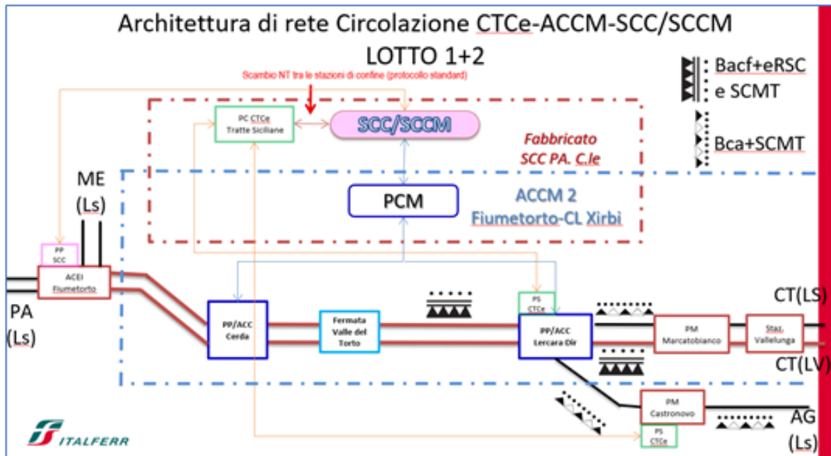
Figura 21 Architettura ACCM - SCCM - CTCe
