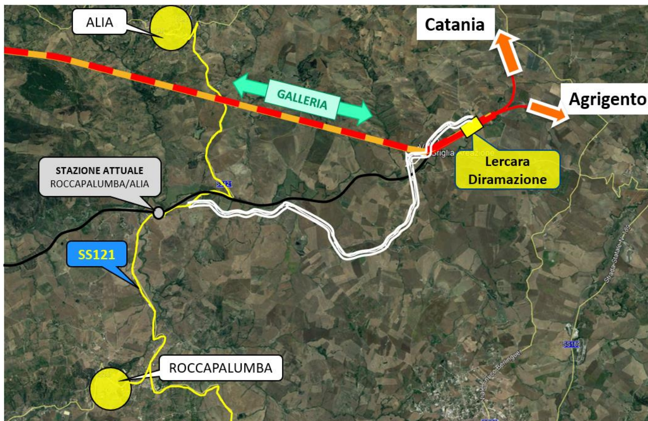
Figura 15 – Viabilità di accesso alla stazione di Lercara (NV20 – NV21 – NV22)
