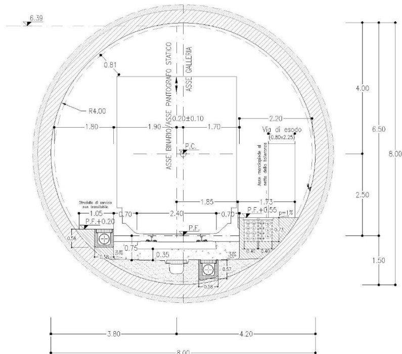
Figura 4 Sezione di intradosso in scavo meccanizzato
