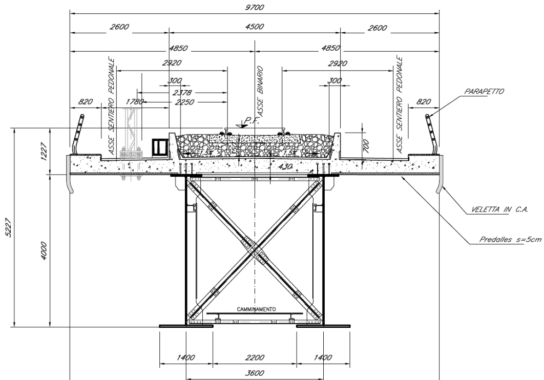
Figura 8 – VI01 Sezione mista acciaio - cls
