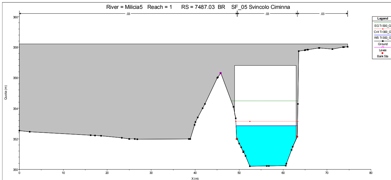
Figura 18- River station 7487.03D del modello idraulico del fiume Mulinazzo con Tr 300 anni
