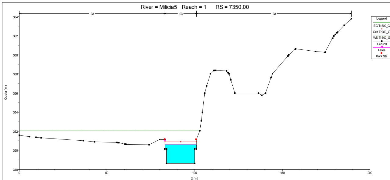
Figura 24- River station 7350.00 del modello idraulico del fiume Mulinazzo con Tr 300 anni
