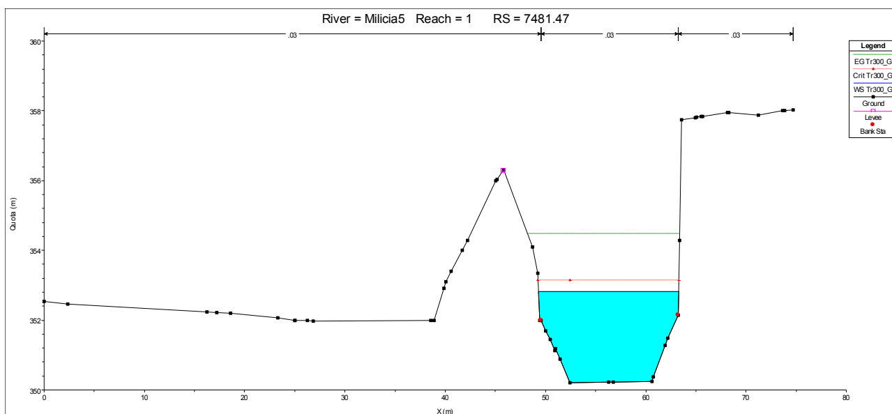
Figura 19- River station 7481.47 del modello idraulico del fiume Mulinazzo con Tr 300 anni
