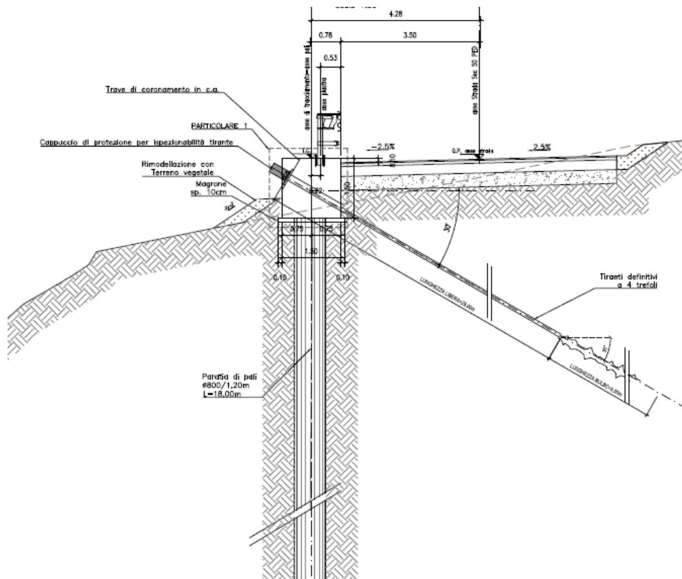
Figura 10 Sezione tipologica
