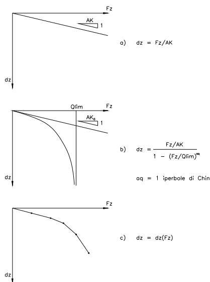
Pali soggetti a carichi assiali: reazioni carico-cedimento
