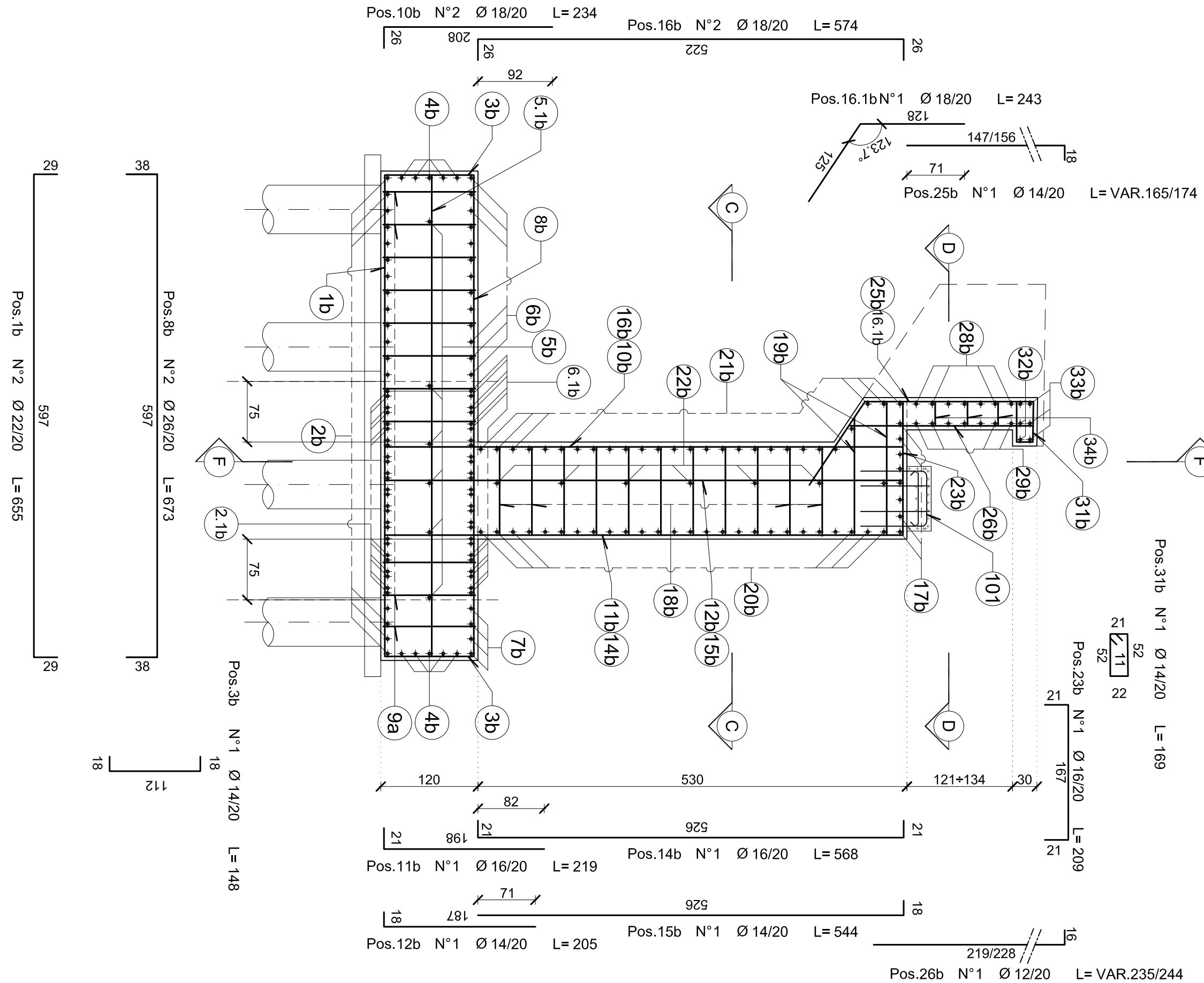
Spalla S2b Sezione B-B (Fondazione e fuso) Scala 1:50
