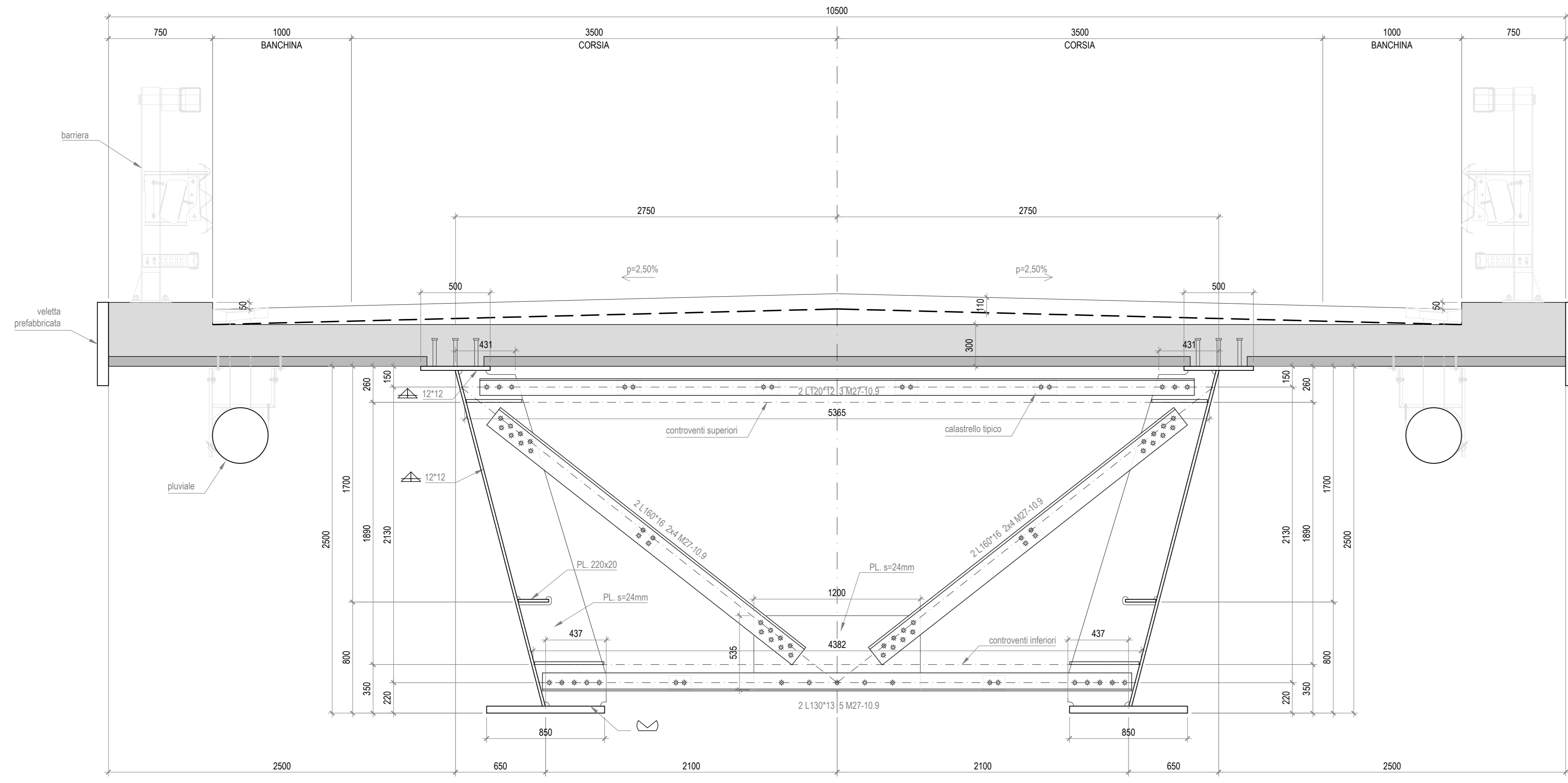
TIPOLOGIA DIAFRAMMI D8: SEZIONE TIPICA SCALA 1:20
