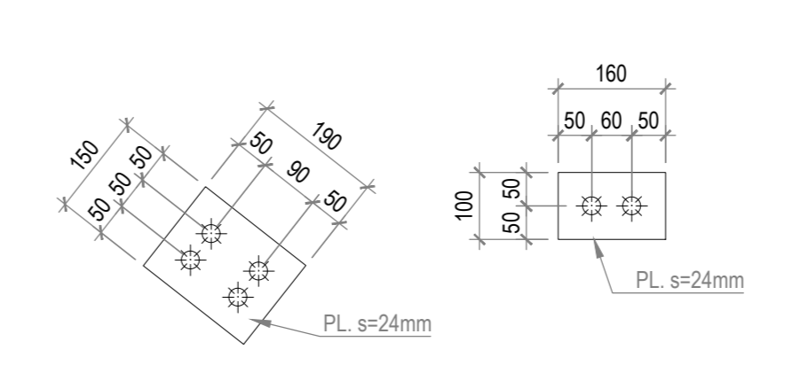
PARTICOLARE CALASTRELLO SCALA 1:10
