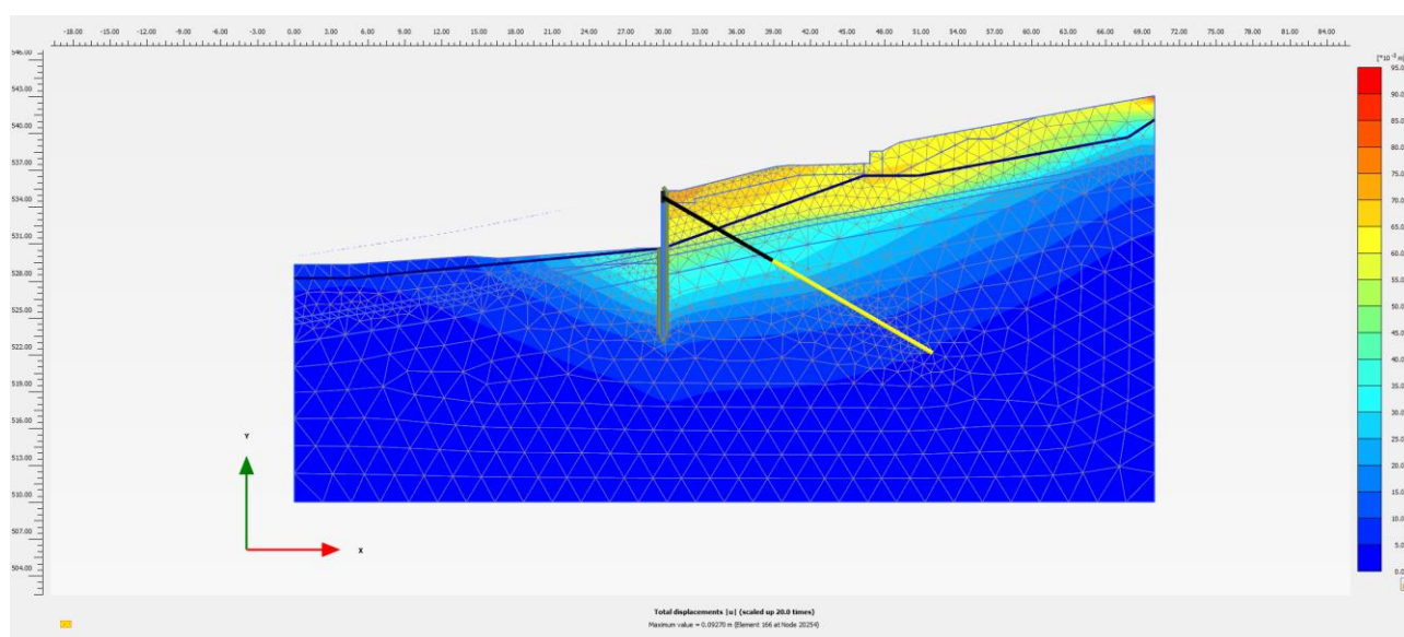
Figura 36: SLU(SLV)/GEO A2+M2+R1 - Combinazione fondamentale, campo di spostamenti
