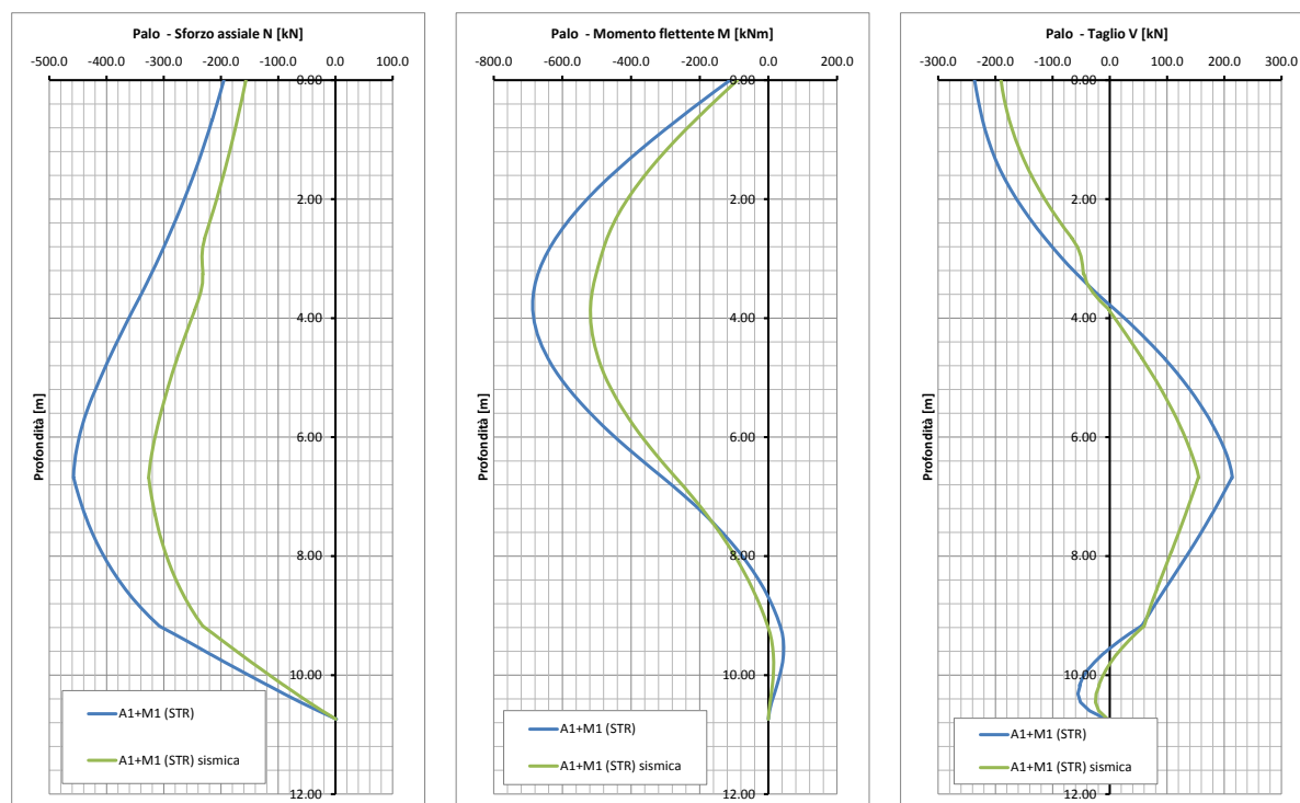
Figura 20: SLU(SLV)/STR A1+M1+R1-Pali. Diagrammi delle sollecitazioni
