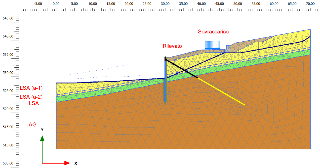
Figura 26: Sezione 30. Modello di calcolo Plaxis
