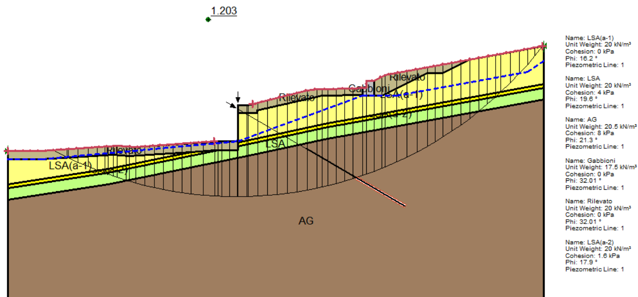
Figura 40: SLU(SLV)/GEO_stab A2+M2+R2-Combinazione sismica (kv<0)- - Superficie di scorrimento critica
