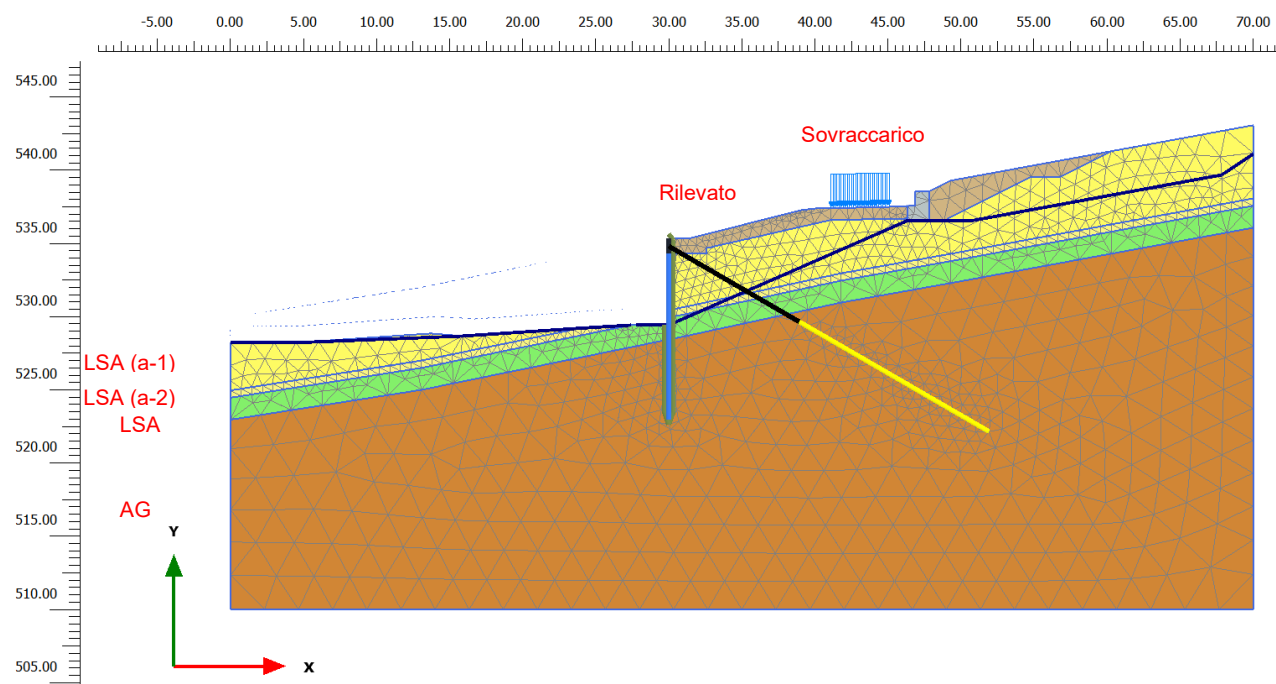
Figura 41: Sezione 35. Modello di calcolo Plaxis
