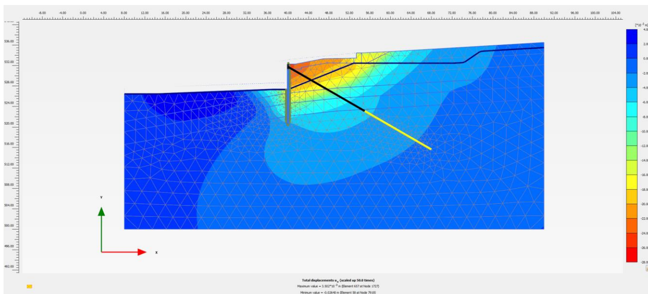
Figura 16: SLE-Combinazione caratteristica (rara).
