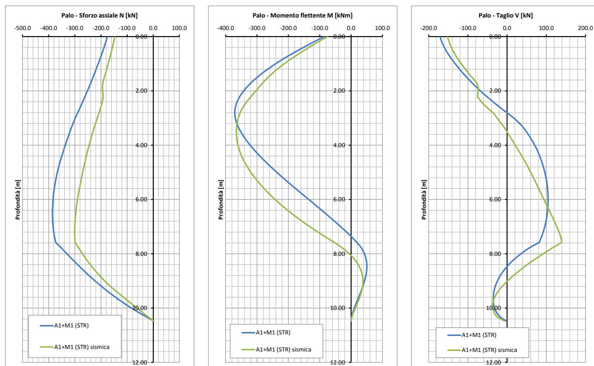
Figura 50: SLU(SLV)/STR A1+M1+R1-Pali. Diagrammi delle sollecitazioni
