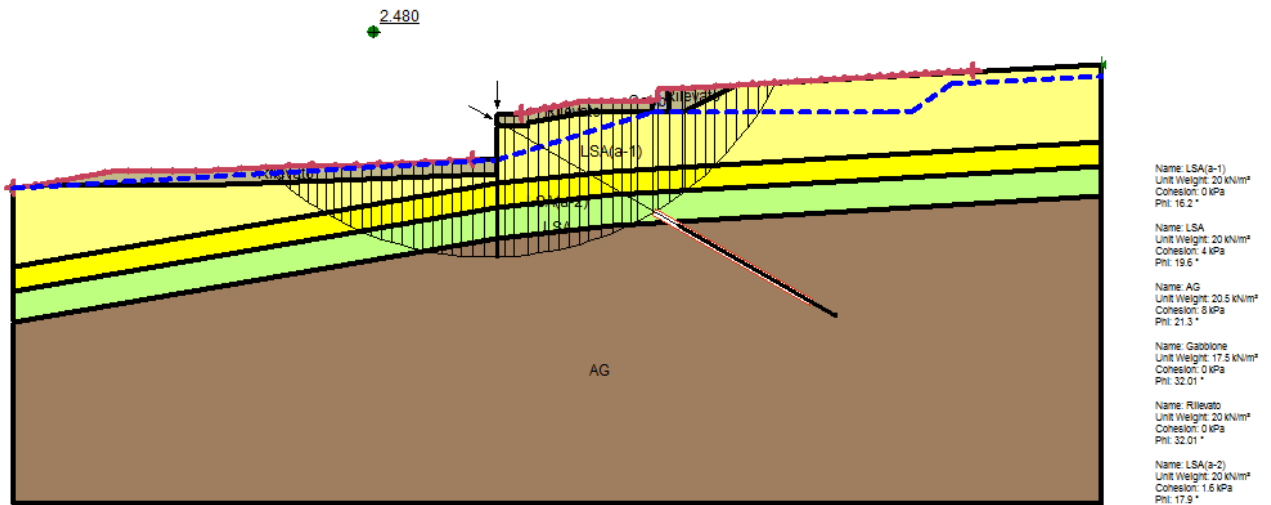
Figura 24: SLU(SLV)/GEO_stab A2+M2+R2-Combinazione sismica ( k_v > 0 )- Superficie di scorrimento critica
