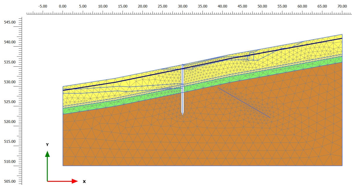
Figura 27: Fase 1. Fase geostatica iniziale con falda a -1.0 m da p.c.
