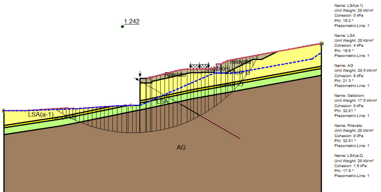
Figura 38: SLU(SLV)/GEO_stab A2+M2+R2-Combinazione fondamentale - Superficie di scorrimento critica
