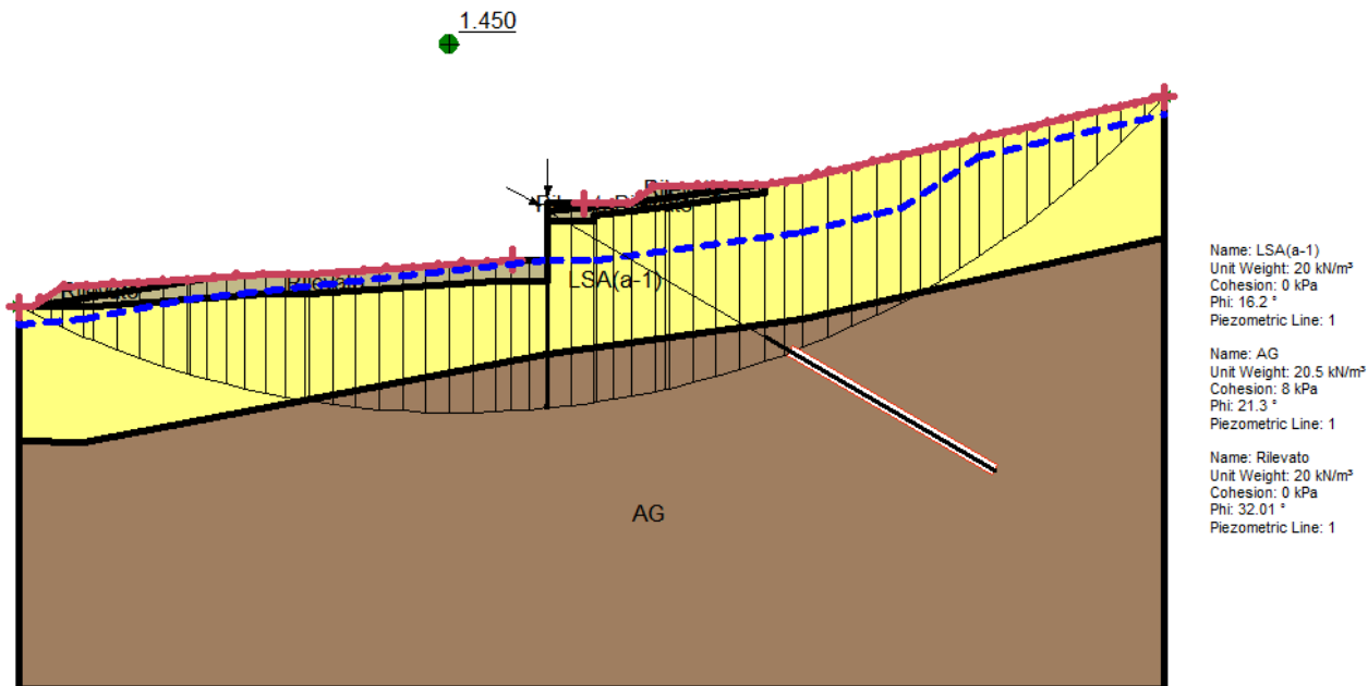
Figura 55: SLU(SLV)/GEO_stab A2+M2+R2-Combinazione sismica ( k_v < 0 )- - Superficie di scorrimento critica
