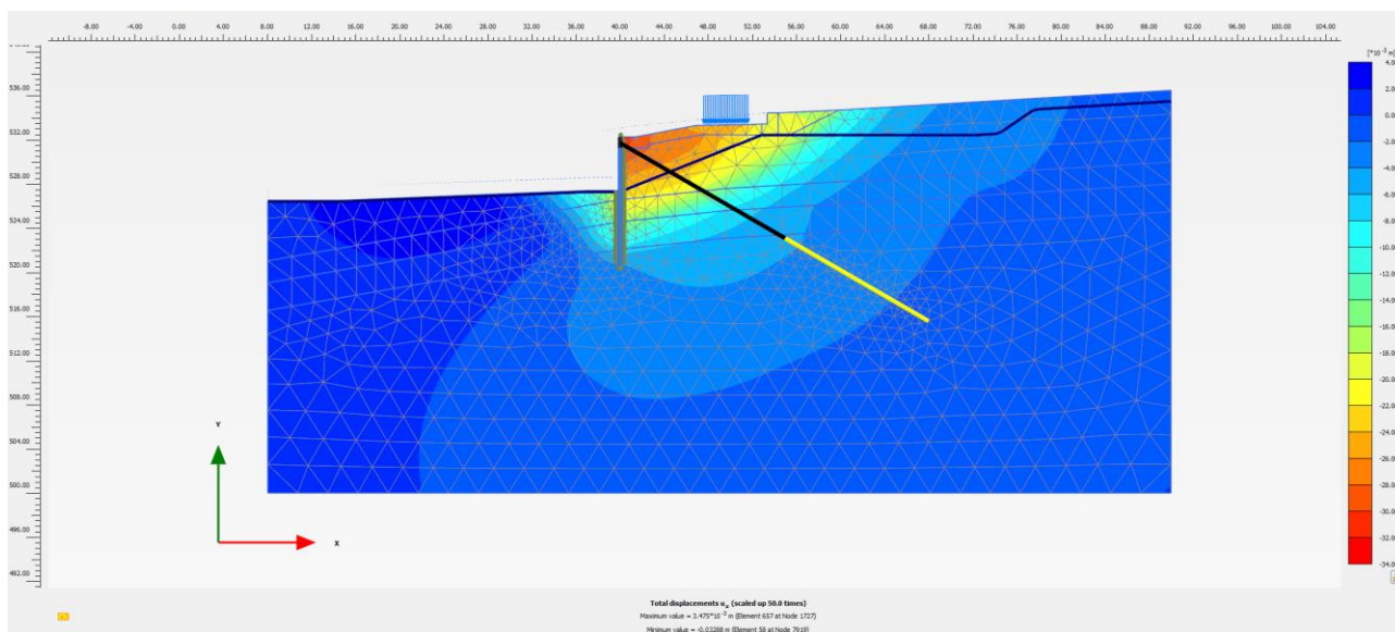
Figura 17: SLE-Combinazione frequente.
