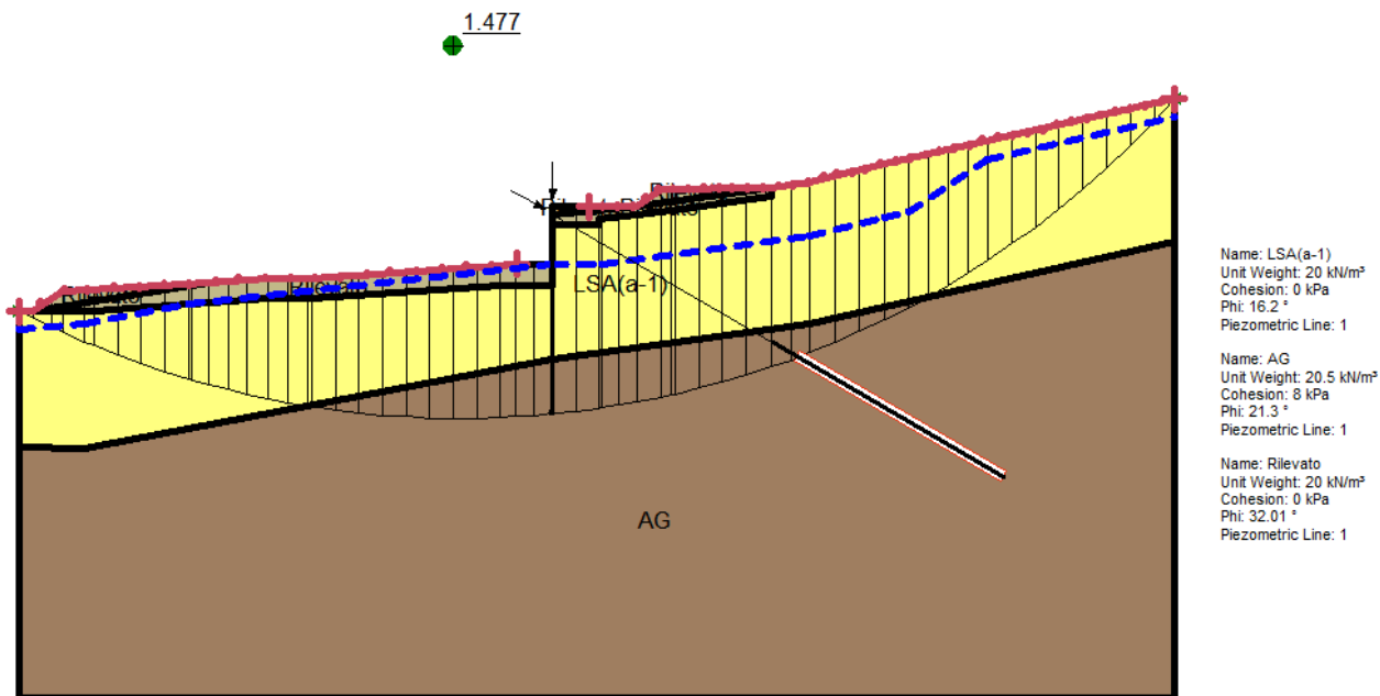
Figura 54: SLU(SLV)/GEO_stab A2+M2+R2-Combinazione sismica ( k_v > 0 )- Superficie di scorrimento critica
