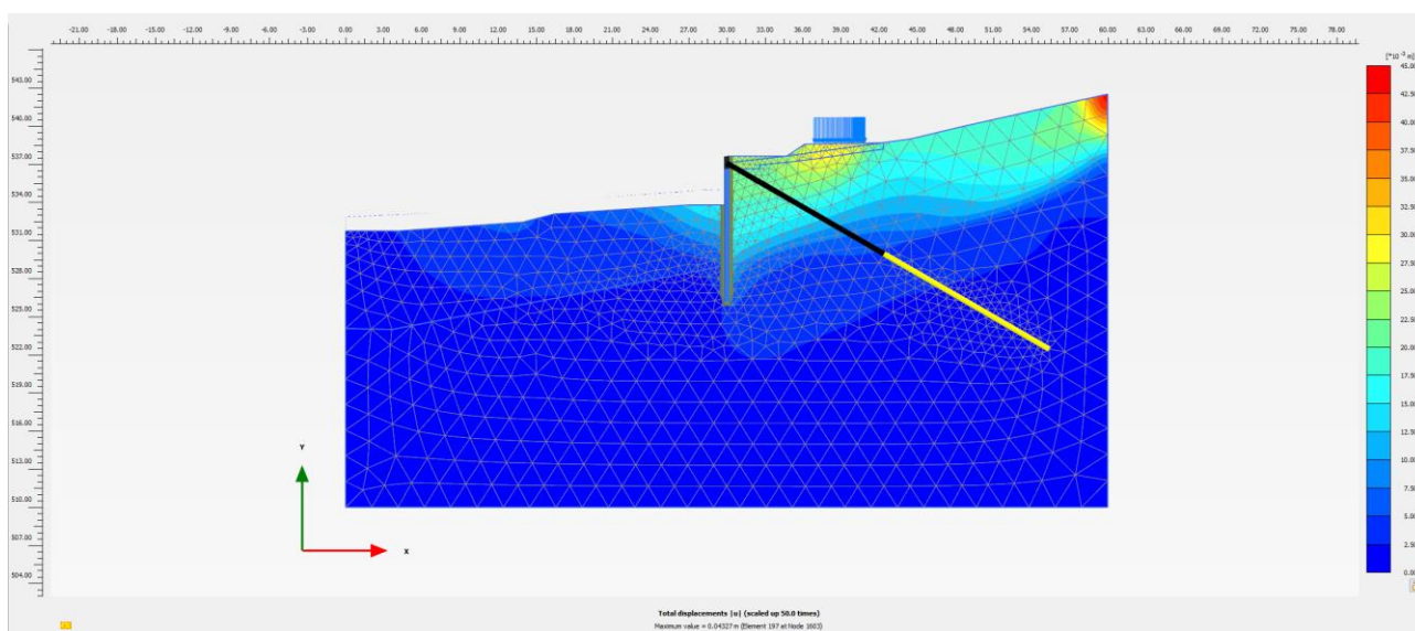
Figura 51: SLU(SLV)/GEO A2+M2+R1 - Combinazione fondamentale, campo di spostamenti
