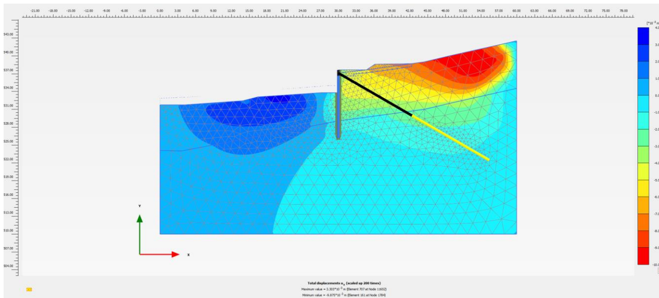
Figura 48: SLE-Combinazione quasi permanente.
