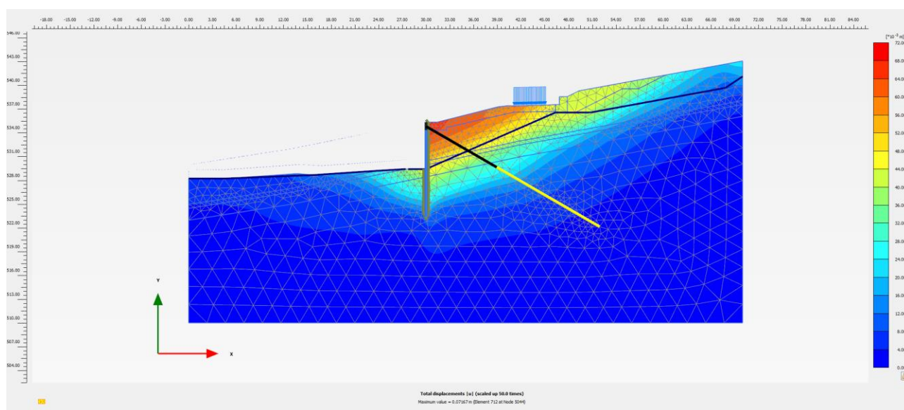
Figura 37: SLU(SLV)/GEO A2+M2+R1 – Combinazione sismica, campo di spostamenti
