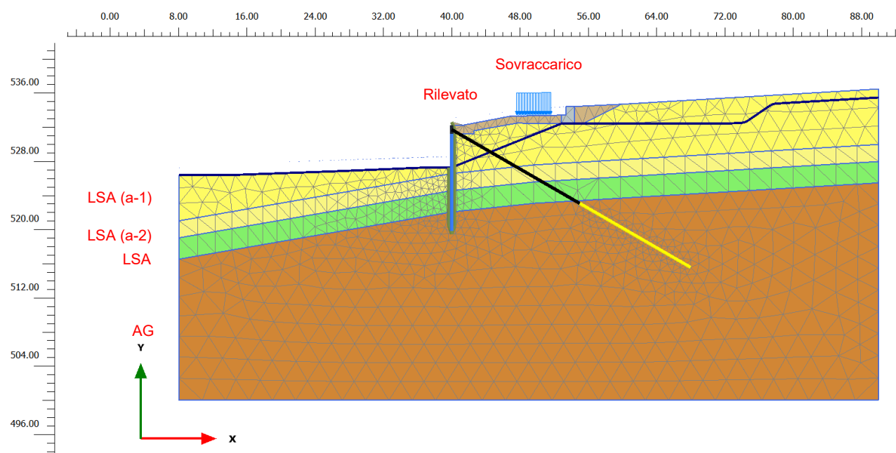
Figura 4: Sezione 28. Modello di calcolo Plaxis
