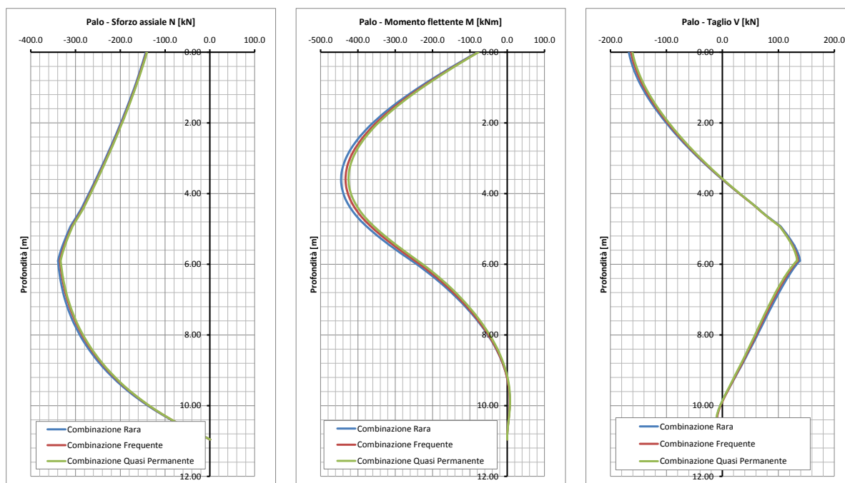
Figura 34: SLE-Pali. Diagrammi delle sollecitazioni
