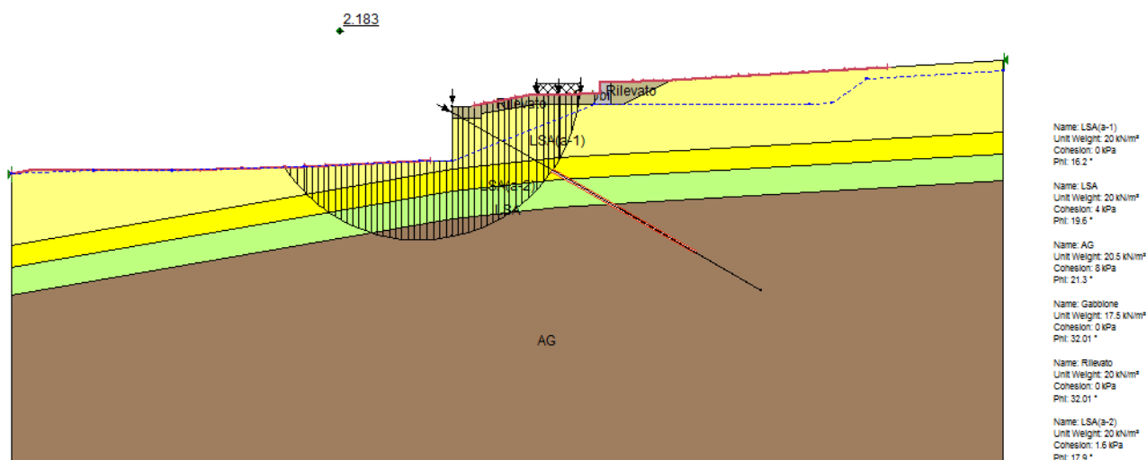
Figura 23: SLU(SLV)/GEO_stab A2+M2+R2-Combinazione fondamentale - Superficie di scorrimento critica
