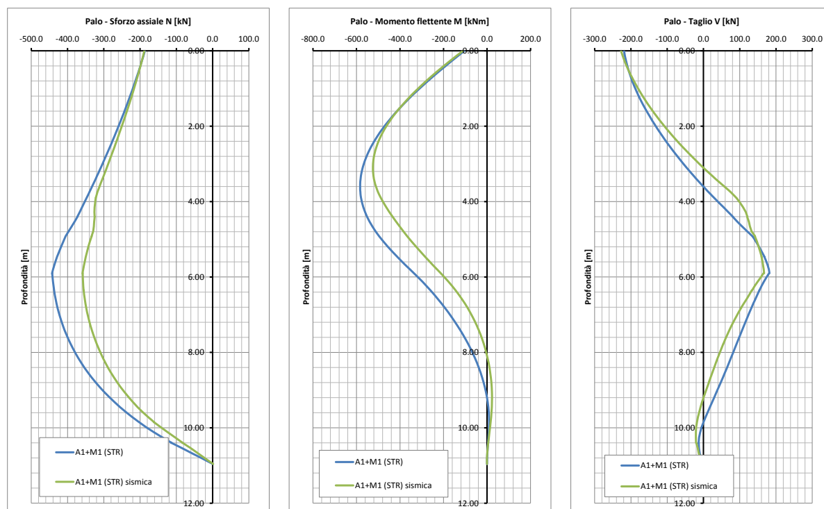
Figura 35: SLU(SLV)/STR A1+M1+R1-Pali. Diagrammi delle sollecitazioni
