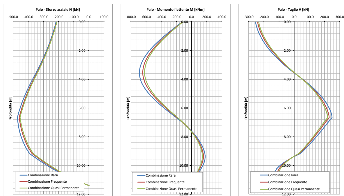
Figura 9: SLE-Pali. Diagrammi delle sollecitazioni
