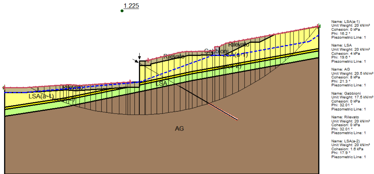
Figura 39: SLU(SLV)/GEO_stab A2+M2+R2-Combinazione sismica (kv>0)- Superficie di scorrimento critica
