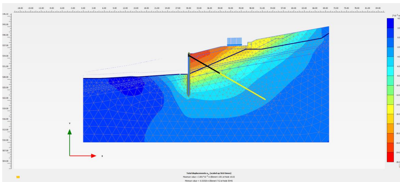
Figura 33: SLE-Combinazione quasi permanente.
