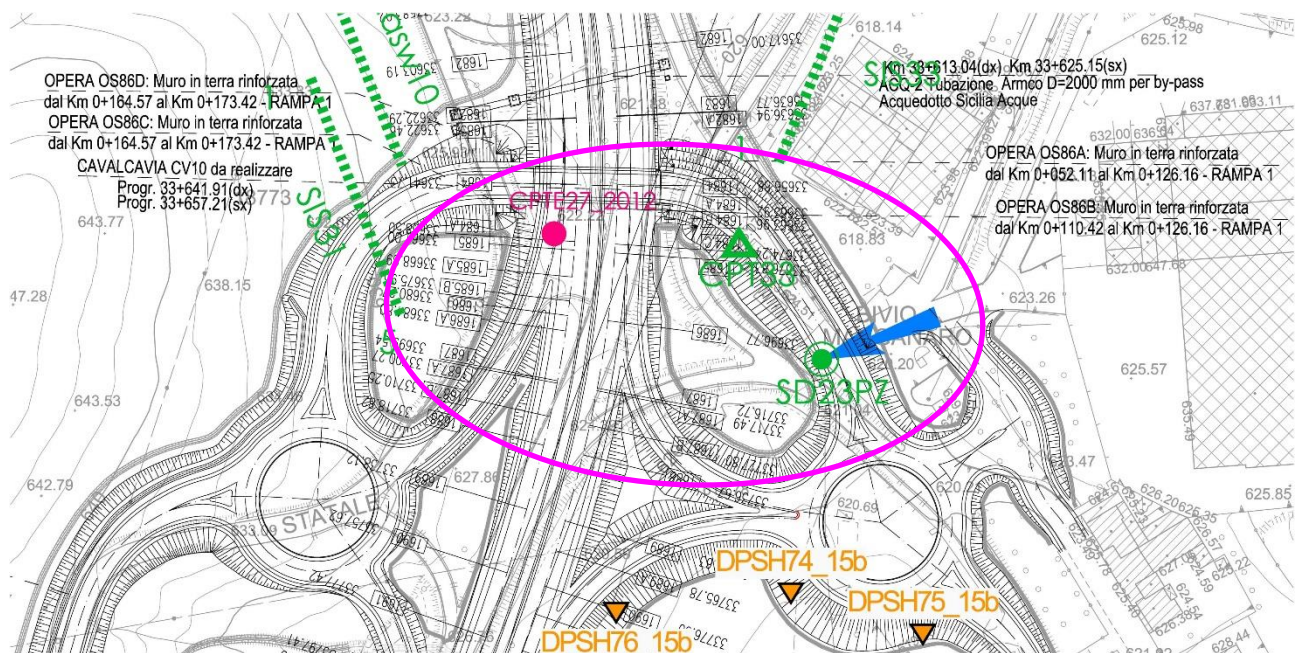
Fig. 8. Planimetria con ubicazione indagini geotecniche disponibili.
