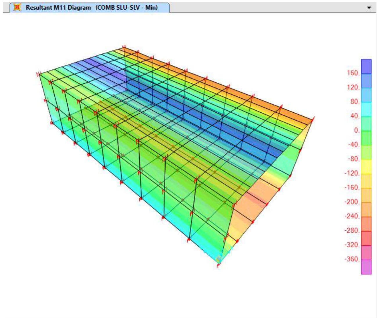
Figura 39 Diagramma dei momenti M11 min (Inviluppo SLU-SLV)
