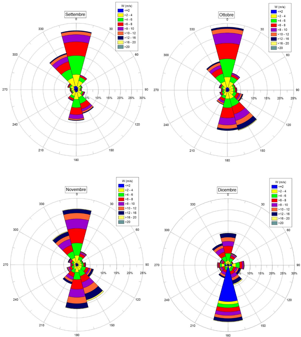
Figura A.3: Rose Mensili del Vento – Settembre, Ottobre, Novembre, Dicembre
