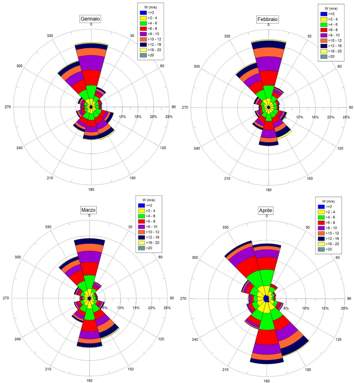
Figura A.1: Rose Mensili del Vento – Gennaio, Febbraio, Marzo, Aprile
