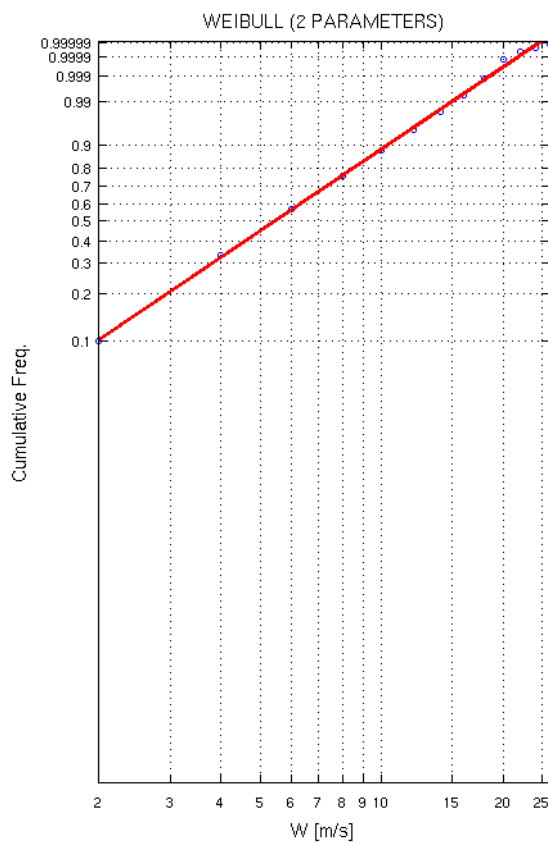
Figura 6.3: Fitting dei Dati di Vento con Distribuzione Biparametrica di Weibull
