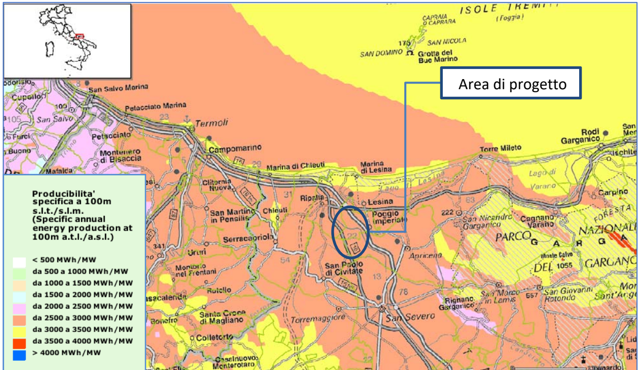
Impianto su Atlante eolico interattivo con produttività specifica a 100 m s.l.m.
