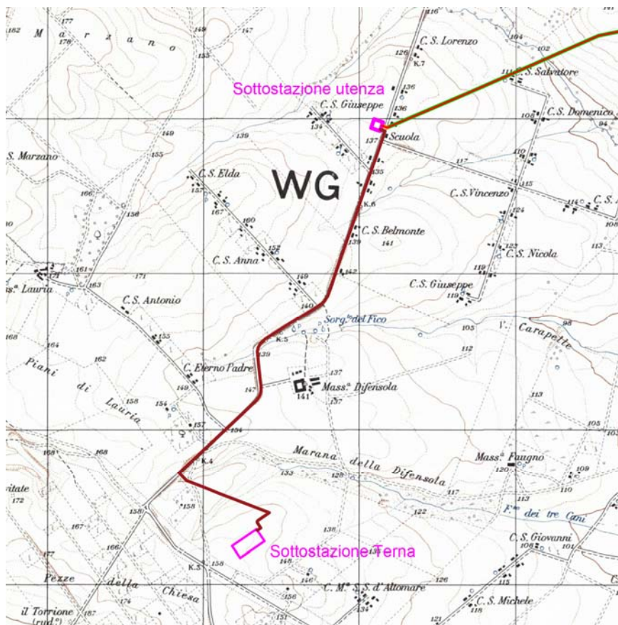
Inquadramento territoriale stazioni elettriche: Stazione Terna S.p.a. e Stazione di Utenza del parco eolico ATS ALEXINA.
