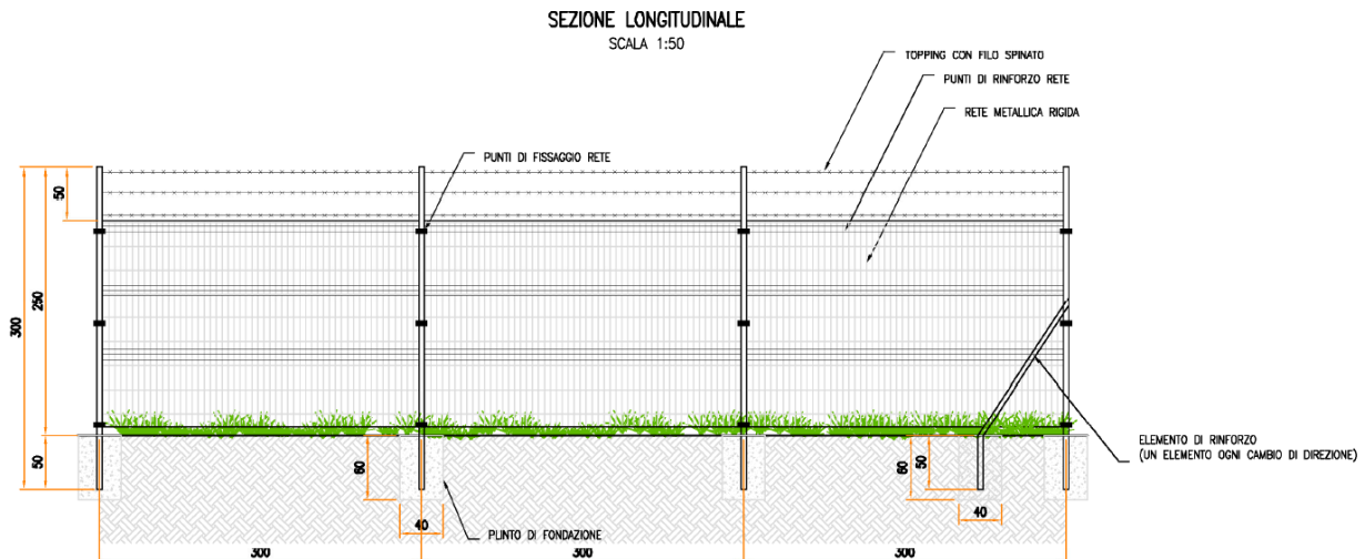
Figura 5.1: Tipico recinzione
