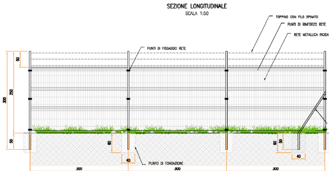
Figura 2.10: Particolare recinzione
