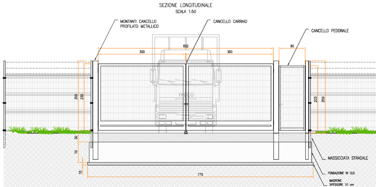
Figura 2.12: Particolare accesso
