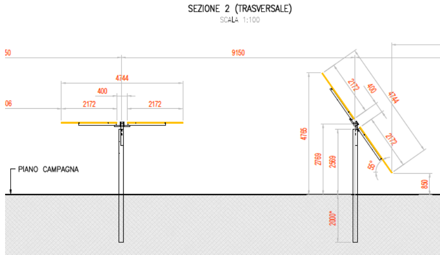
Figura 2.8: Particolare strutture di sostegno moduli
