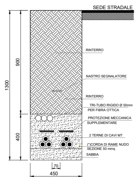
SEZIONE E-E CAVIDOTTO MT INTERRATO - 2 TERNE DI CAVI PERCORSO IN BANCHINA SOTTO STRADA COMUNALE/VICINALE
