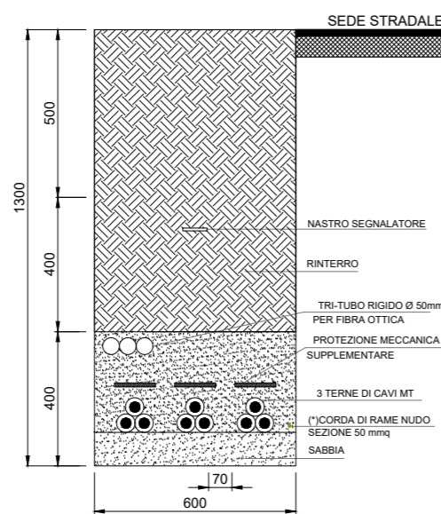
SEZIONE G-G CAVIDOTTO MT INTERRATO - 3 TERNE DI CAVI PERCORSO IN BANCHINA SOTTO STRADA COMUNALE/VICINALE
