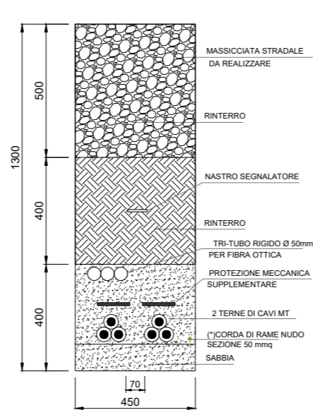
SEZIONE D-D CAVIDOTTO MT INTERRATO - 2 TERNE DI CAVI PERCORSO SOTTO STRADA IN FASE ESERCIZIO
