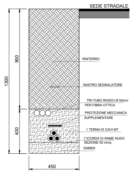
SEZIONE B-B CAVIDOTTO MT INTERRATO - 1 TERNA DI CAVI PERCORSO IN BANCHINA STRADA VICINALE/COMUNALE
