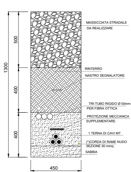
SEZIONE C-C CAVIDOTTO MT INTERRATO - 1 TERNA DI CAVI PERCORSO SOTTO STRADA COMUNALE/VICINALE
