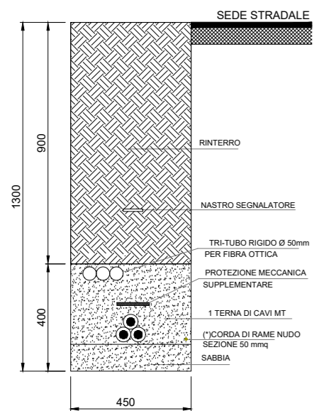
SEZIONE F-F CAVIDOTTO MT INTERRATO - 1 TERNA DI CAVI PERCORSO IN BANCHINA SOTTO STRADA COMUNALE/VICINALE
