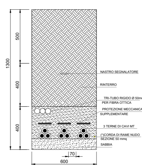
SEZIONE I-I CAVIDOTTO MT INTERRATO - 3 TERNE DI CAVI PERCORSO IN TERRENO
