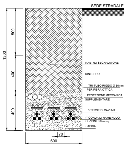
SEZIONE H-H CAVIDOTTO MT INTERRATO - 3 TERNE DI CAVI PERCORSO IN BANCHINA SOTTO STRADA STATALE
