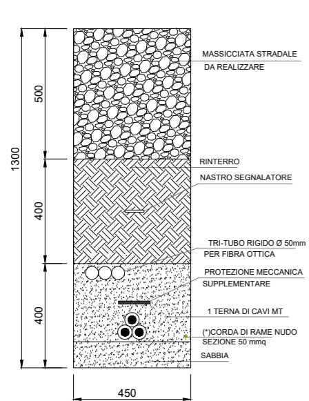
SEZIONE A-A CAVIDOTTO MT INTERRATO - 1 TERNA DI CAVI PERCORSO SOTTO STRADA IN FASE ESERCIZIO
