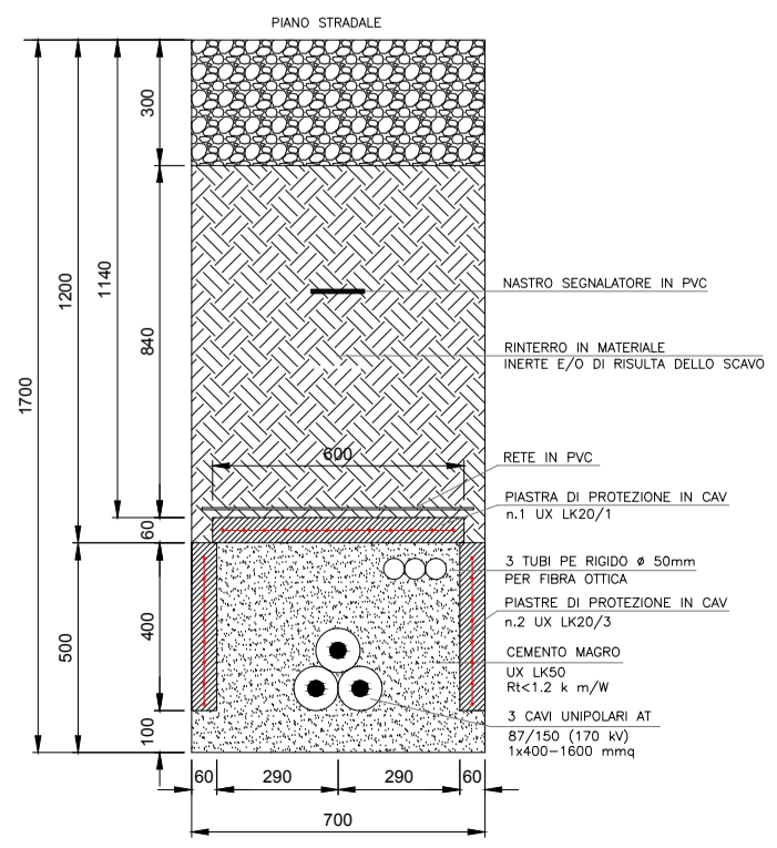
PARTICOLARE A CAVIDOTTO AT SINGOLA TERNA-PERCORSO IN MASSICIATA scala 1:20
