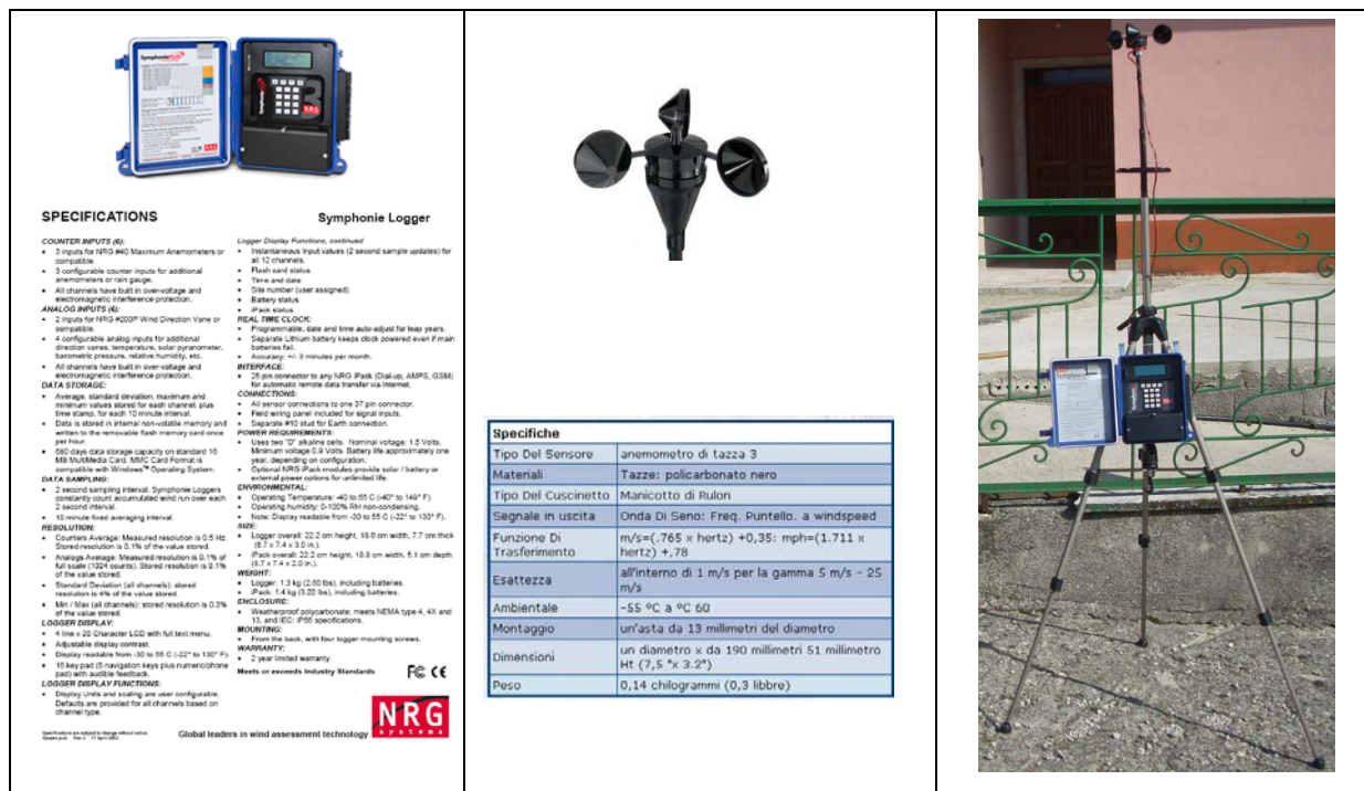
Figura 2: Stazione meteo portatile utilizzata- l'altezza di misura dei sensori è 1,5 m; Specifiche tecniche dell'NRG #40 Maximum caratteristiche tecniche DATA LOGGER
