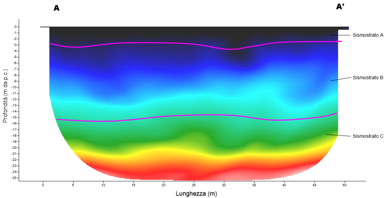
Fig. 9 – Interpretazione sezione tomografica del profilo AA'
