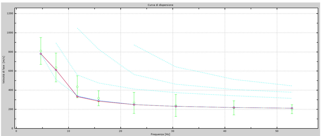
Fig.22 - Velocità numeriche – punti sperimentali (verde), modi di Rayleigh (ciano), curva apparente (blu), curva numerica (rosso). La percentuale di differenza è: 9%.
