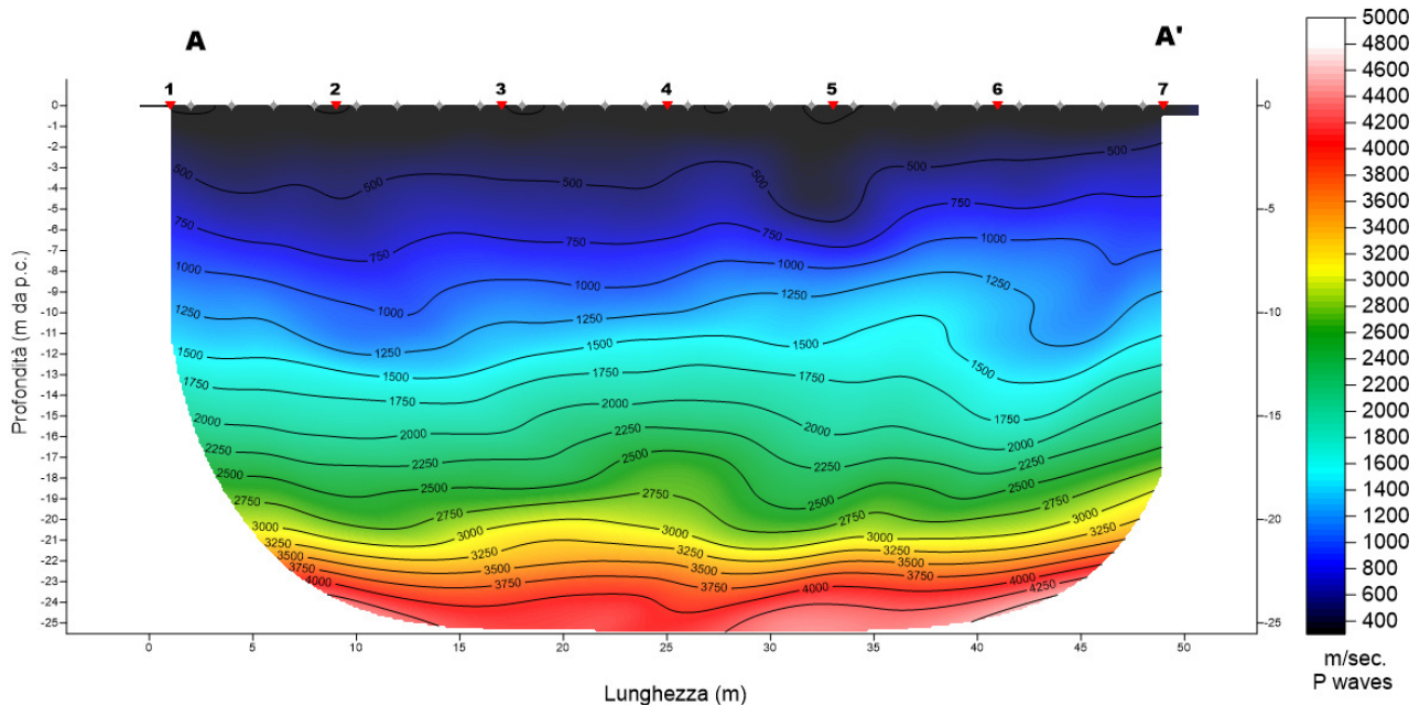
Fig. 8 – Sezione tomografica del profilo AA'
