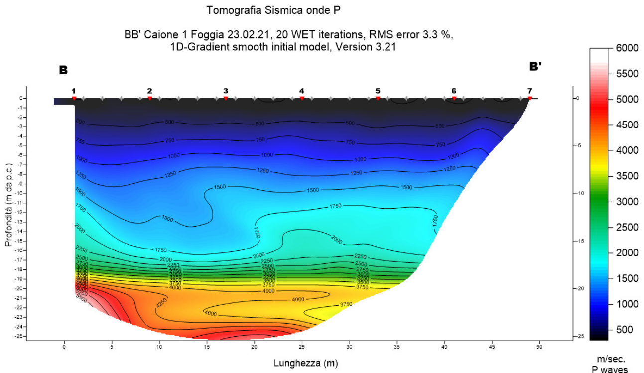
Fig. 11 – Sezione tomografica del profilo BB'
