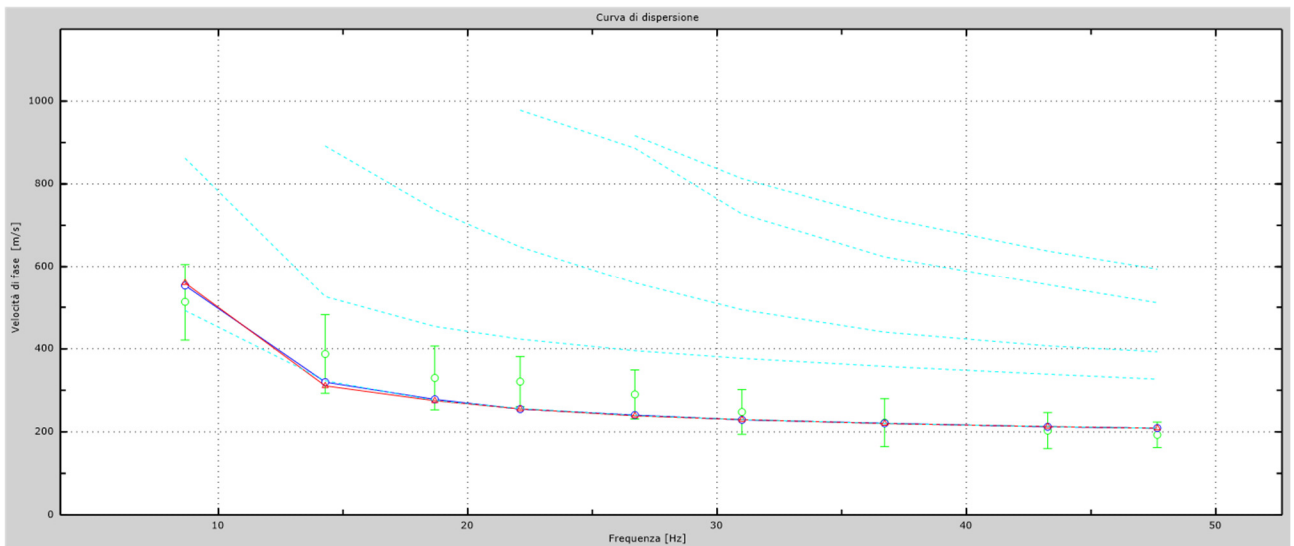
Fig.18 - Velocità numeriche – punti sperimentali (verde), modi di Rayleigh (ciano), curva apparente (blu), curva numerica (rosso). La percentuale di differenza è: 13%.
