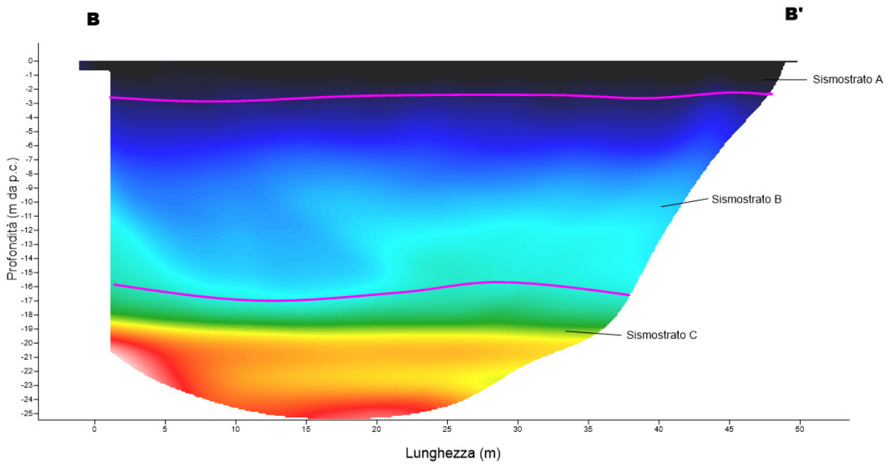
Fig. 8 – Interpretazione sezione tomografica del profilo BB'
