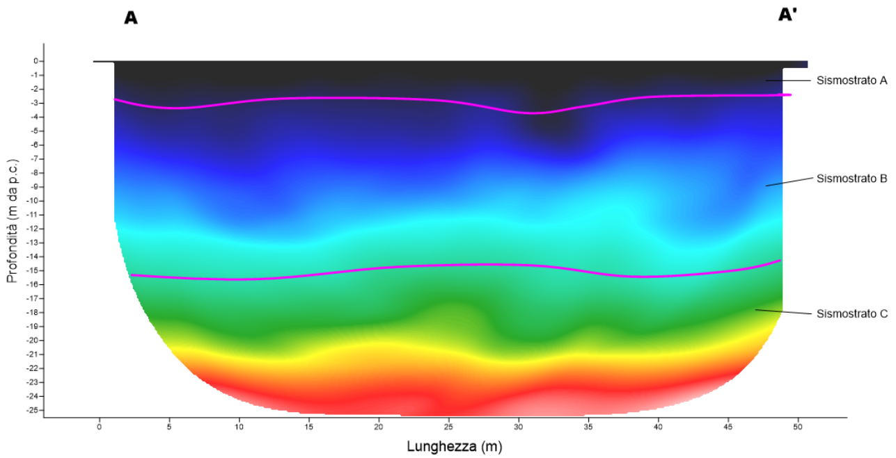
Fig. 7 – Interpretazione sezione tomografica del profilo AA'
