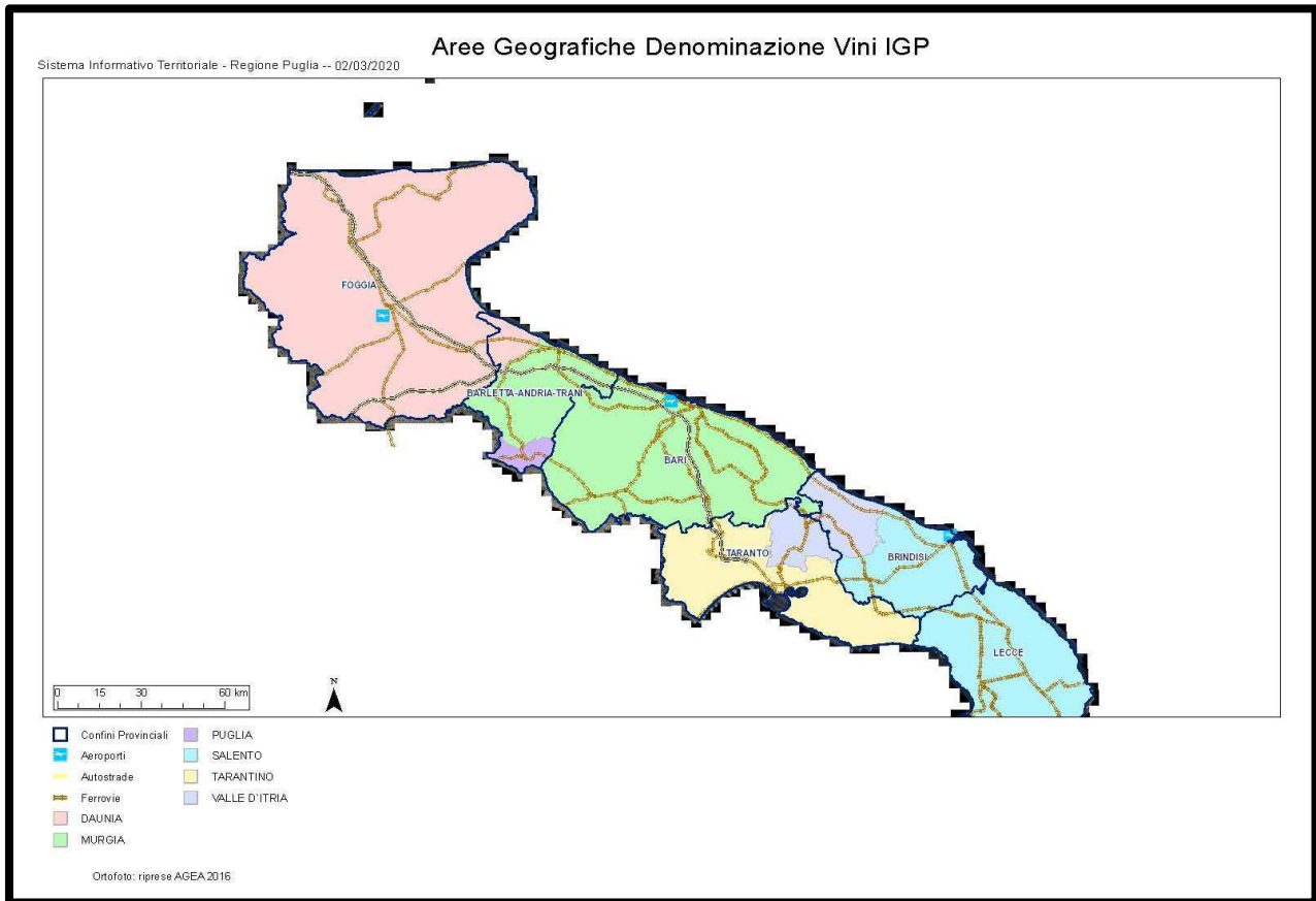
Tav. 26 – Cartografia delle perimetrazioni vini IGP Puglia(fonte Agea)
