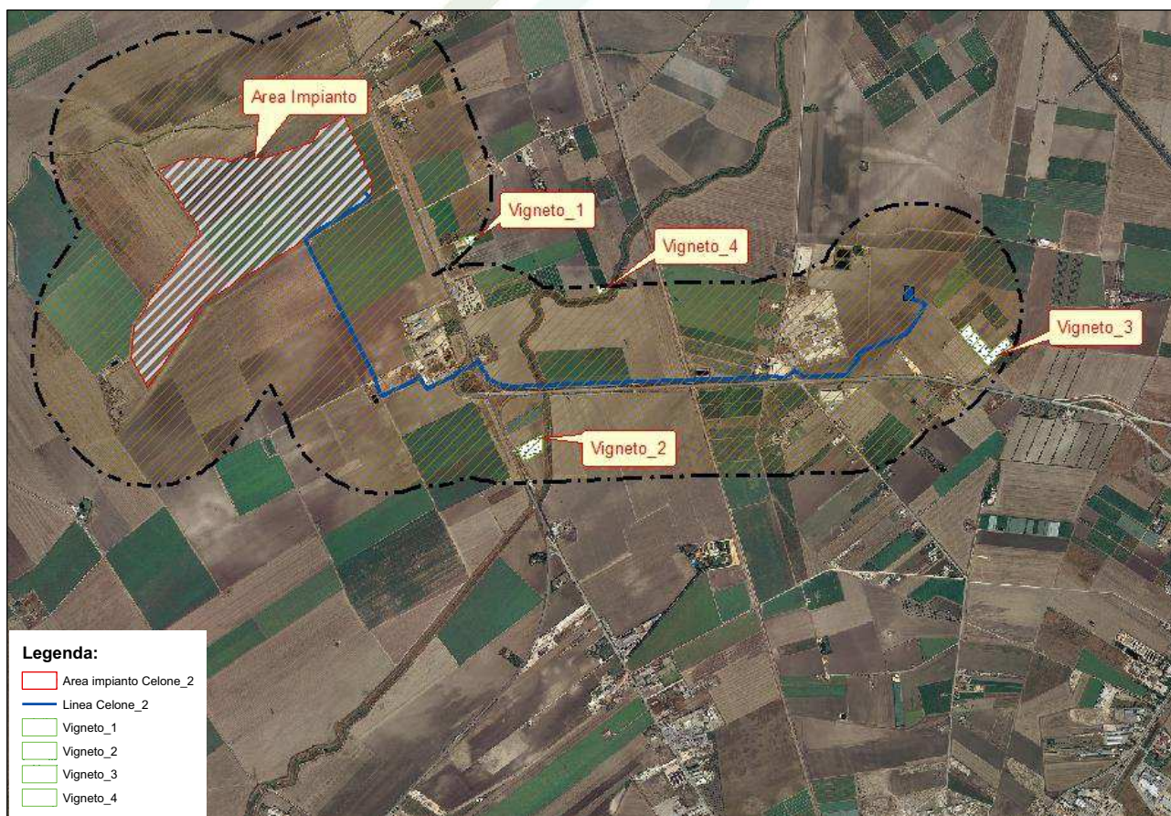
Tav.29 – Superfici vitate all'interno dell'area buffer mt. 500 dell'area di interesse e nell'immediato intorno. Scala 1:25.000
