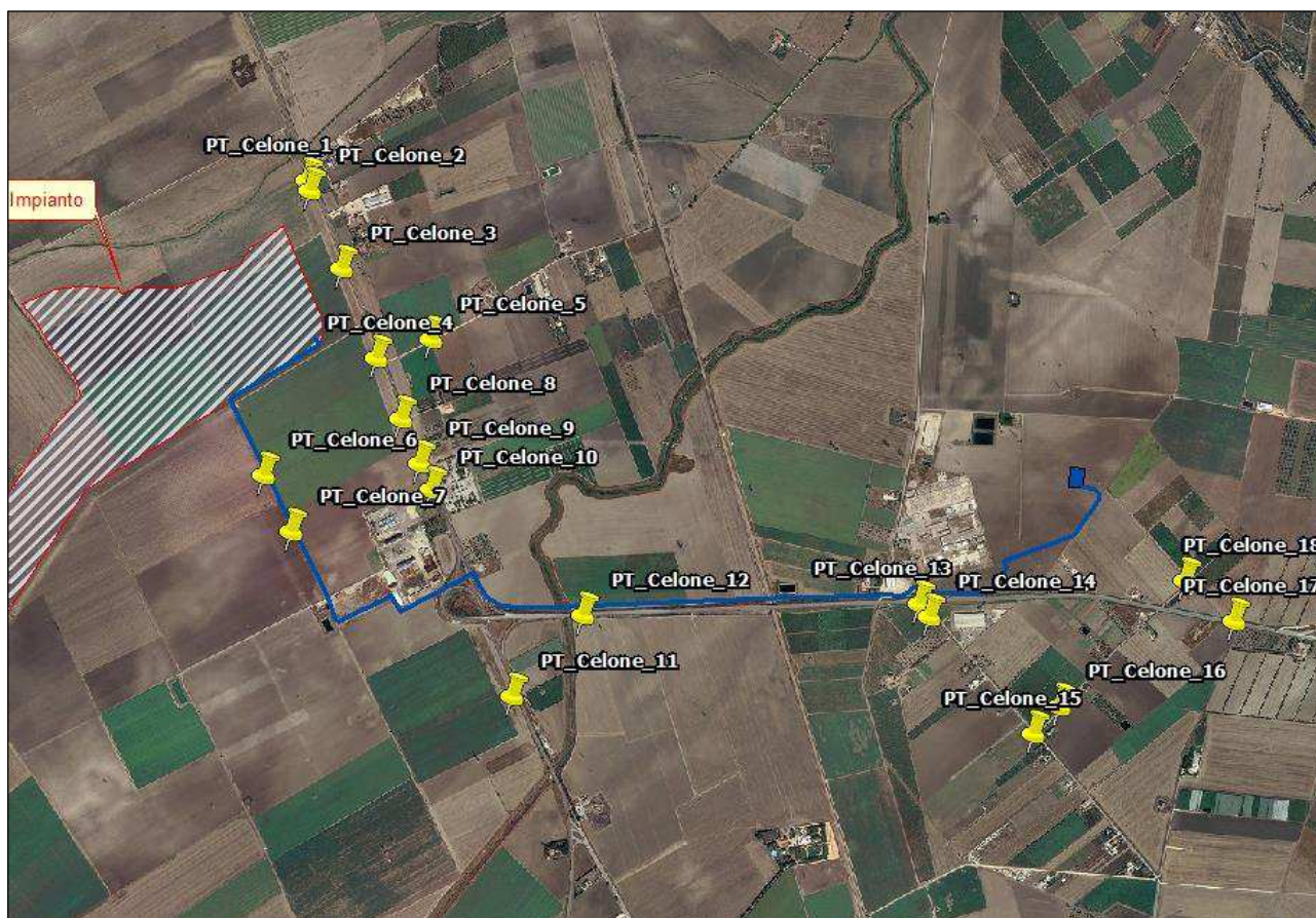
Tav.30- Punti di ripresa fotografica con georeferenziazione. Scala 1:20.000
