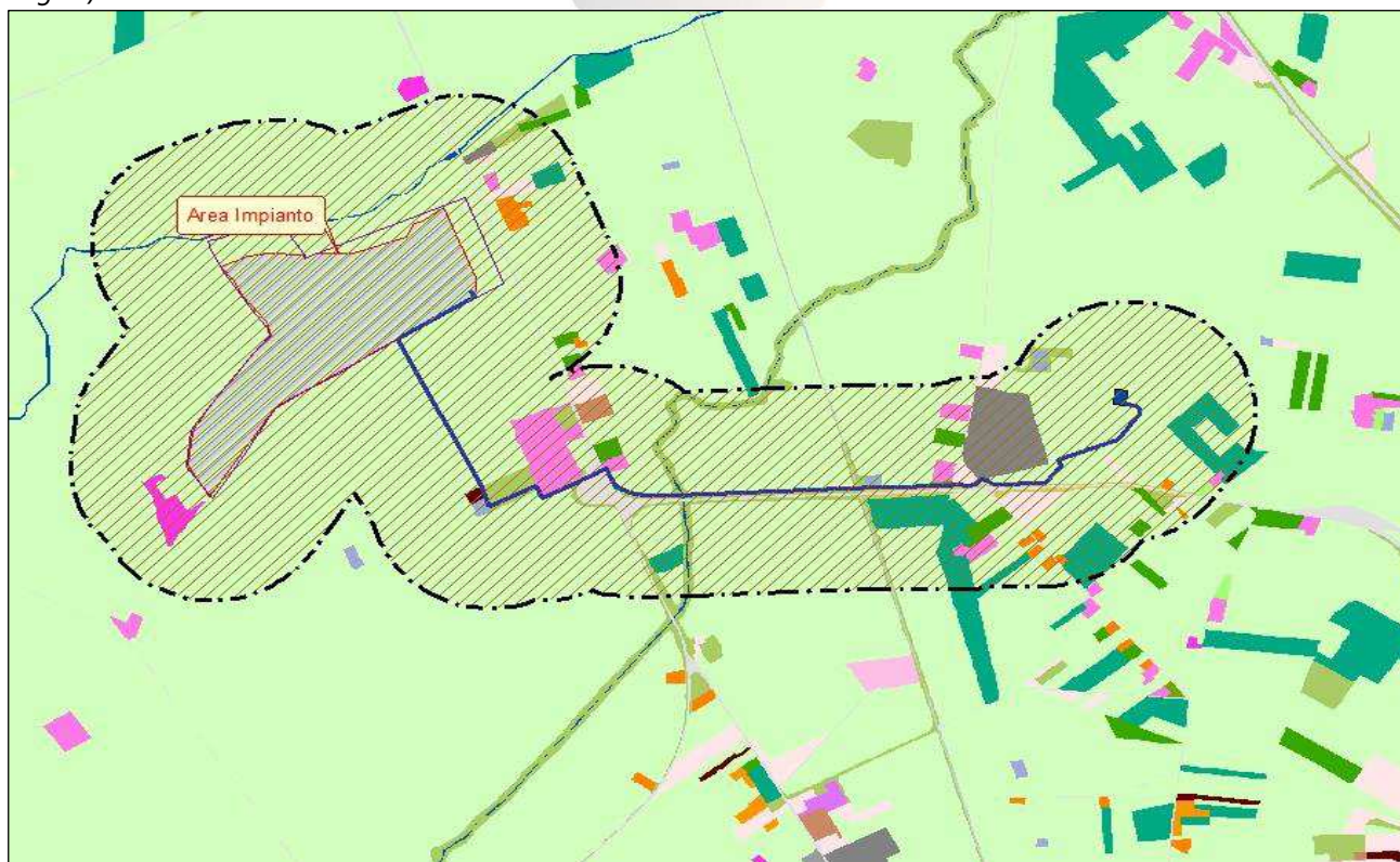
Tav. 28– Inquadramento territoriale su carta uso del solo, area buffer mt. 500 scala 1:25.000 (Fonte dati SIT Puglia)
