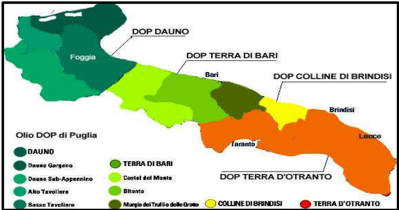
Tav. 24 – Cartografia delle perimetrazioni olio DOP Puglia (Fonte Agea)
