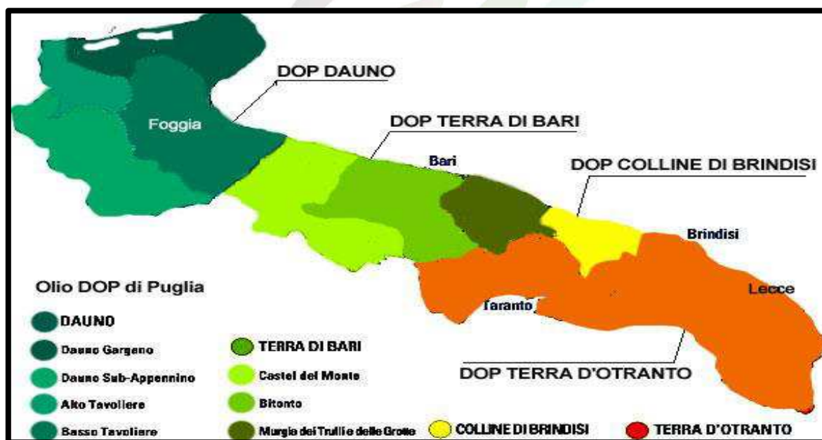
Tav. 15 - Cartina delle perimetrazioni olio DOP Puglia
