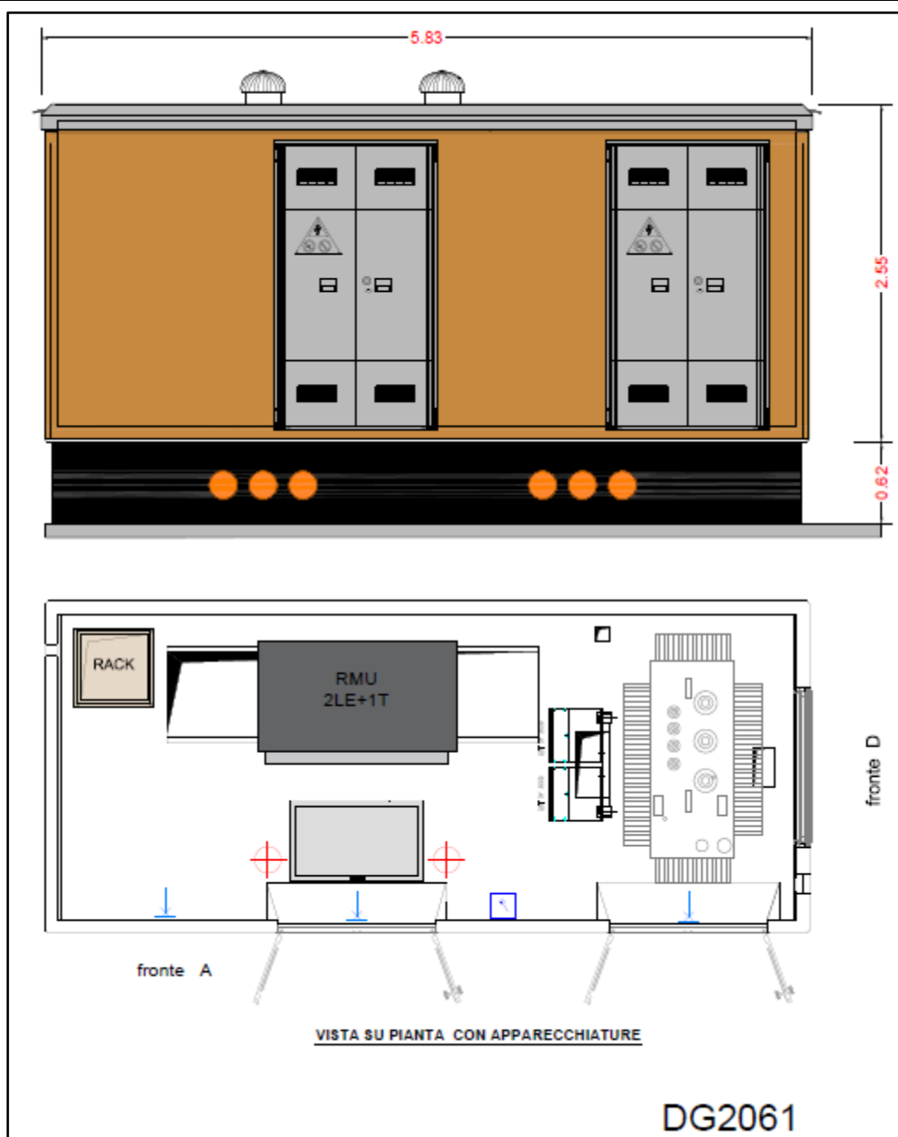
Figura 26 Tipologico Cabina di Sezionamento
