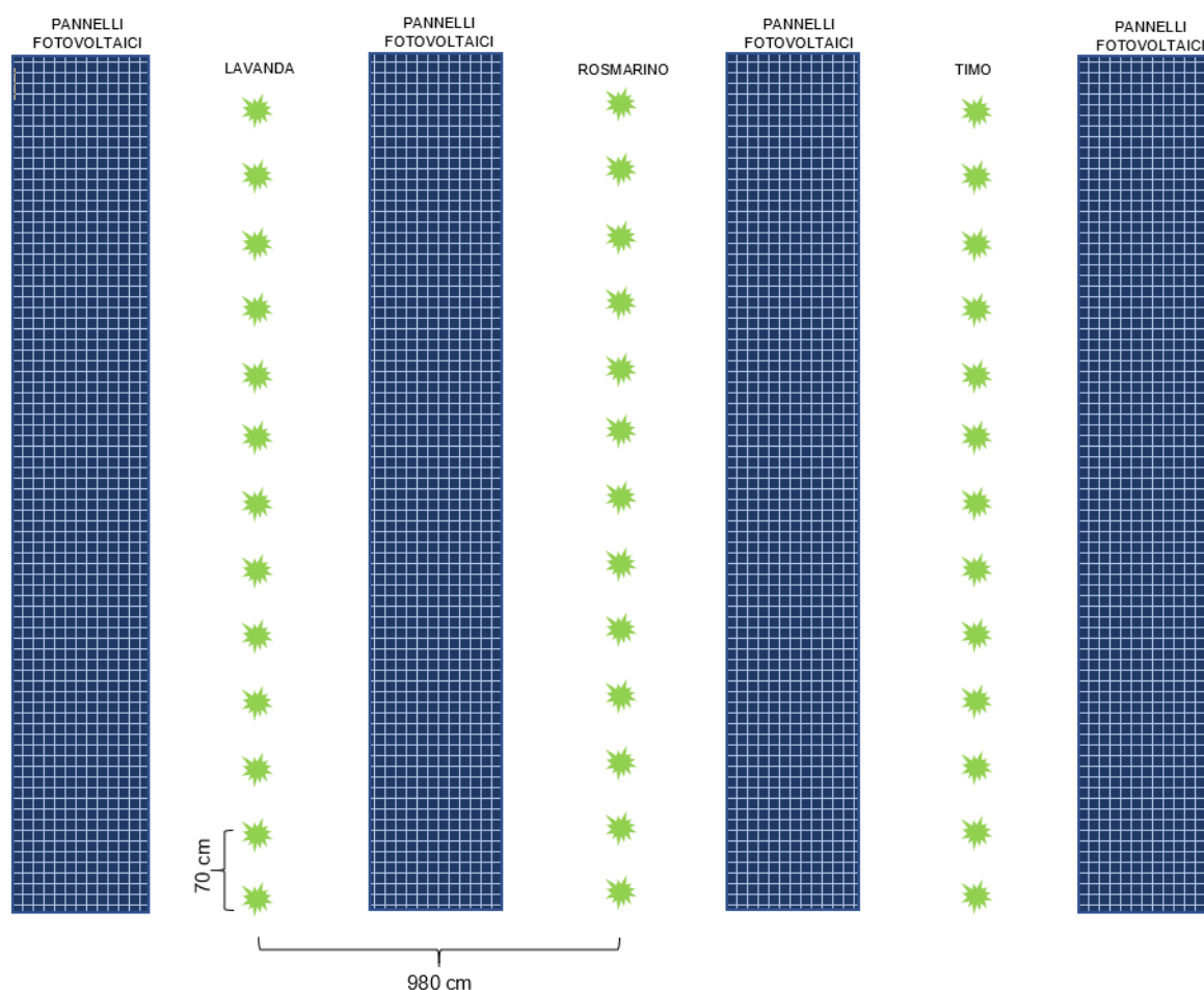
Figura 37 - Porzione dell'area oggetto di intervento, vista dall'alto dell'impianto fotovoltaico integrato con apiario
