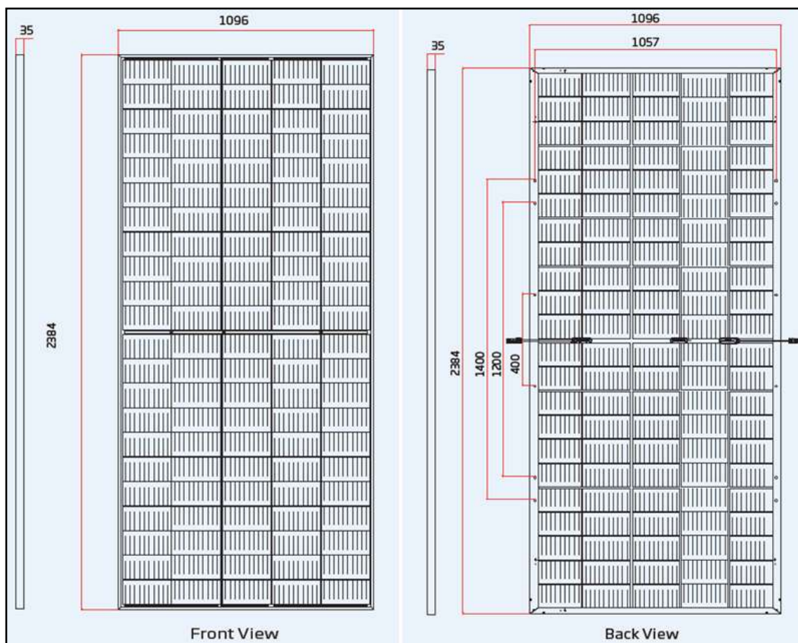
Figura 13 Dimensioni modulo "TSM-DEG19C.20"
