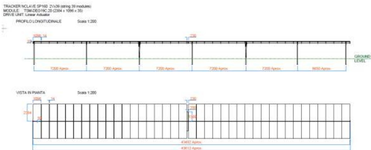
Figura 15: Configurazione Struttura tracker 2x39
