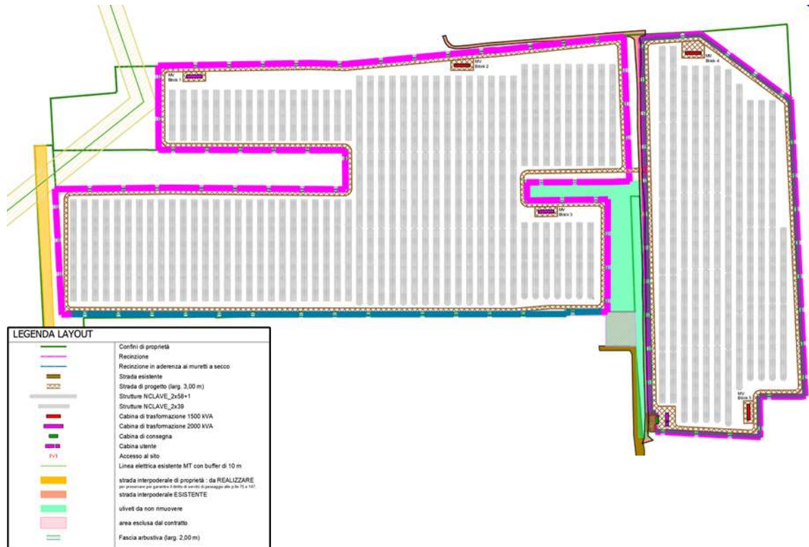
Figura 19: Area di impianto – In magenta le recinzioni aventi altezza pari a 2,65 m.
