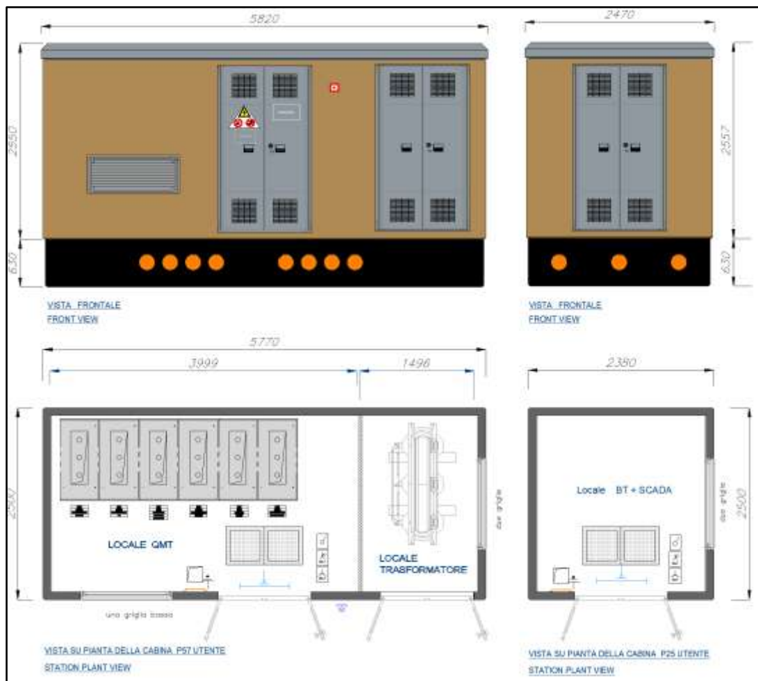
Figura 27 Cabina Utente (MT -TSA) e (SCADA - bt)
