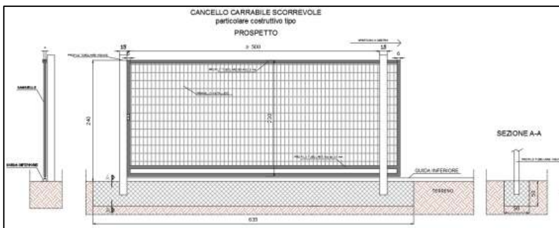
Figura 18 Cancelli carrabili scorrevoli (rif. doc. XXX_ElaboratoGrafico_0_23 - Particolari costruttivi recinzione)
