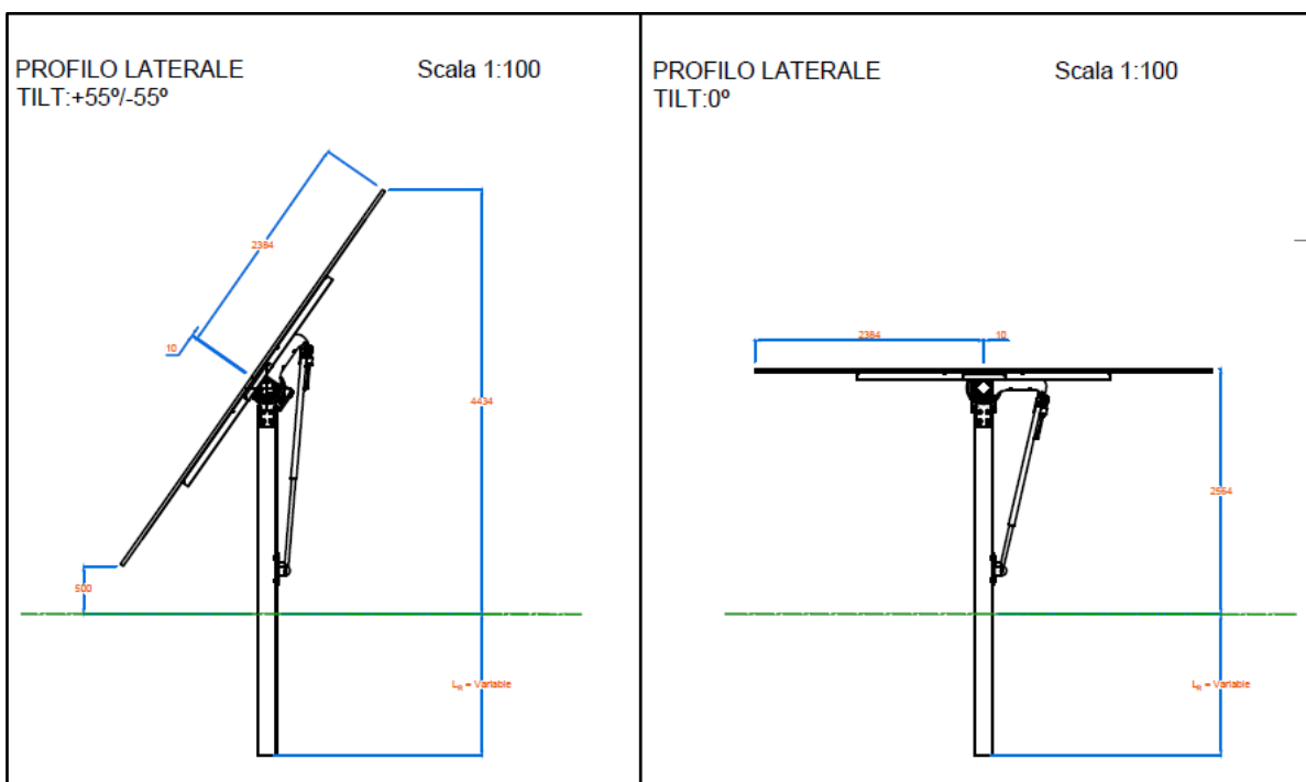
Figura 16: Sezione tipo Struttura tracker
