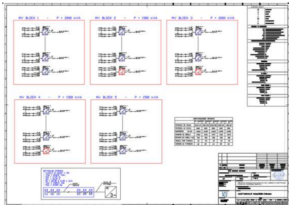
Figura 28 schema elettrico unifilare generale Grottaglie
