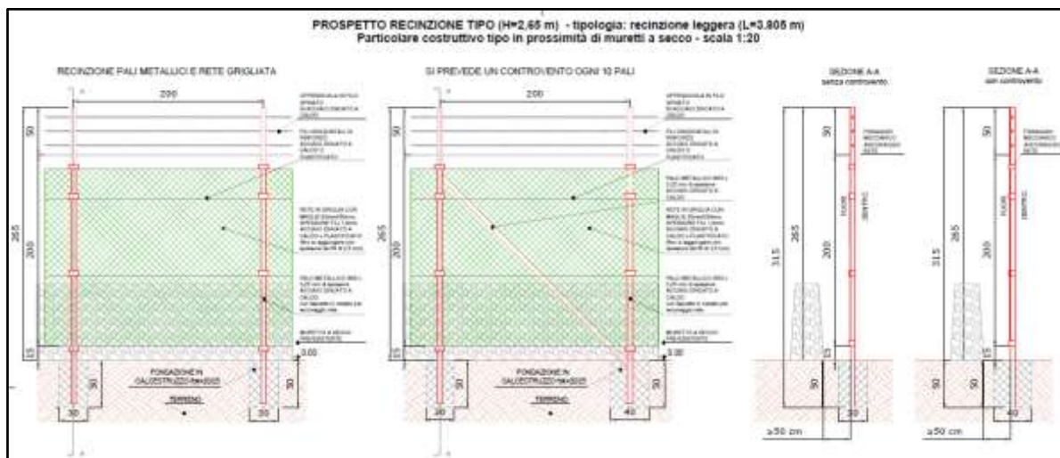
Figura 21 Rappresentazione della recinzione tipo.
