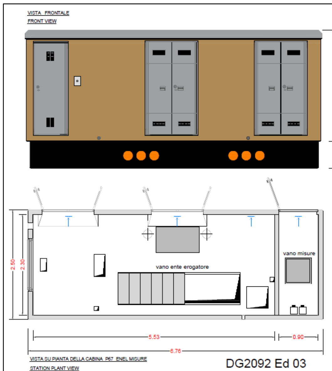
Figura 25 Tipologico Cabina di Consegna
