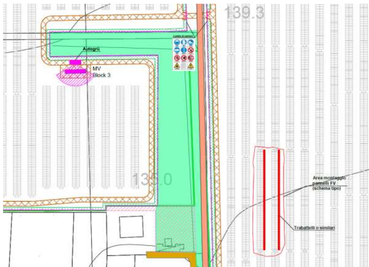
Figura 12 Layout di cantiere – dettaglio
