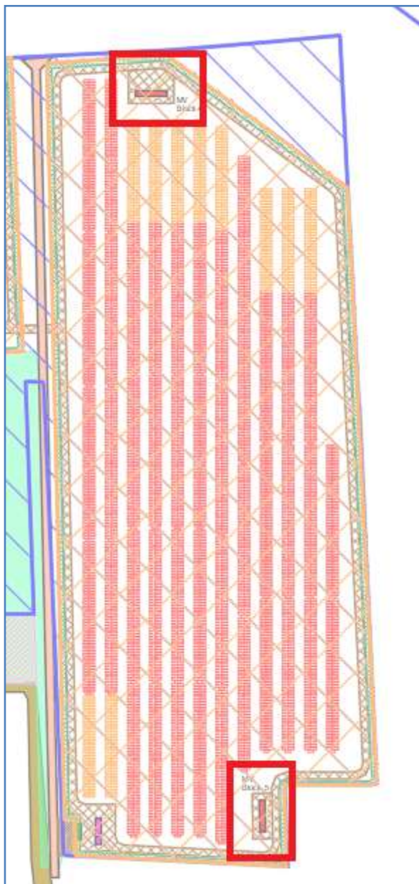
Figura 24 Individuazione dei cabinati di trasformazione di riferimento per l'area a sud
