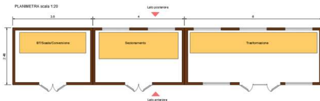
Figura 22 Rappresentazione della cabina di trasformazione
