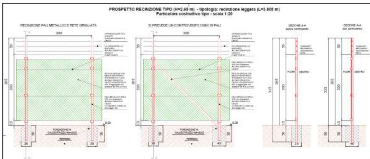
Figura 41 Rappresentazione della recinzione tipo.
