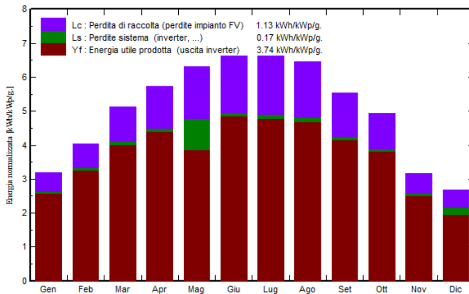
Produzione normalizzata (per kWp installato): Potenza nominale 27298 kWp
