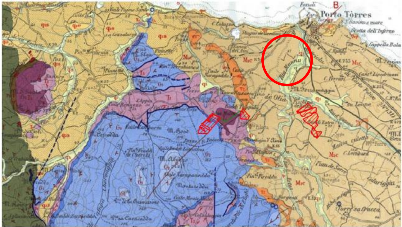
Stralcio della Carta Geologica d'Italia – Foglio 179 – Nel cerchio rosso l'area della SSE
