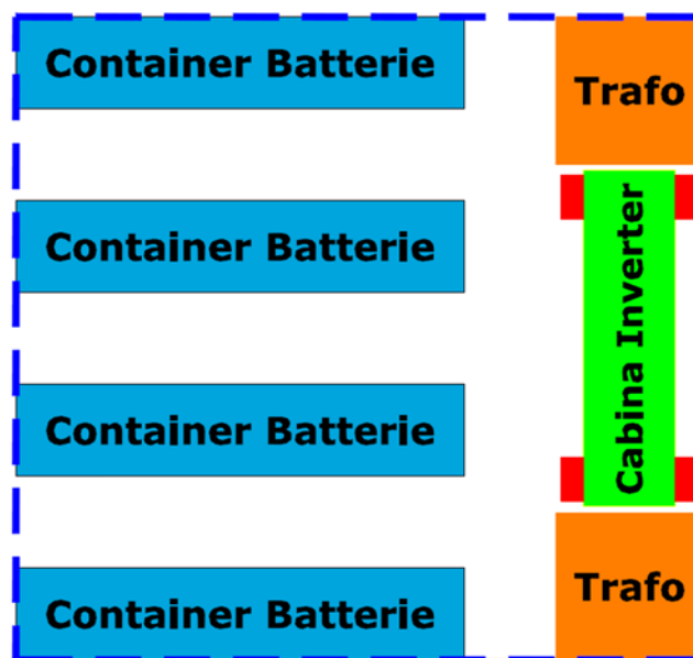
Schema Modulo Sistema di Accumulo
