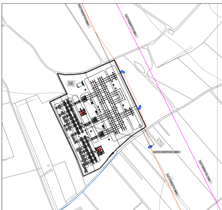
In blu i sostegni della linea 380 kV
