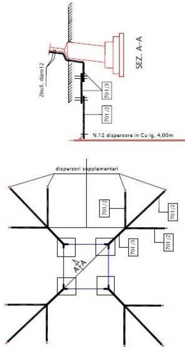
Figura 9 Tipico messa a terra sostegni
