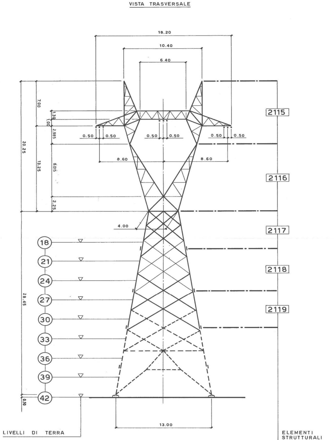
Figura 1 Schema sostegno di amarro
