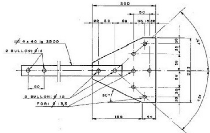
Figura 11 Tipico messa a terra sostegni
