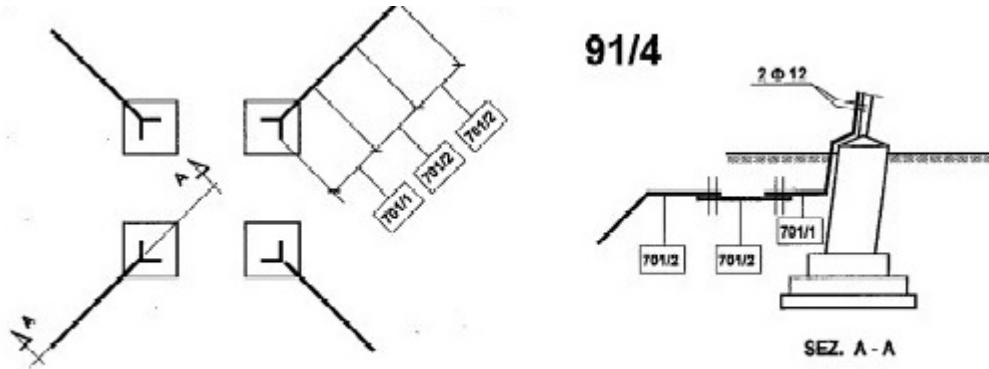
Figura 7 Tipico messa a terra sostegni
