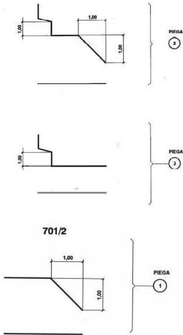
Figura 10 Tipico messa a terra sostegni
