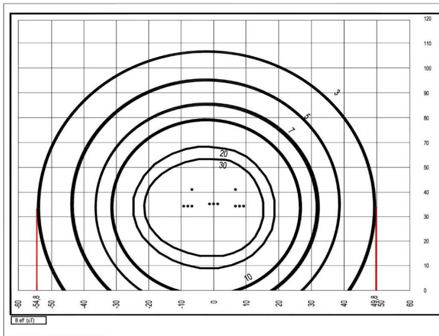
Figura 3: Curve di isocampo a 3 \mu T in una sezione perpendicolare all'asse linea per un sostegno in amarro 380 kV. DPA = 54,80m.
