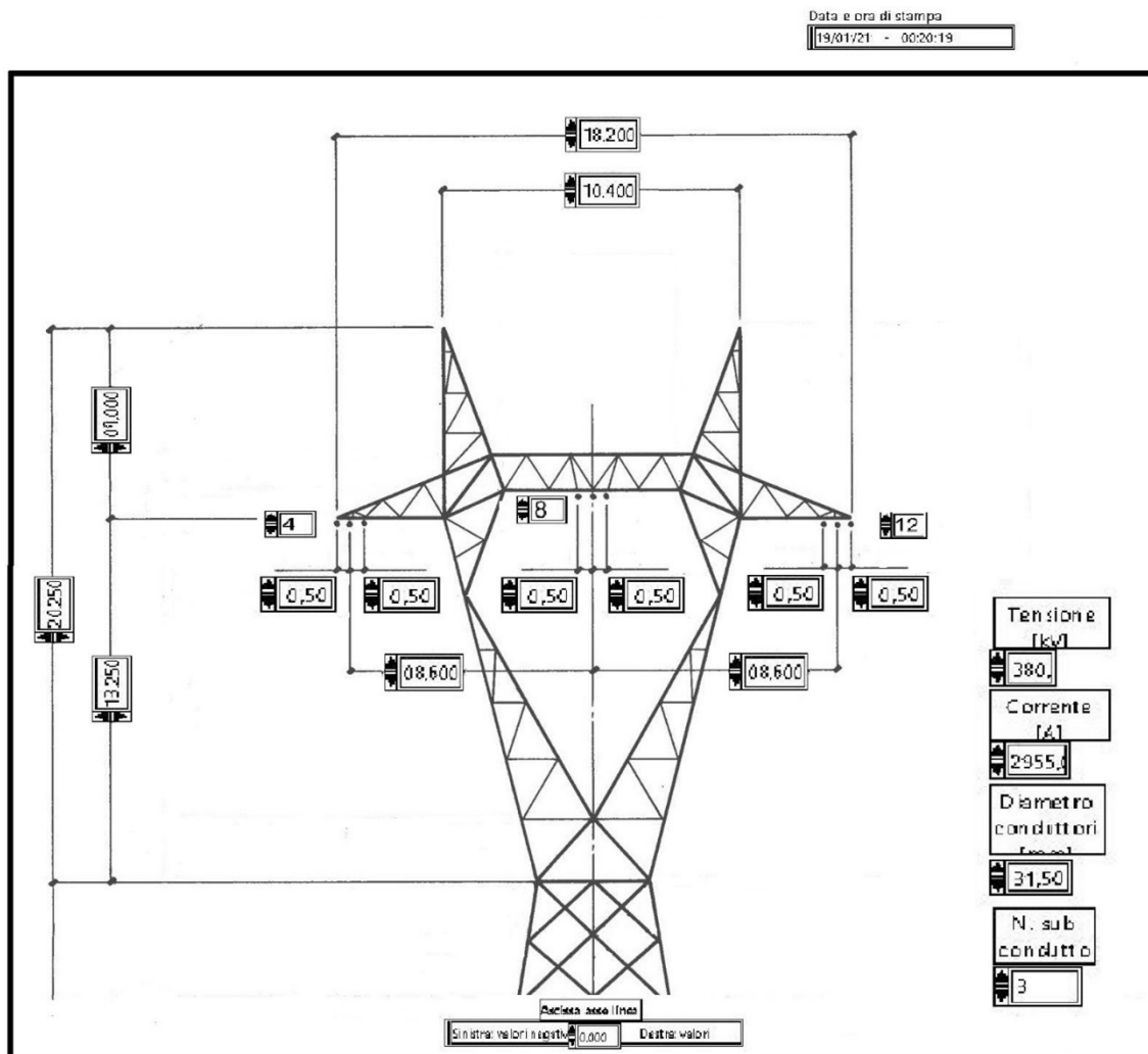
Figura 2: Geometria testa del sostegno in amarro 380 kV.
