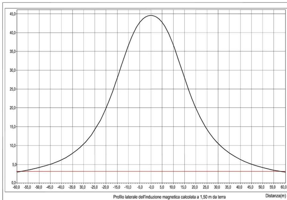
Figura 1: andamento dell'induzione magnetica in una sezione perpendicolare agli assi delle linee, calcolata ad 1,5 m dal suolo nel caso di franco minimo pari a 10,0 m per il sostegno di amaro 380 kV. (in rosso l'obiettivo di qualità pari a 3 \mu T).
