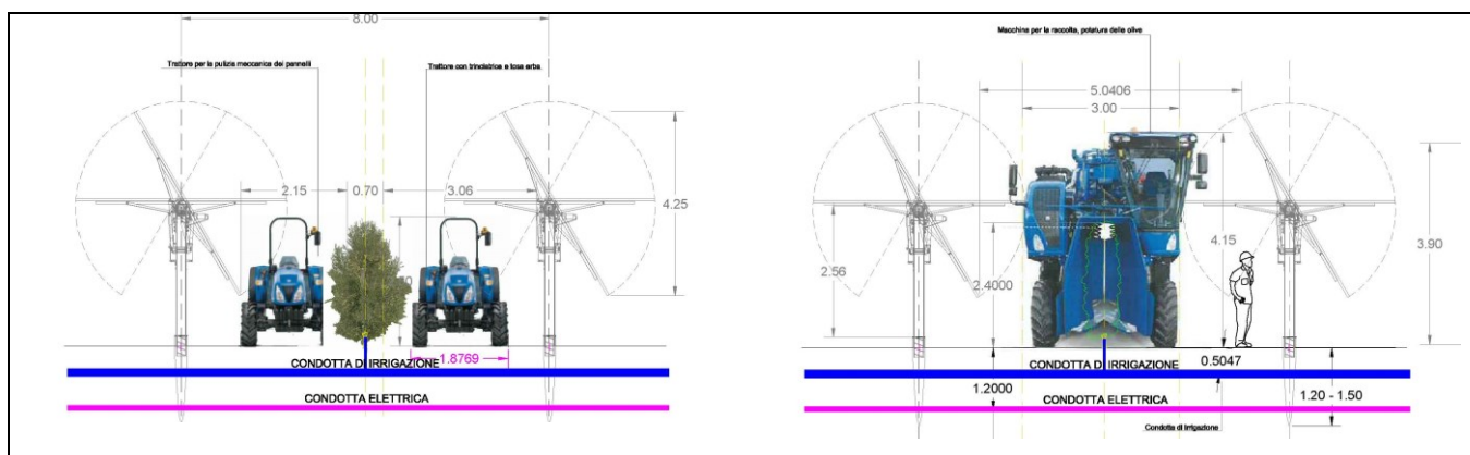
Profilo dell'interfila dell'impianto olivicolo (larghezza m. 8.0)
