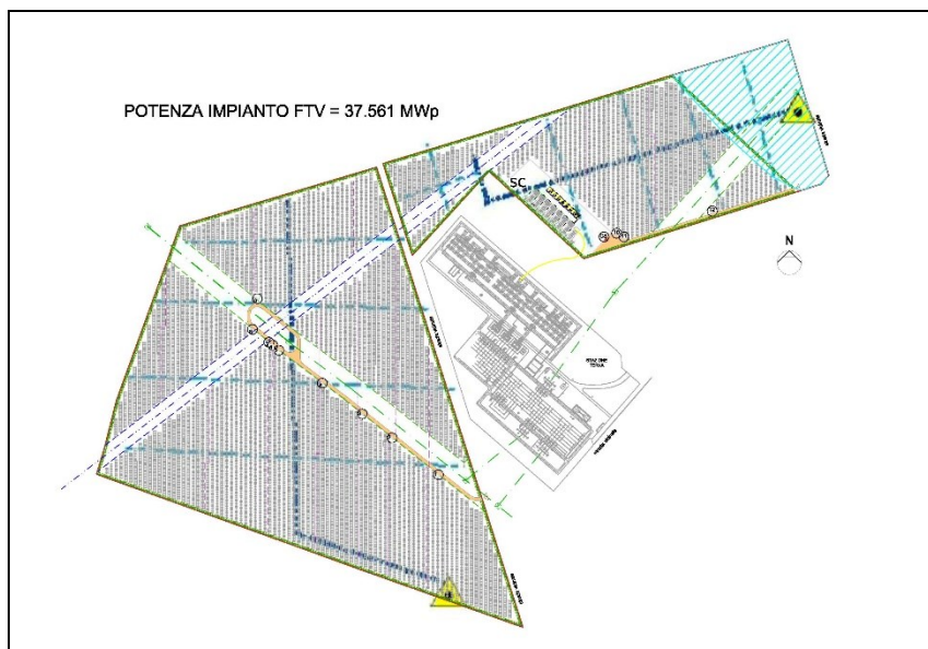
Layout impianto irriguo con sezioni fotovoltaico
