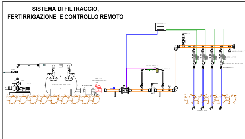
Tav. n. 4 - Sistema di filtraggio, fertirrigazione e controllo remoto
