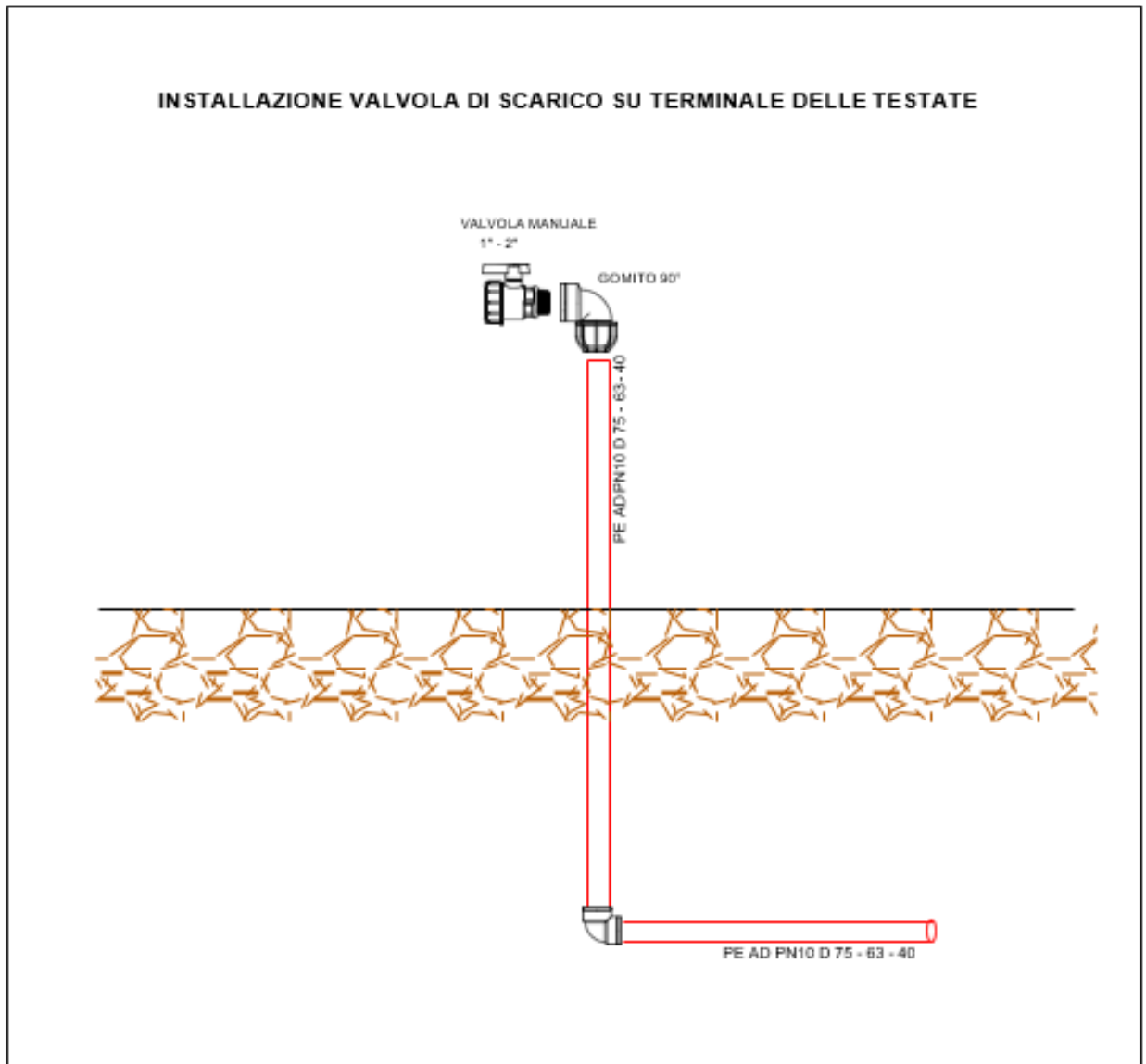
Tav. n. 6 - Installazione valvola di scarico su terminale delle testate
