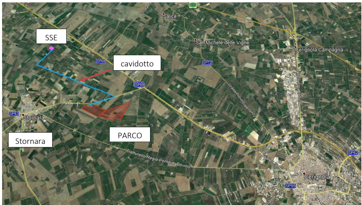
Figura 2.1: Localizzazione intervento (rosso=area parco; ciano=cavidotto; magenta SSE)
