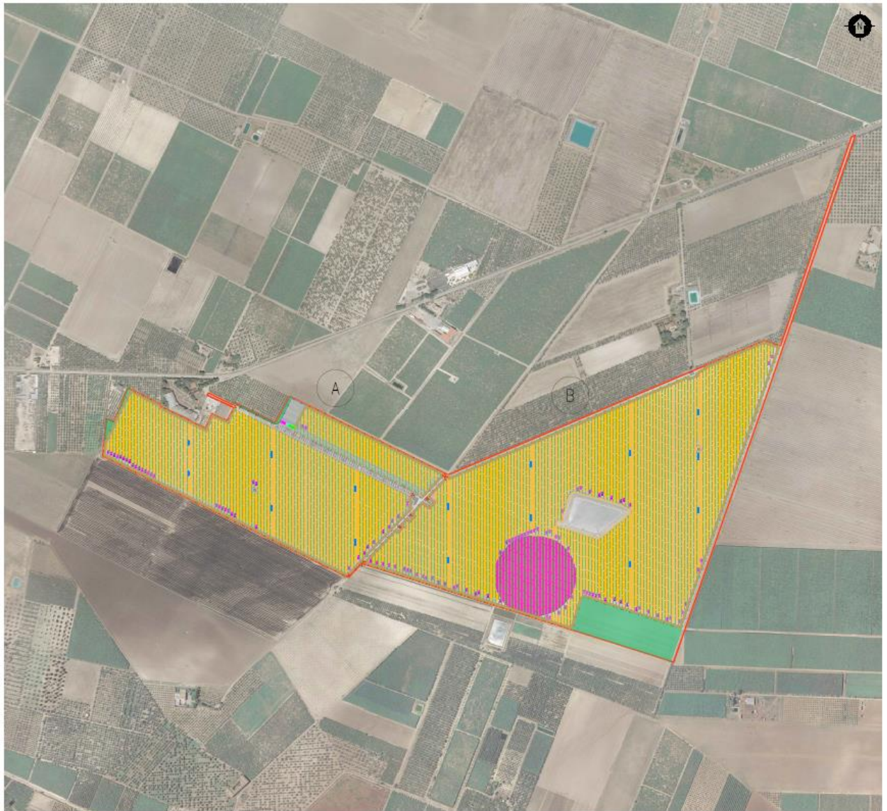
Figura 3.1: Layout di progetto
