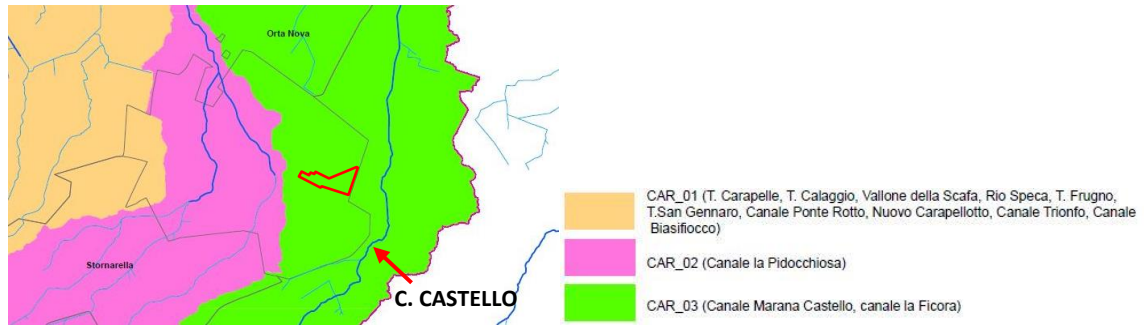
Figura 2.6: Stralcio carta dei corsi d'acqua ricadenti nel bacino del T. Carapelle con area contribuyente uguale o maggiore di 25 kmq. In rosso l'area di progetto.
