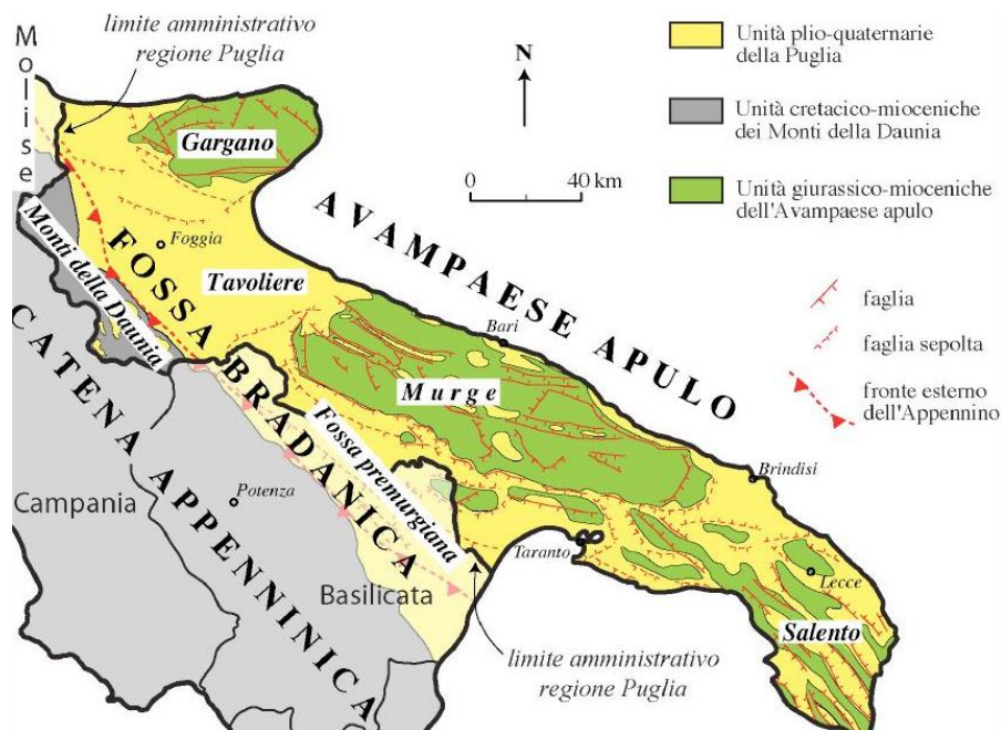
Figura 2.7: Carta geologica schematica della regione Puglia (da Pieri et alii, 1997, modificata)
