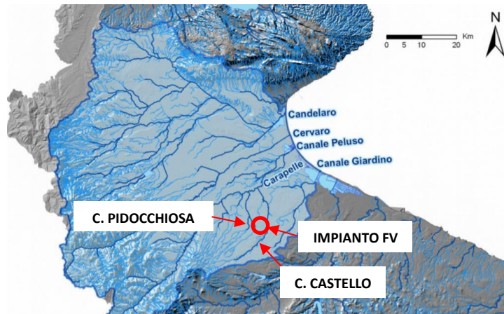
Figura 2.5: Corpi idrici superficiali (Relazione PGR - AdB Puglia, modificata) ed ubicazione area di progetto.
