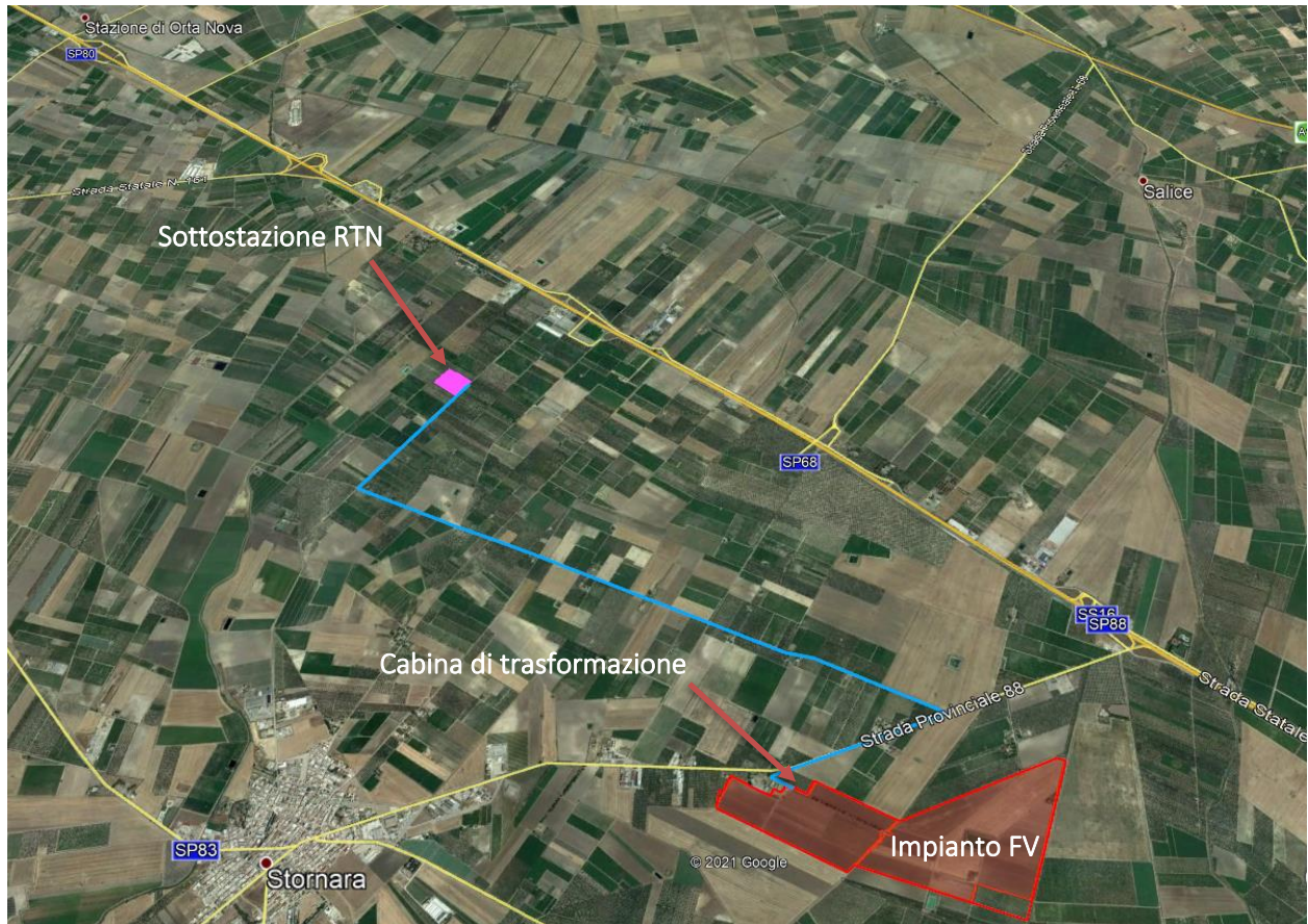
Figura 3.7. percorso di connessione dalla cabina di trasformazione alla Sottostazione AT di Stornara
