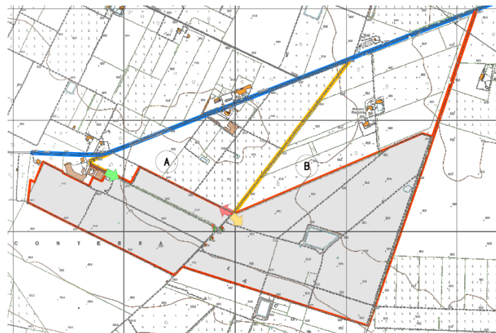
Figura 3.5: Accessi area impianto
