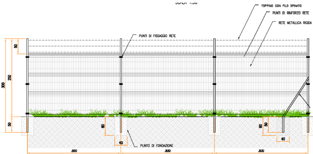
Figura 3.4: Particolare recinzione
