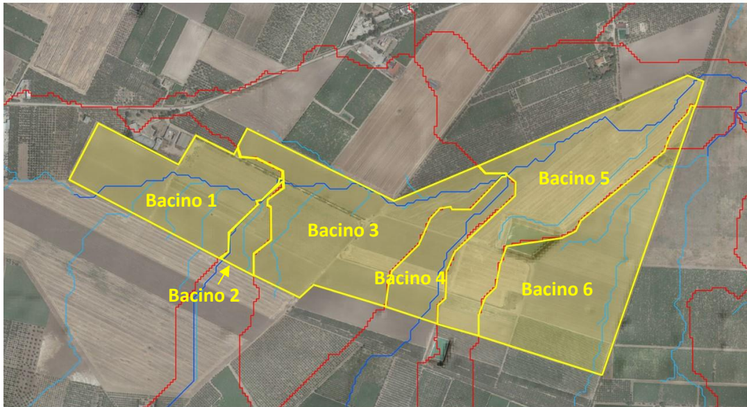
Figura 5.5: Delimitazione bacini scolanti e codifica, reticolo di drenaggio esterno ed interno alle sezioni di progetto (blu) e limiti bacini idrografici (rosso).
