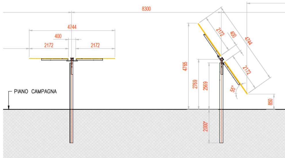
Figura 4.1: Particolare strutture di sostegno moduli.
