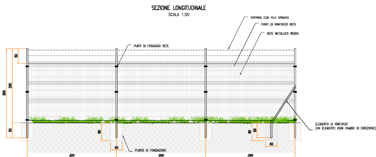
Figura 5.1: Tipico recinzione
