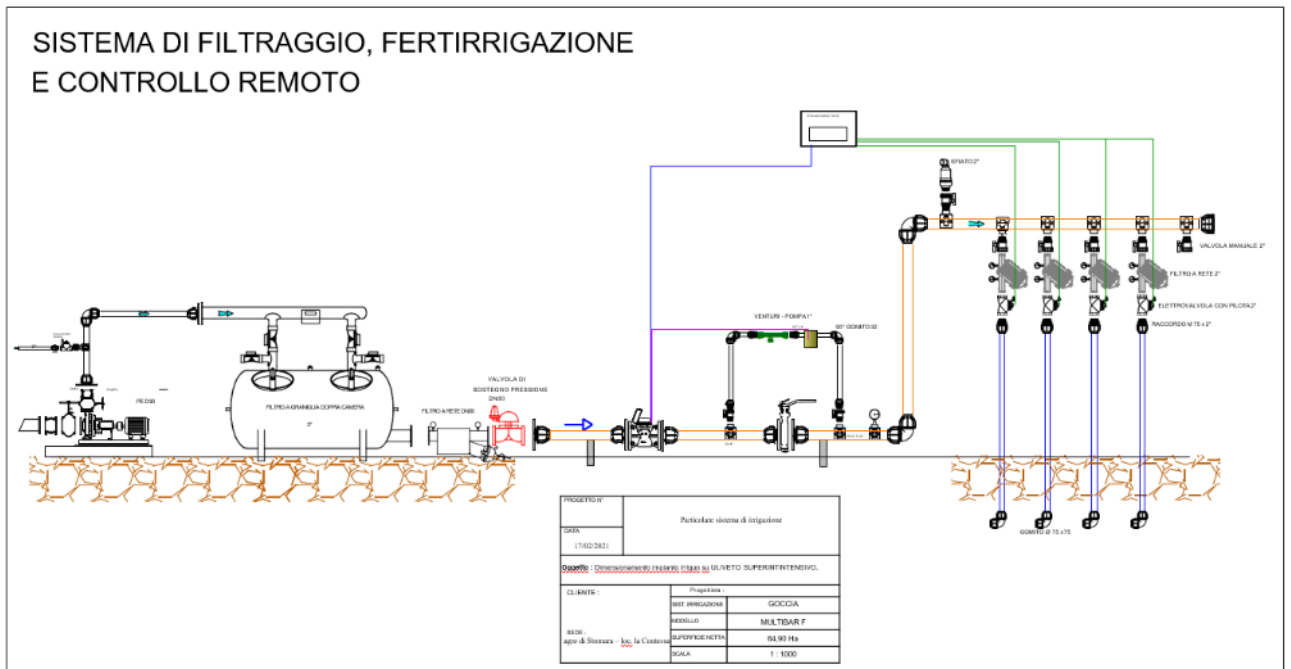
Tav. n. 4 Schema installazione ali gocciolanti
