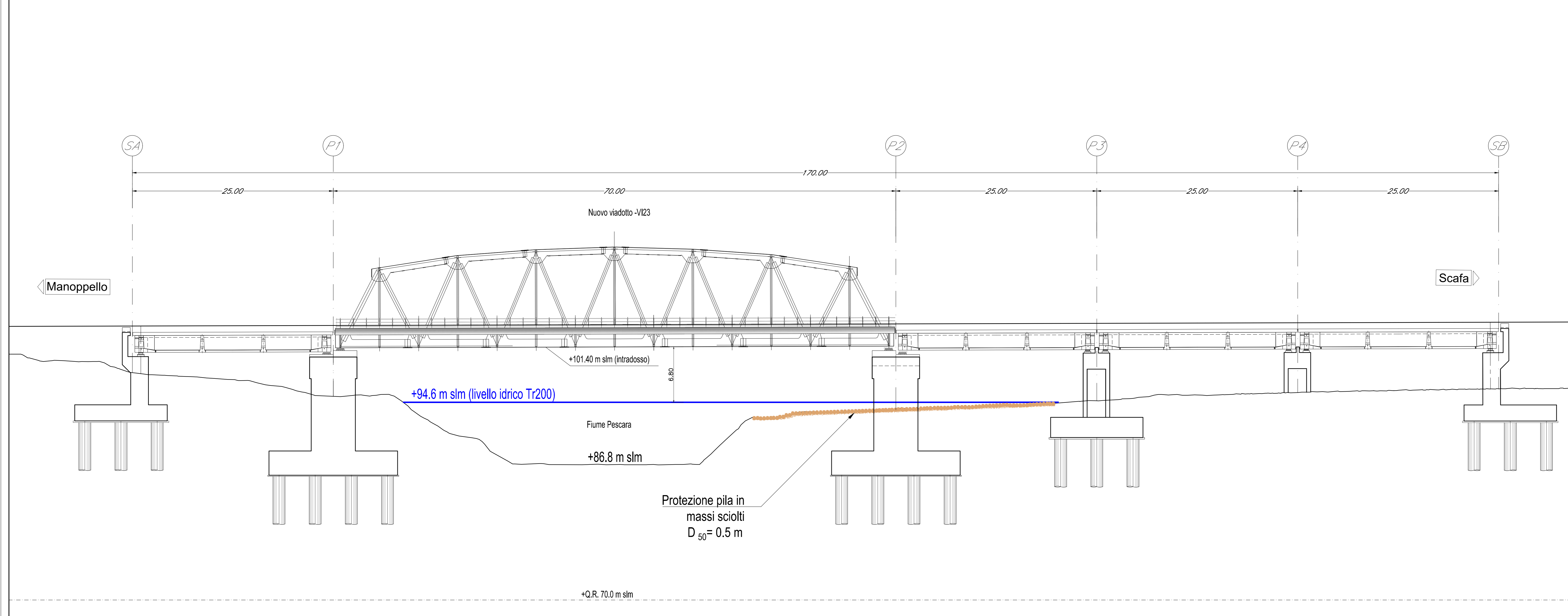
Sezione A-A sistemazione idraulica (scala 1:200)
