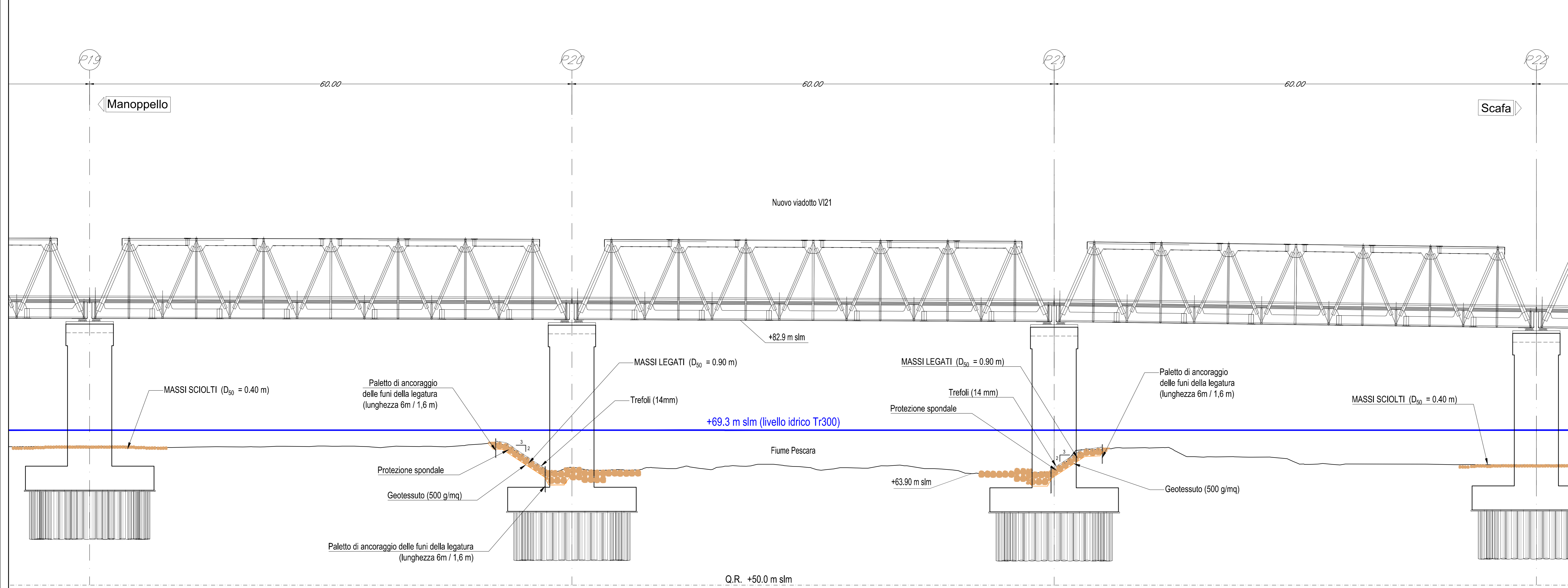
Sezione A-A sistemazione idraulica (scala 1:200)
