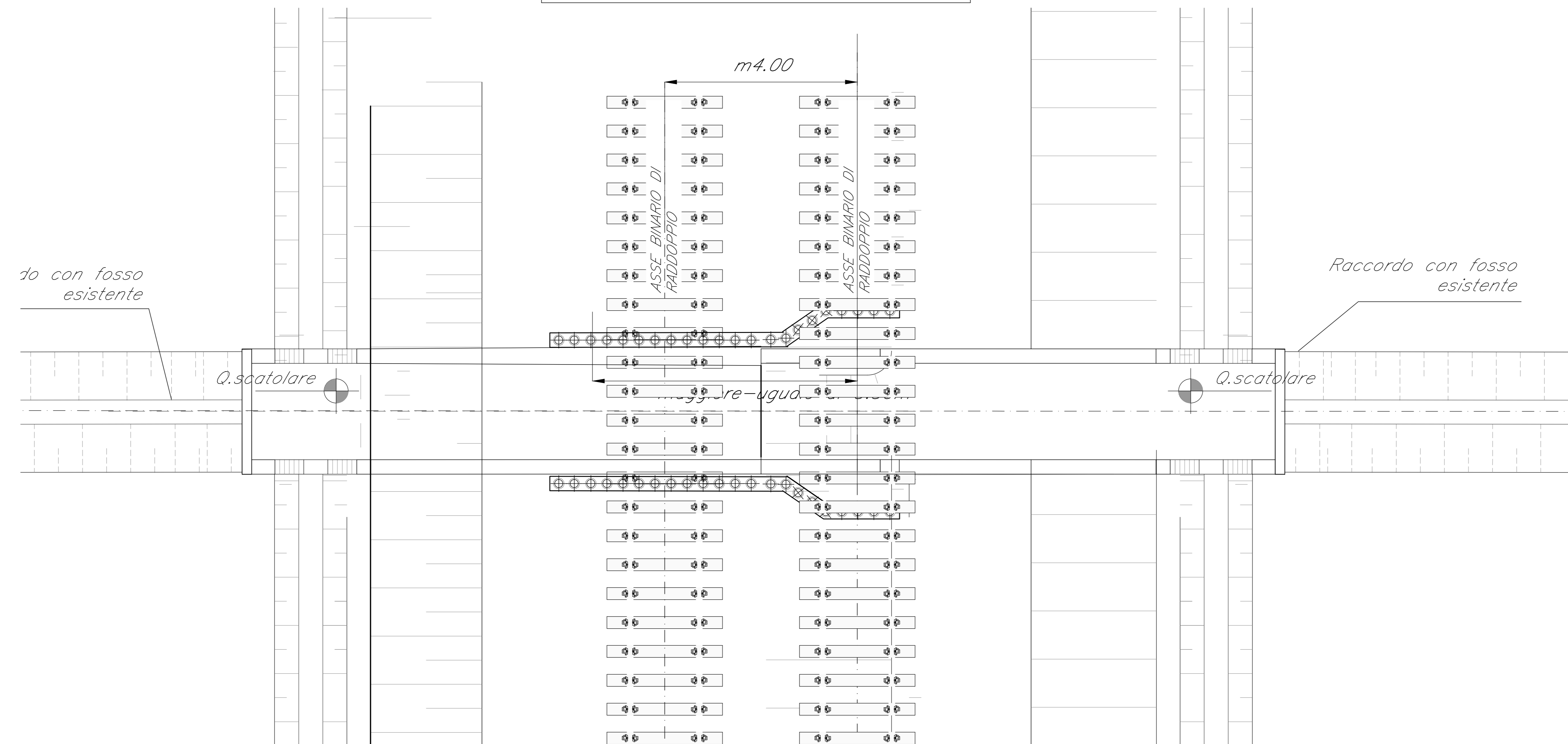
PLANIMETRIA Fase 3 - Scala 1:50
