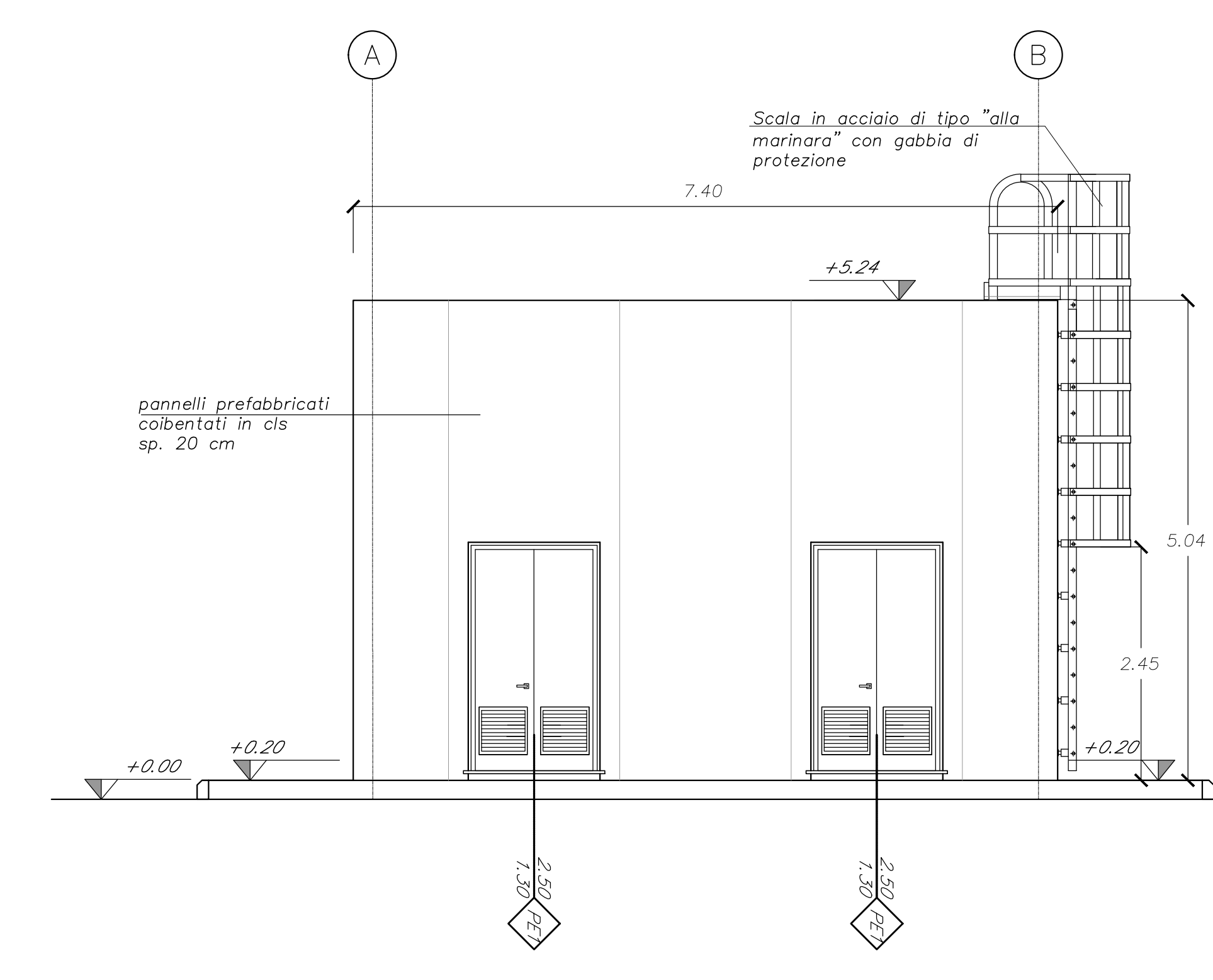
Prospetto 4 Scala 1:50
