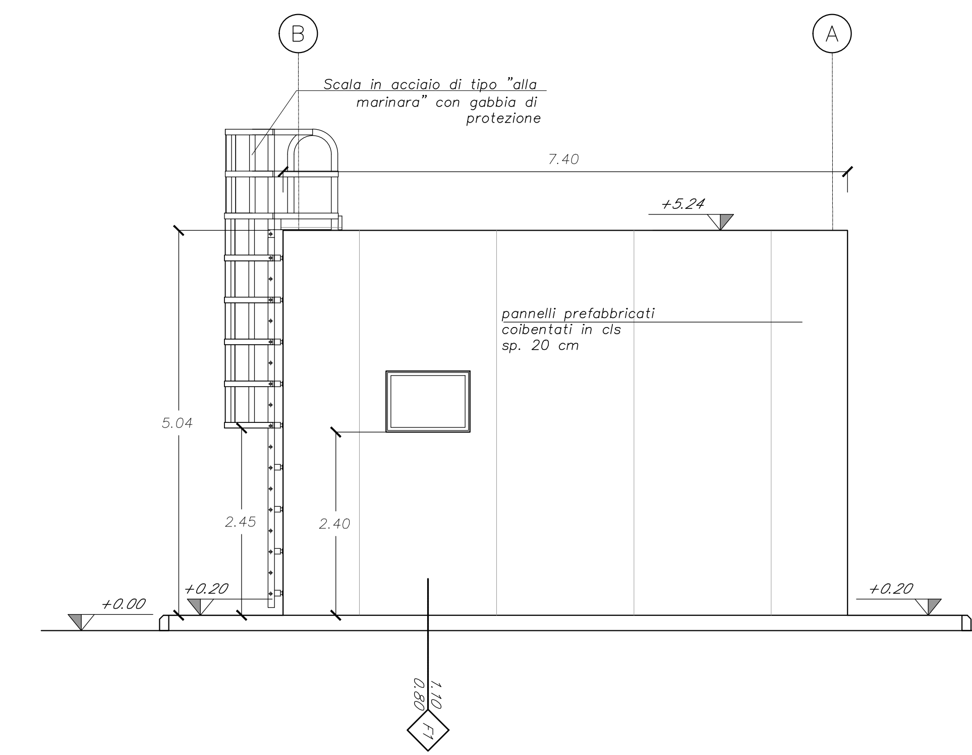
Prospetto 4 Scala 1:50
